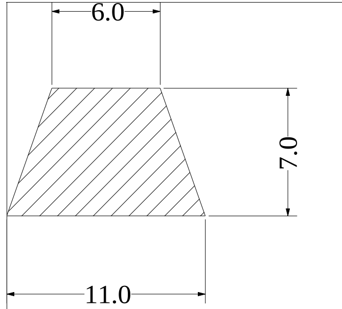
Die No: 460 Category: Trapeze
