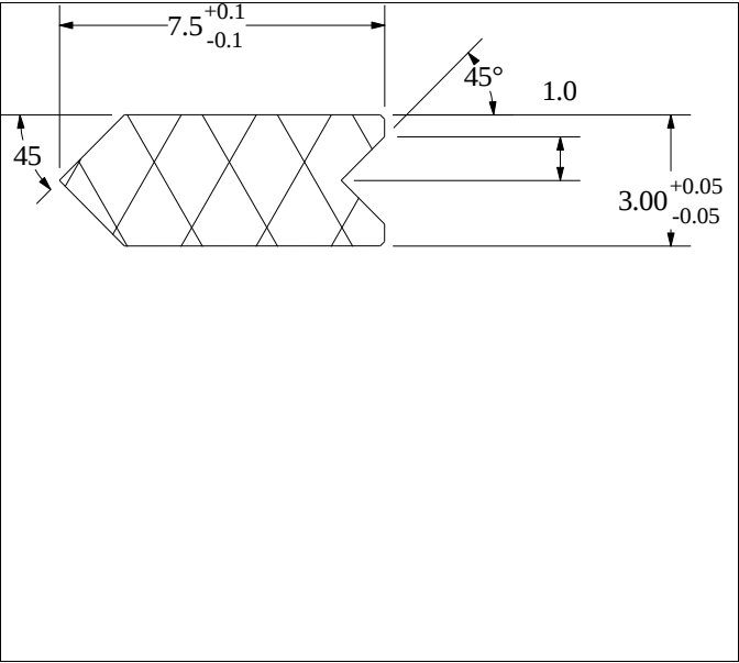
Die No: 2410 Category: Trapeze
