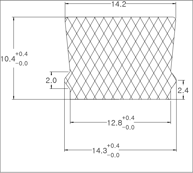
Die No: 7810 Category: Trapeze
