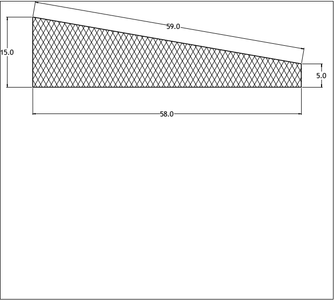
Die No: 7533 Category: Trapeze
