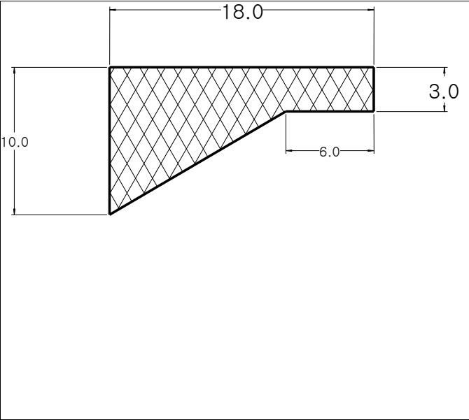
Die No: 8772 Category: Trapeze
