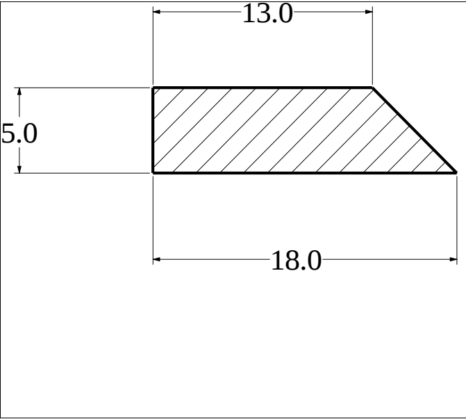
Die No: 2232 Category: Trapeze
