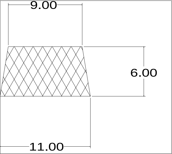
Die No: 4665 Category: Trapeze
