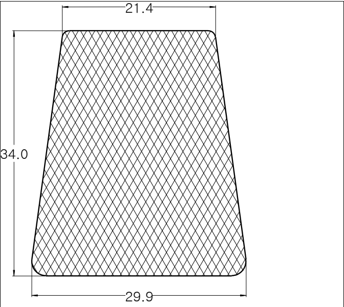
Die No: 8391 Category: Trapeze
