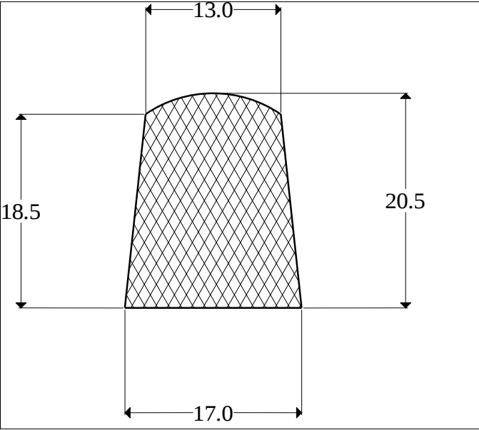
Die No: 5314 Category: Trapeze
