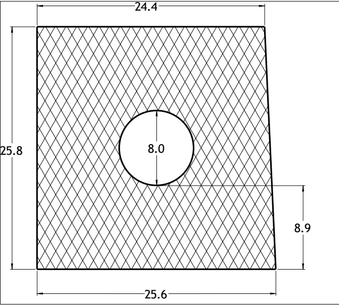
Die No: 6376 Category: Trapeze
