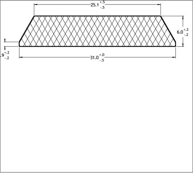
Die No: 6189 Category: Trapeze
