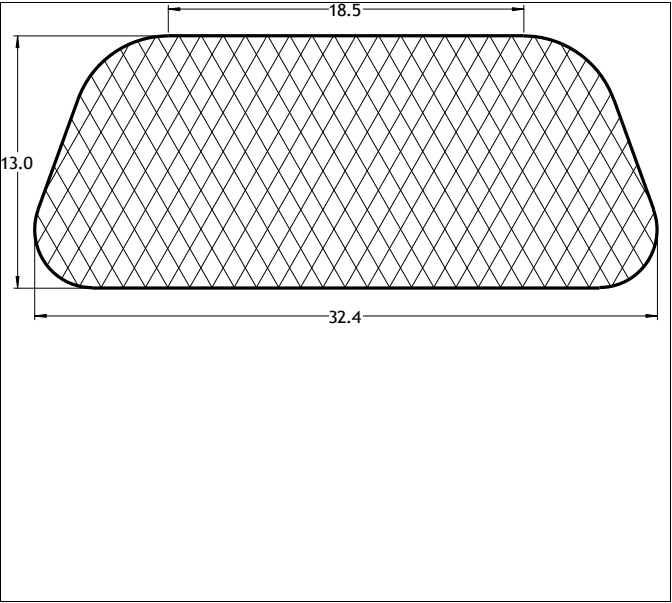
Die No: 6913 Category: Trapeze
