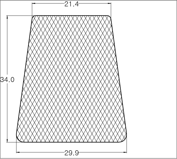
Die No: 9821 Category: Trapeze
