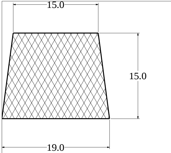
Die No: 2855 Category: Trapeze
