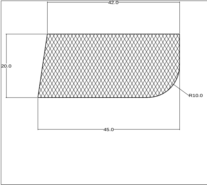
Die No: 4861 Category: Trapeze
