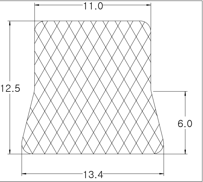
Die No: 8043 Category: Trapeze
