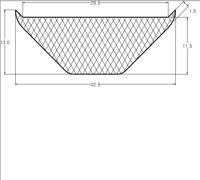
Die No: 8397 Category: Trapeze
