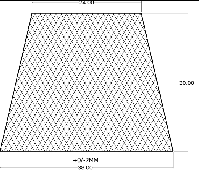
Die No: 5622 Category: Trapeze
