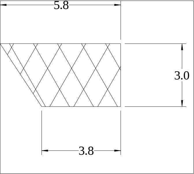
Die No: 5236 Category: Trapeze
