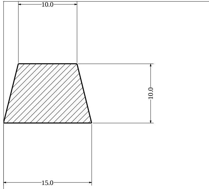
Die No: 341 Category: Trapeze
