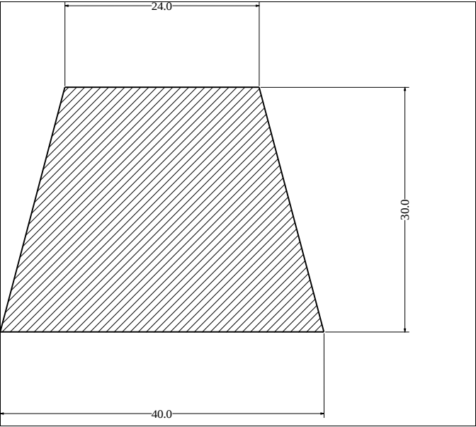
Die No: 1039 Category: Trapeze
