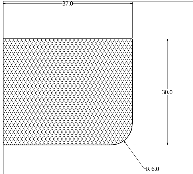
Die No: 3404 Category: Trapeze
