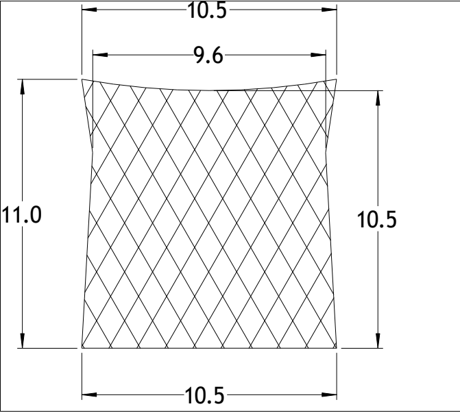
Die No: 6241 Category: Trapeze
