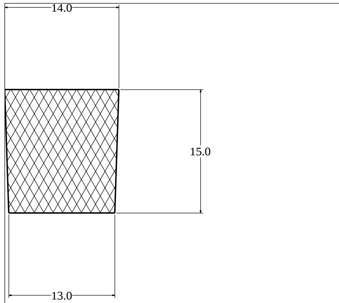
Die No: 2722 Category: Trapeze
