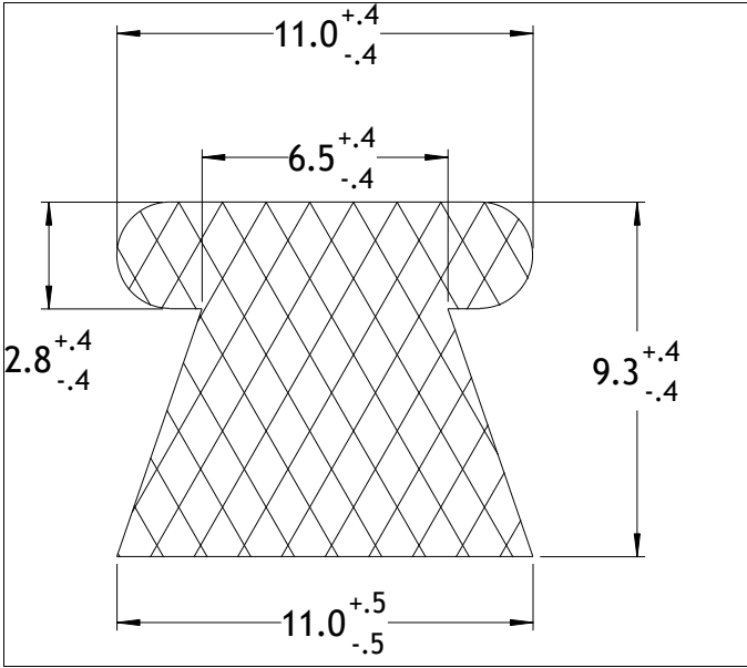
Die No: 6488 Category: Trapeze
