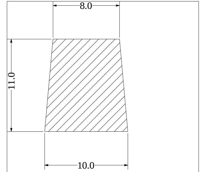
Die No: 342 Category: Trapeze
