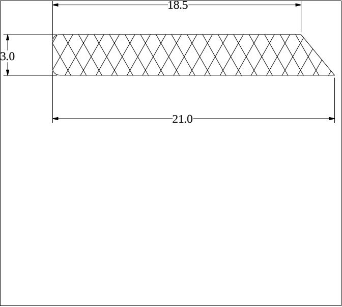
Die No: 2200 Category: Trapeze
