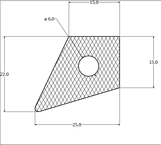
Die No: 2425 Category: Trapeze
