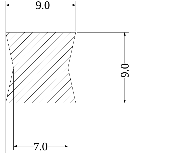
Die No: 881 Category: Trapeze
