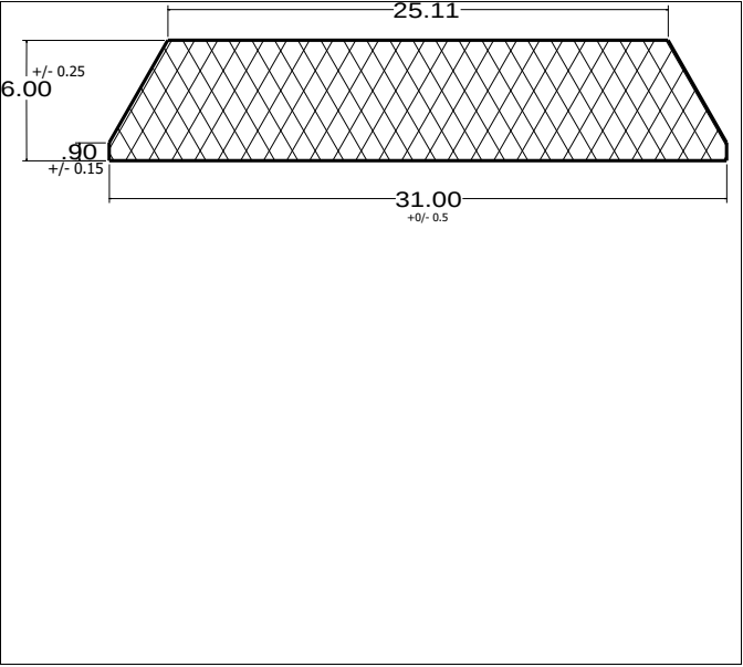
Die No: 5635 Category: Trapeze
