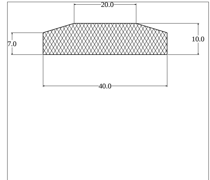
Die No: 2794 Category: Trapeze
