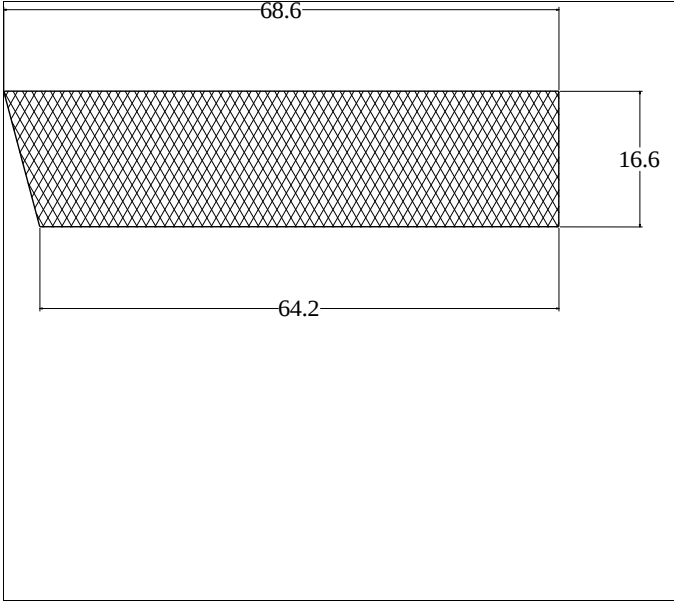
Die No: 2521 Category: Trapeze
