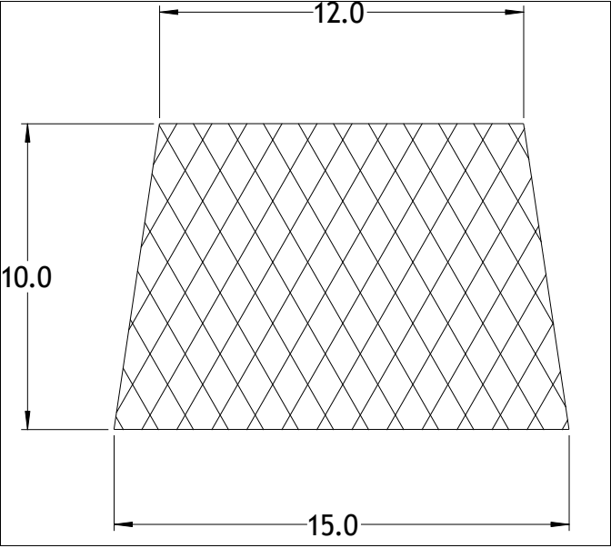
Die No: 7294 Category: Trapeze
