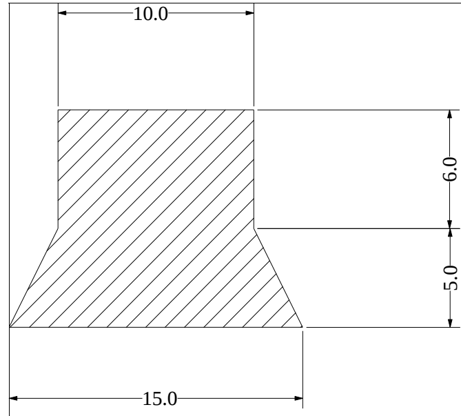
Die No: 874 Category: Trapeze
