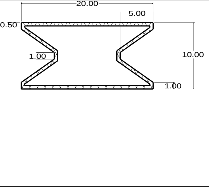
Die No: 4330 Category: Trapeze
