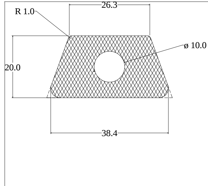
Die No: 2764 Category: Trapeze
