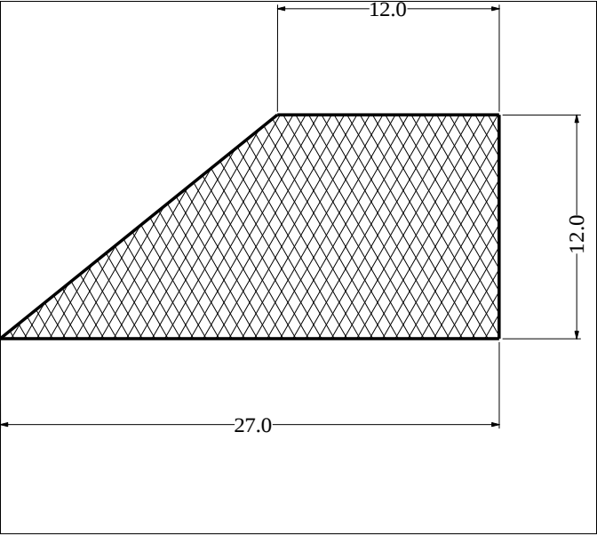
Die No: 1763 Category: Trapeze
