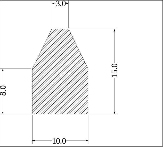
Die No: 1628 Category: Trapeze
