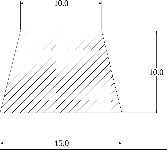
Die No: 1823 Category: Trapeze
