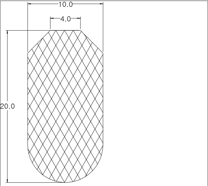
Die No: 8615 Category: Trapeze
