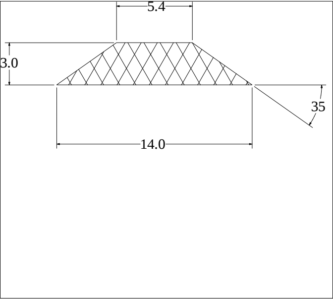
Die No: 3839 Category: Trapeze
