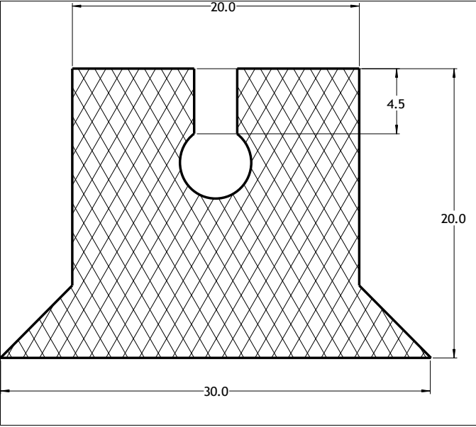
Die No: 6058 Category: Trapeze
