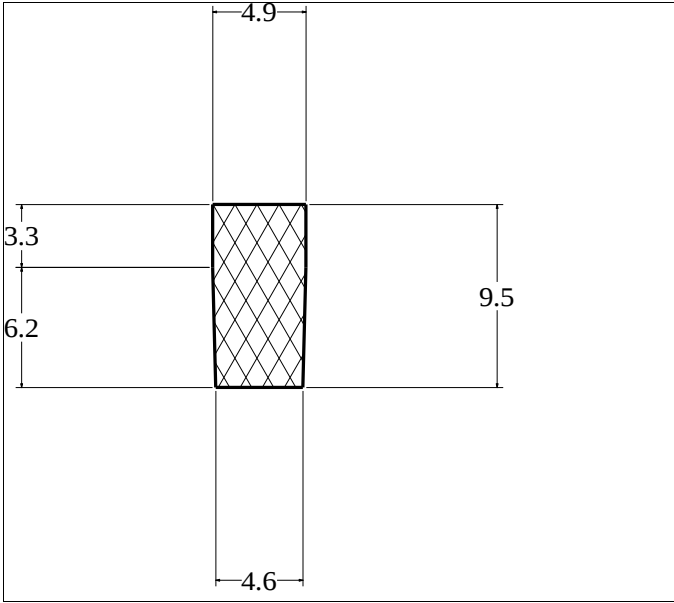
Die No: 3928 Category: Trapeze
