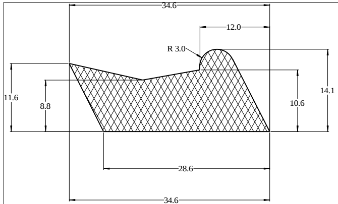
Die No: 5329 Category: Trapeze
