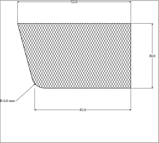
Die No: 3418 Category: Trapeze
