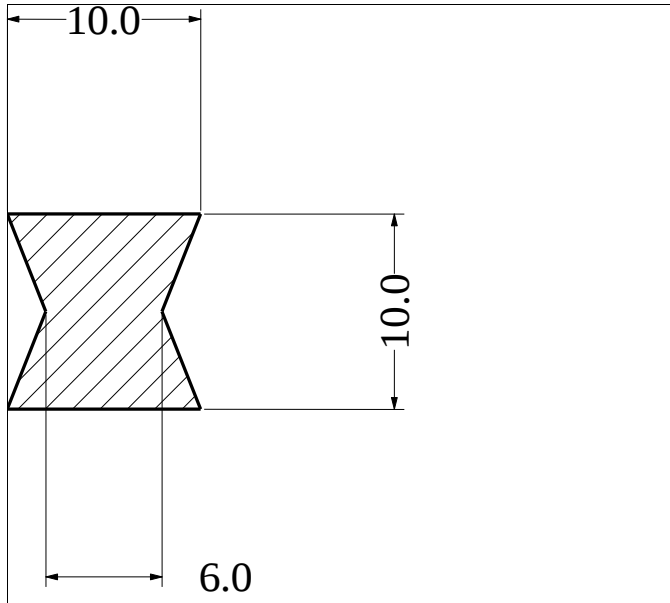
Die No: 314 Category: Trapeze
