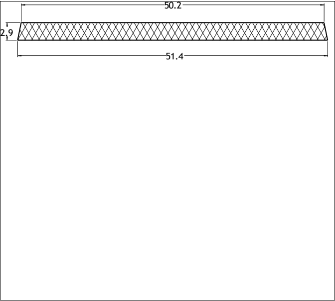
Die No: 6359 Category: Trapeze
