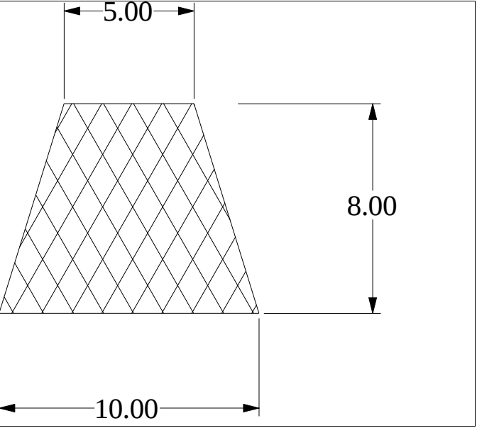
Die No: 3509 Category: Trapeze
