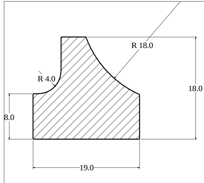
Die No: 1332 Category: Trapeze
