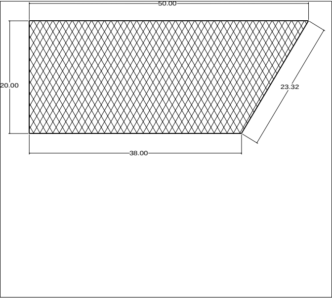
Die No: 5928 Category: Trapeze
