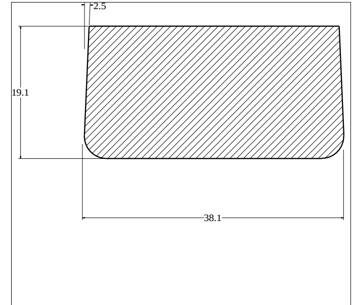
Die No: 1336 Category: Trapeze
