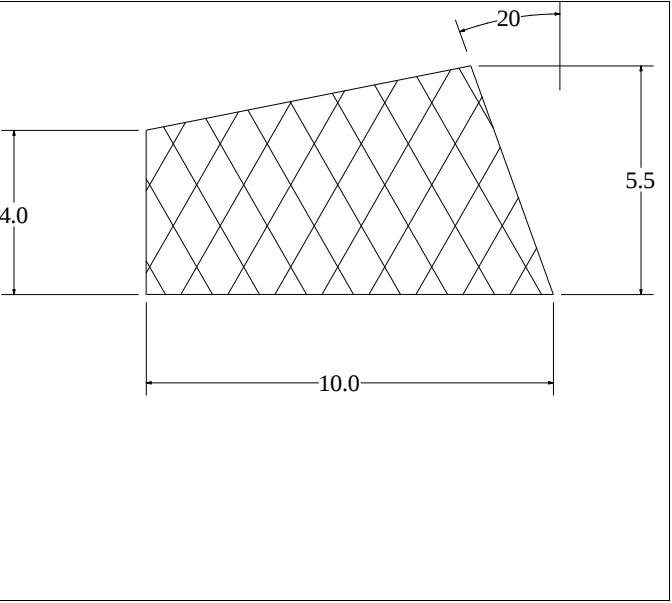
Die No: 3161 Category: Trapeze
