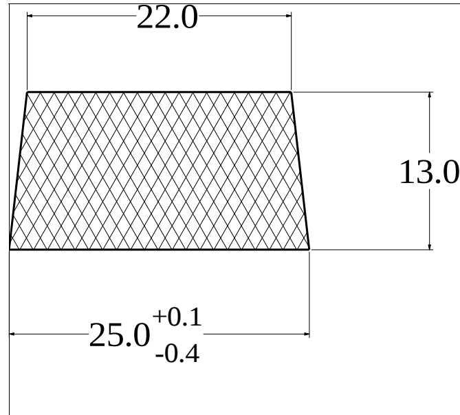
Die No: 2874 Category: Trapeze
