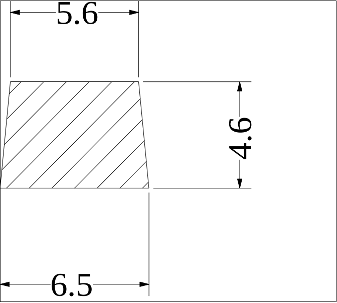
Die No: 1100 Category: Trapeze
