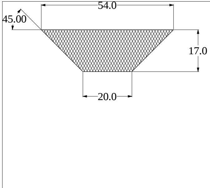
Die No: 3400 Category: Trapeze
