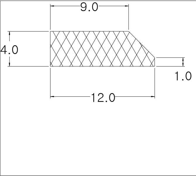
Die No: 9079 Category: Trapeze
