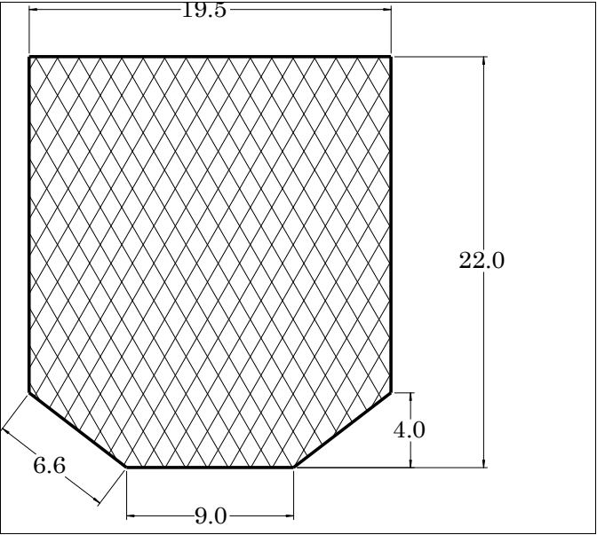
Die No: 7906 Category: Trapeze
