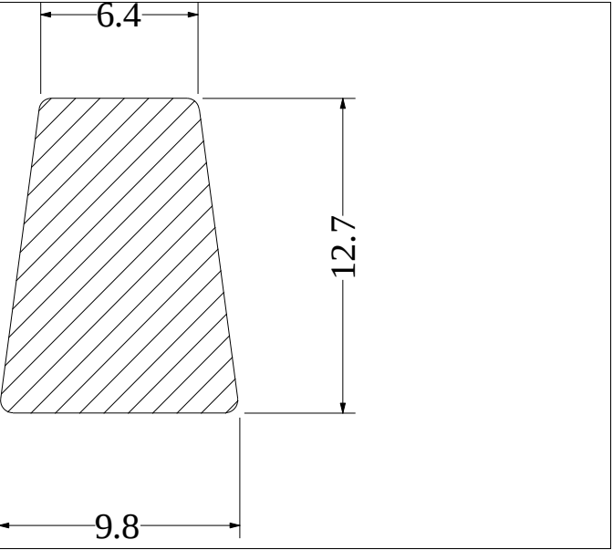
Die No: 1145 Category: Trapeze
