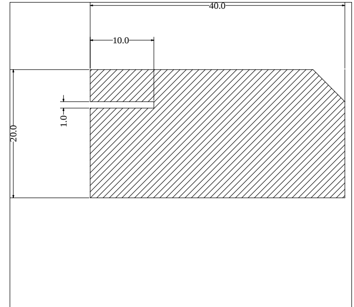
Die No: 476 Category: Trapeze
