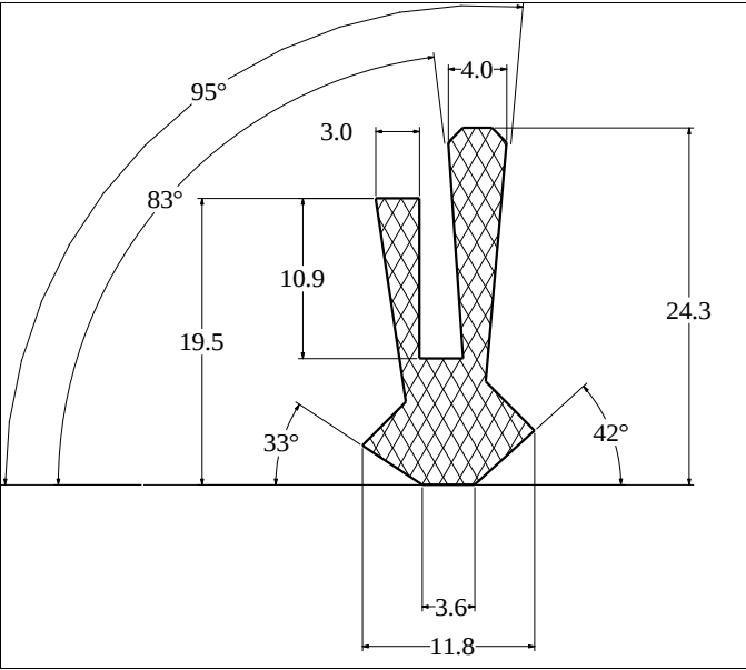
Die No: 3175 Category: Tank-Seal
