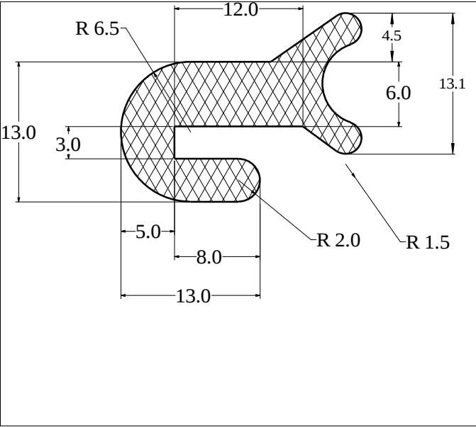
Die No: 5403 Category: Tank-Seal
