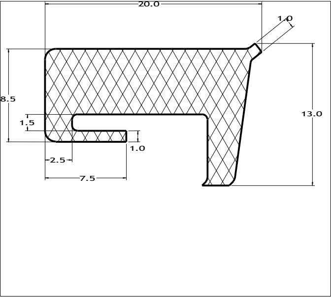
Die No: 8293 Category: Tank-Seal
