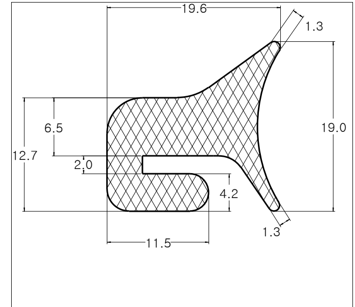
Die No: 9484 Category: Tank-Seal
