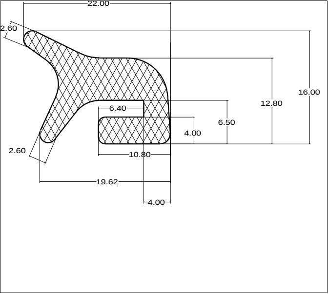
Die No: 5734 Category: Tank-Seal
