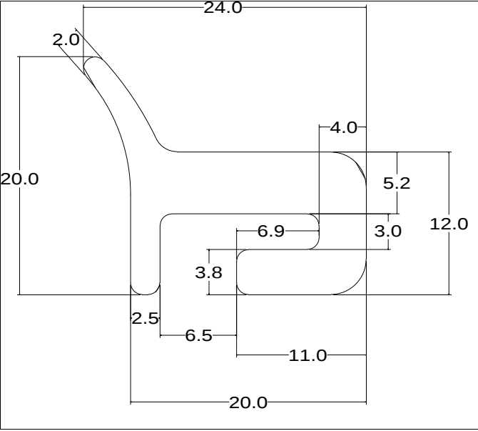
Die No: 5243 Category: Tank-Seal
