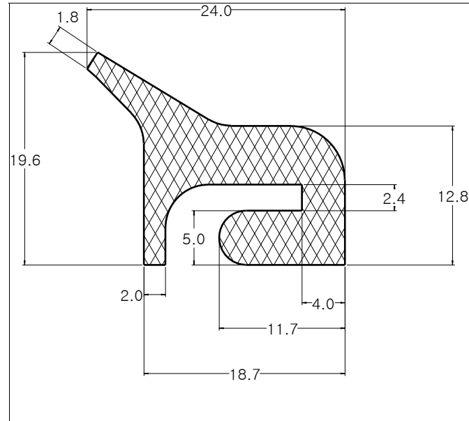
Die No: 9116 Category: Tank-Seal
