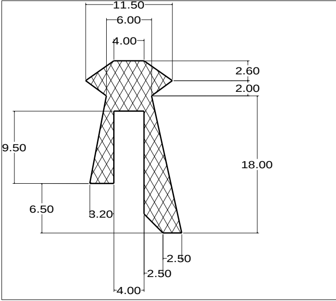
Die No: 4186 Category: Tank-Seal
