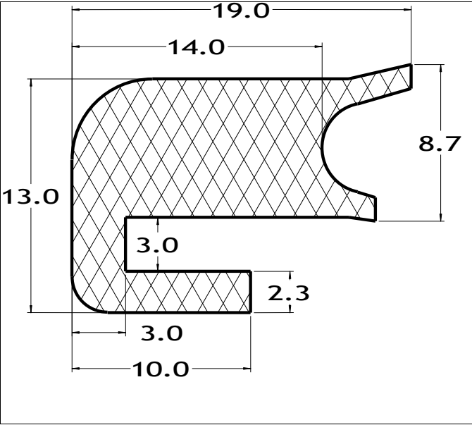
Die No: 8531 Category: Tank-Seal
