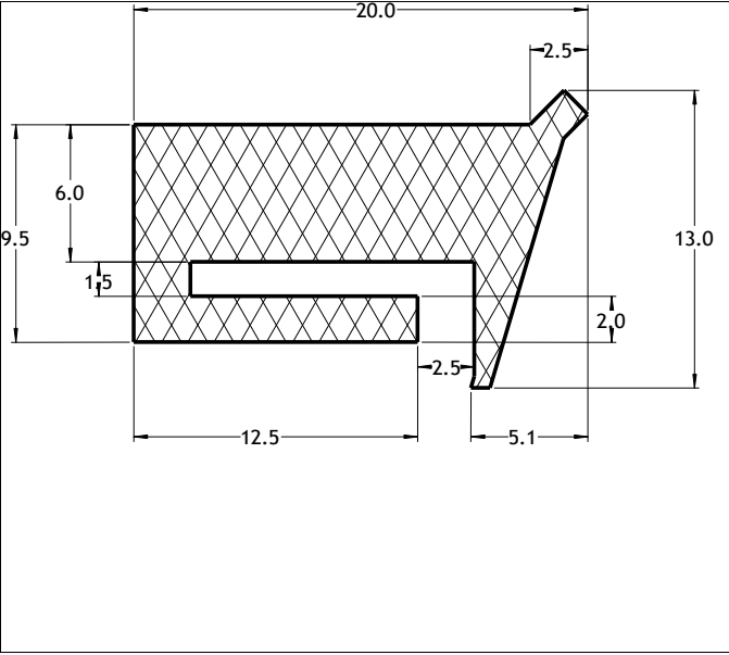
Die No: 7312 Category: Tank-Seal
