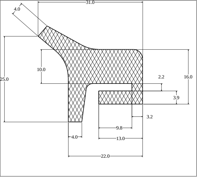
Die No: 3035 Category: Tank-Seal
