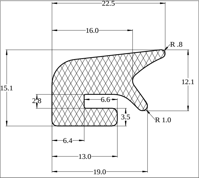
Die No: 5210 Category: Tank-Seal
