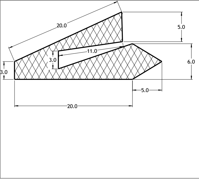
Die No: 7295 Category: Tank-Seal
