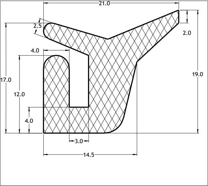
Die No: 7261 Category: Tank-Seal
