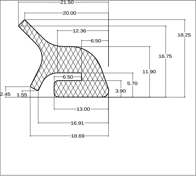
Die No: 5728 Category: Tank-Seal
