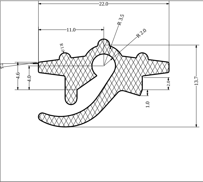
Die No: 2205 Category: Tank-Seal
