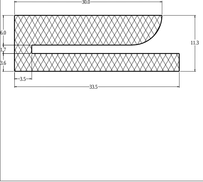
Die No: 10095 Category: Tank-Seal
