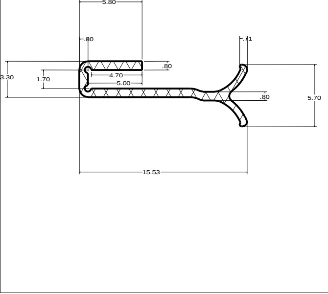
Die No: 4511 Category: Tank-Seal
