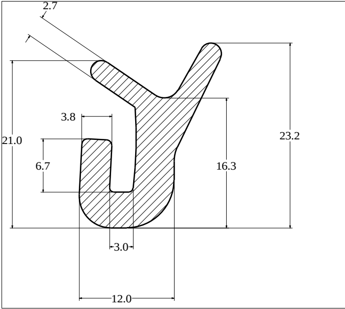
Die No: 2539 Category: Tank-Seal
