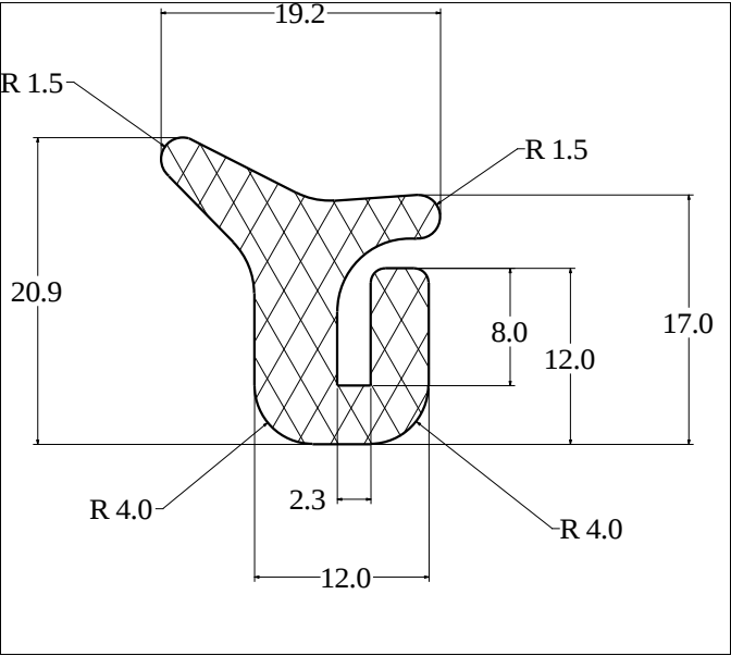
Die No: 2927 Category: Tank-Seal
