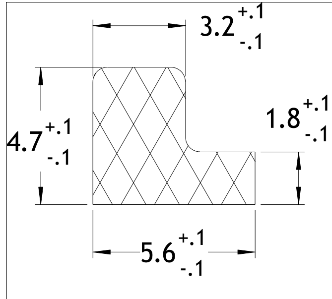
Die No: 7494 Category: L-Section
