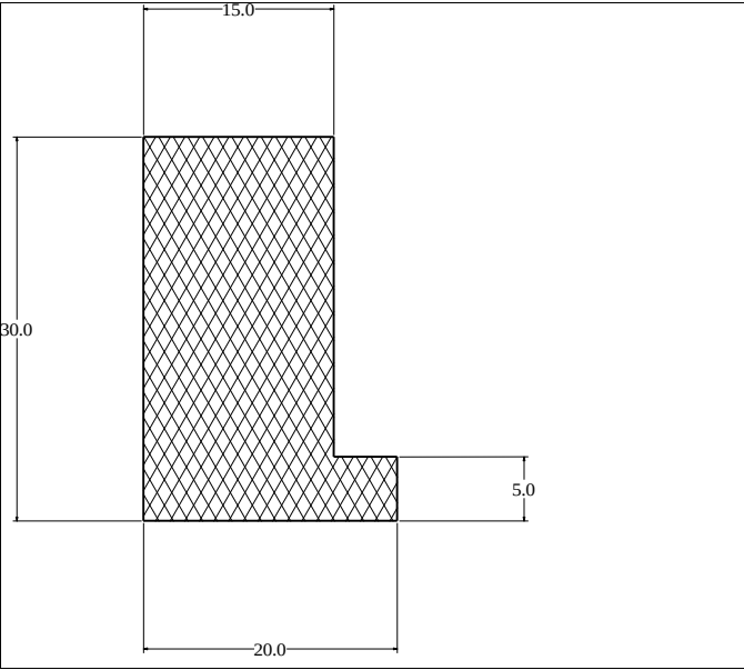
Die No: 3232 Category: L-Section
