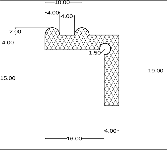
Die No: 4340 Category: L-Section
