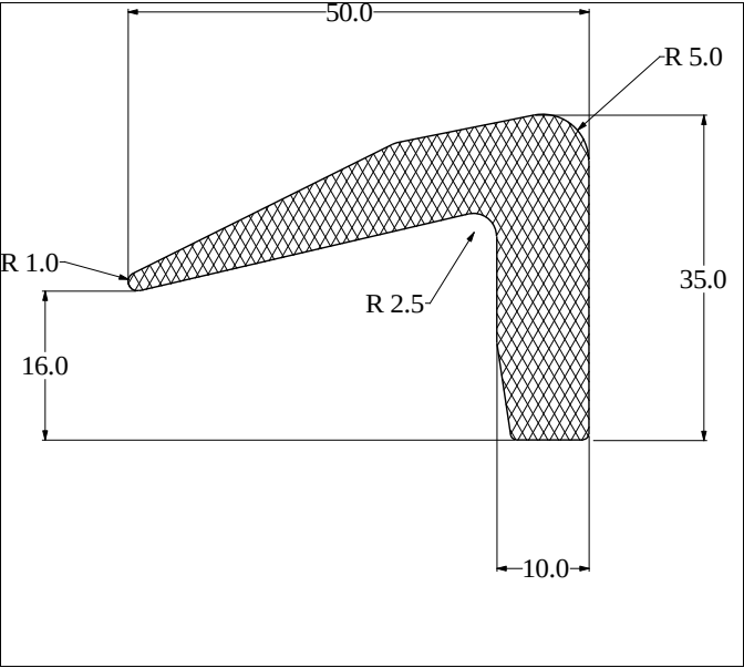
Die No: 2795 Category: L-Section
