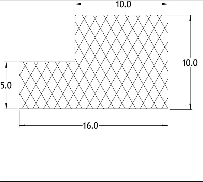
Die No: 6640 Category: L-Section
