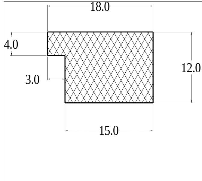
Die No: 9154 Category: L-Section
