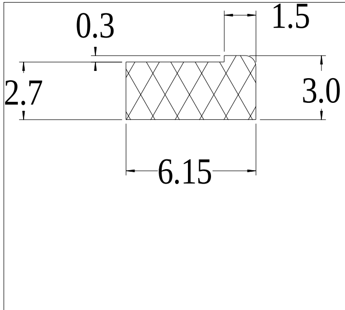
Die No: 9057 Category: L-Section
