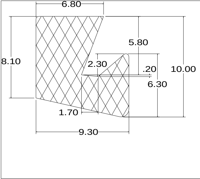
Die No: 6090 Category: L-Section
