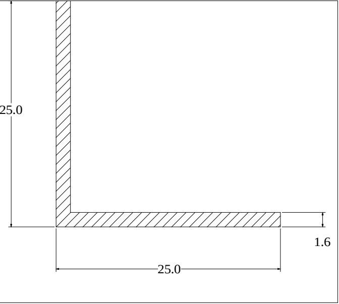
Die No: 752 Category: L-Section
