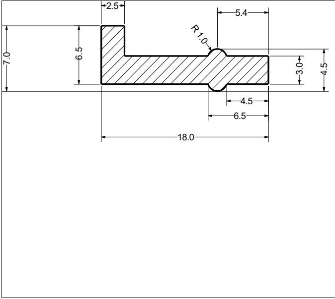
Die No: 1535 Category: L-Section
