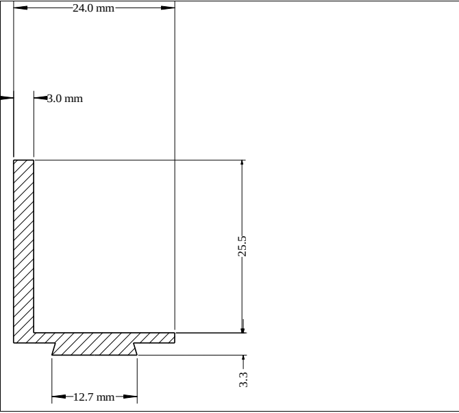
Die No: 1149 Category: L-Section
