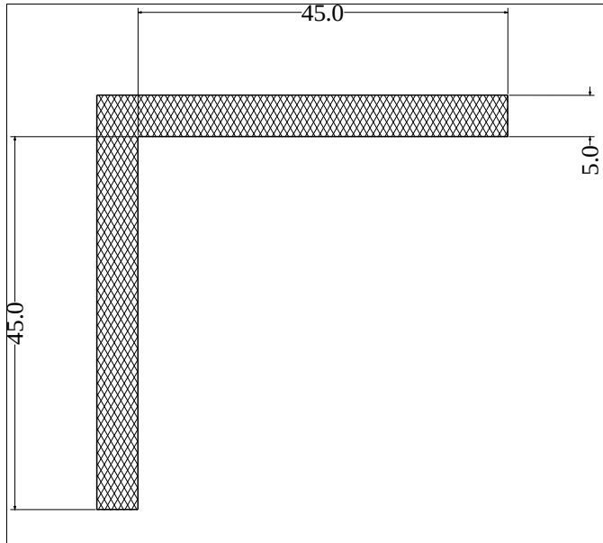
Die No: 1716 Category: L-Section
