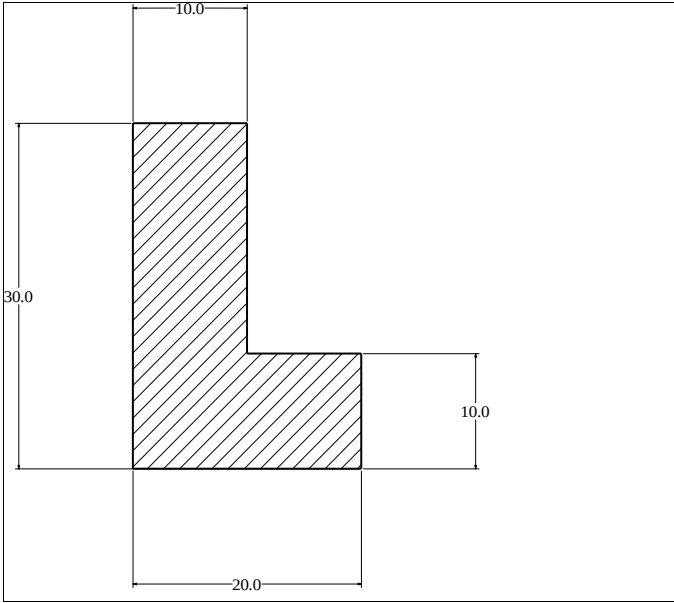
Die No: 1155 Category: L-Section
