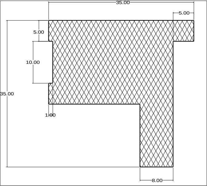
Die No: 4147 Category: L-Section
