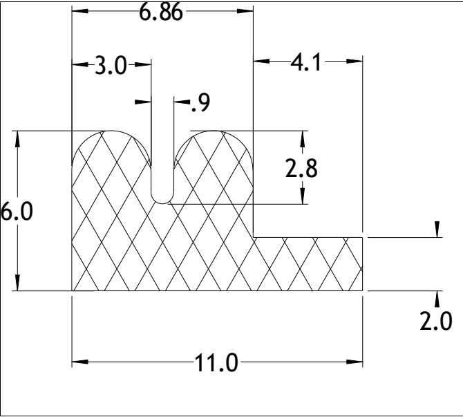
Die No: 7213 Category: L-Section
