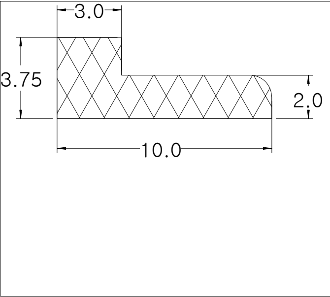
Die No: 8715 Category: L-Section
