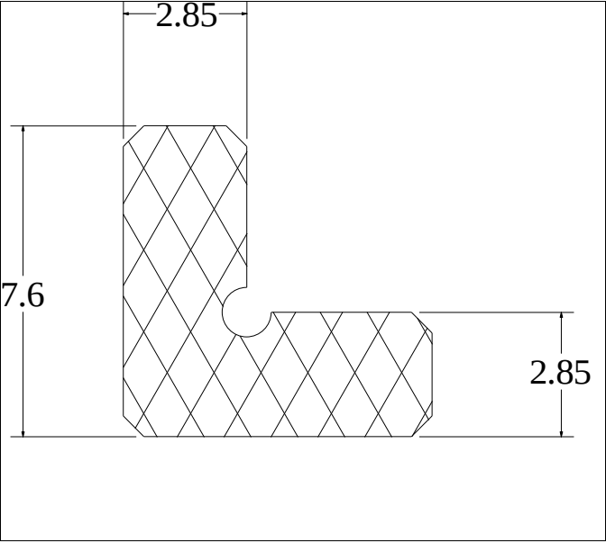
Die No: 3222 Category: L-Section
