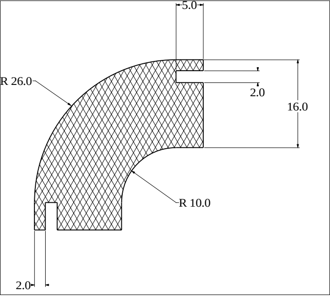
Die No: 3457 Category: L-Section
