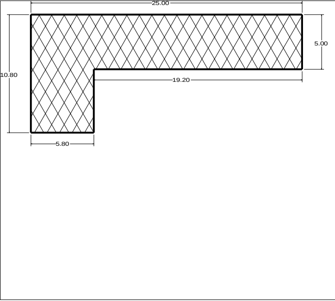
Die No: 5722 Category: L-Section
