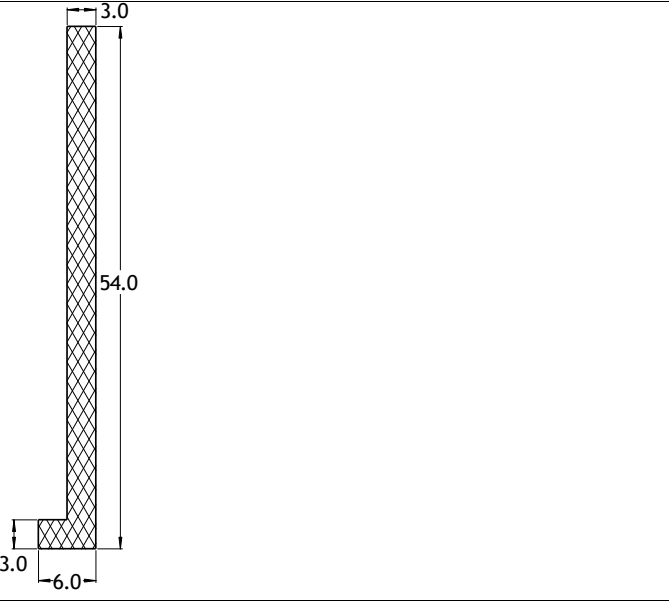
Die No: 6305 Category: L-Section
