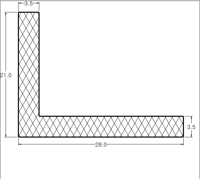
Die No: 8402 Category: L-Section
