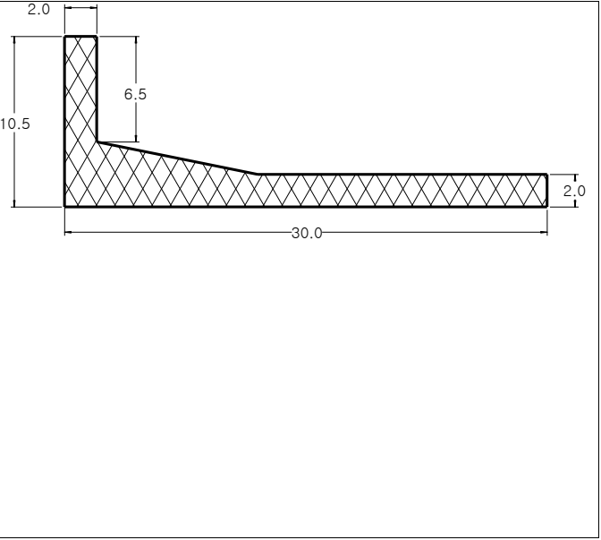
Die No: 8117 Category: L-Section
