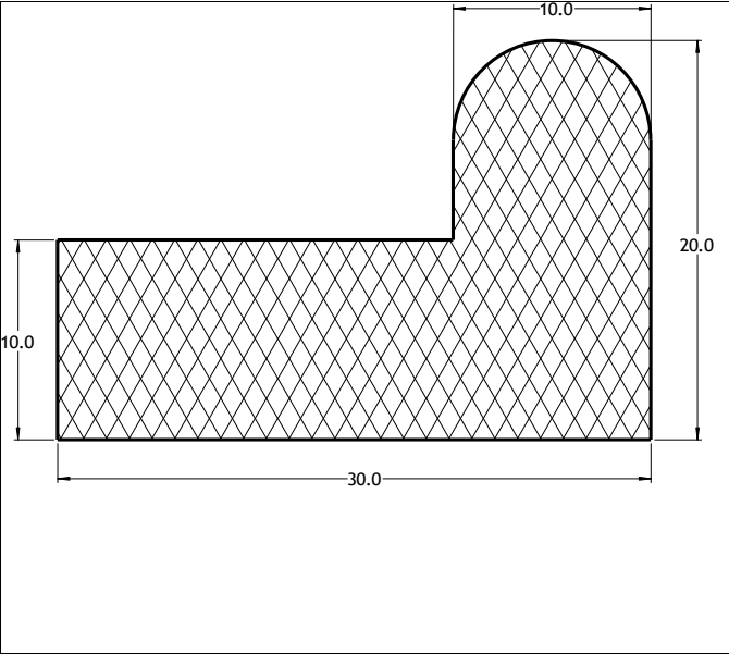
Die No: 6503 Category: L-Section
