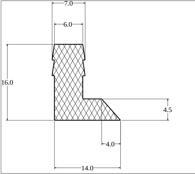
Die No: 3257 Category: L-Section
