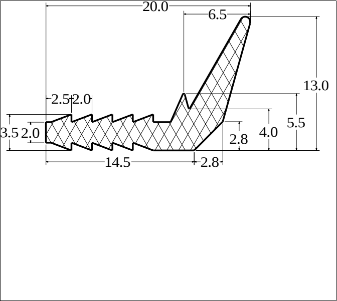
Die No: 3891 Category: L-Section
