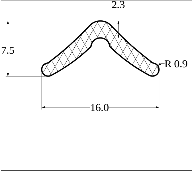
Die No: 2818 Category: L-Section
