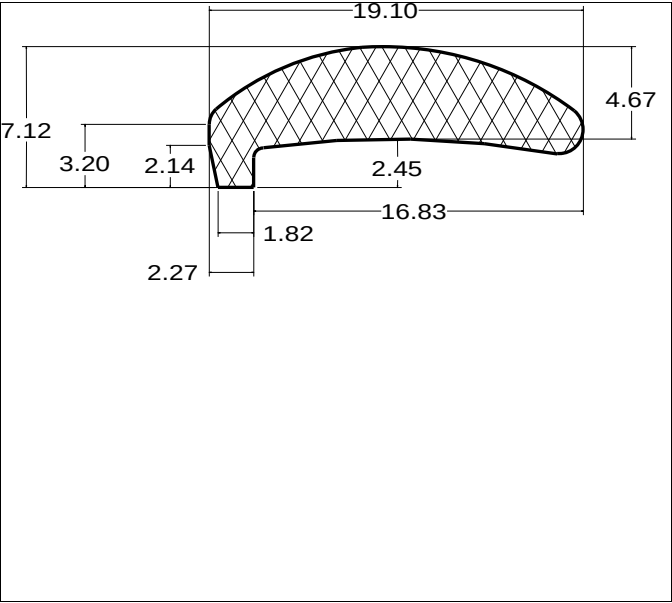
Die No: 5990 Category: L-Section
