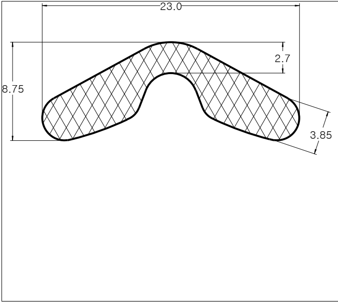
Die No: 8733 Category: L-Section
