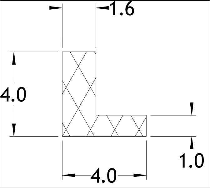
Die No: 7176 Category: L-Section
