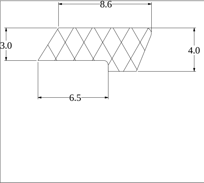
Die No: 2418 Category: L-Section
