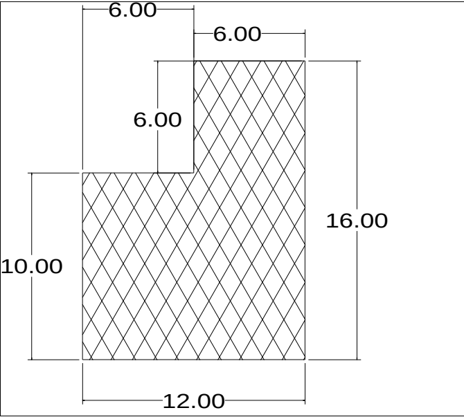
Die No: 6071 Category: L-Section
