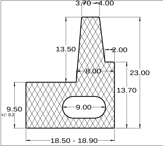
Die No: 5791 Category: L-Section
