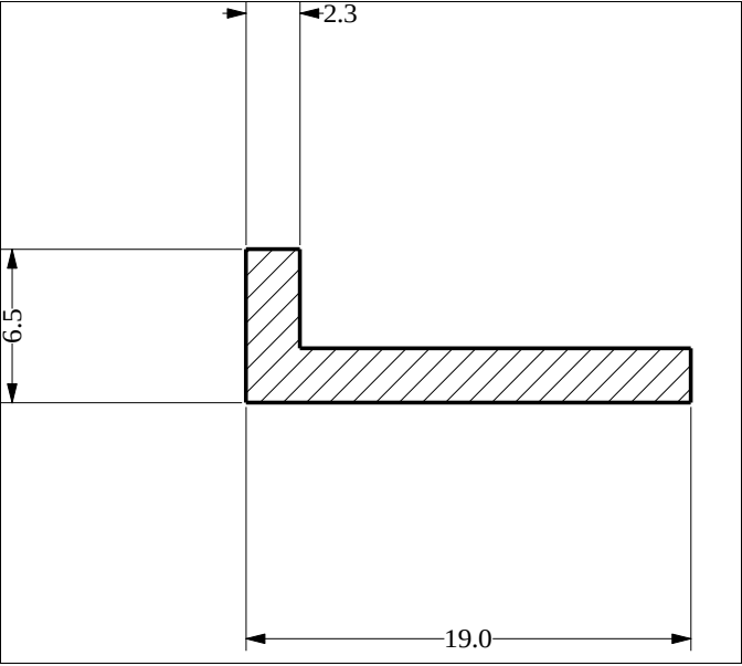
Die No: 1410 Category: L-Section
