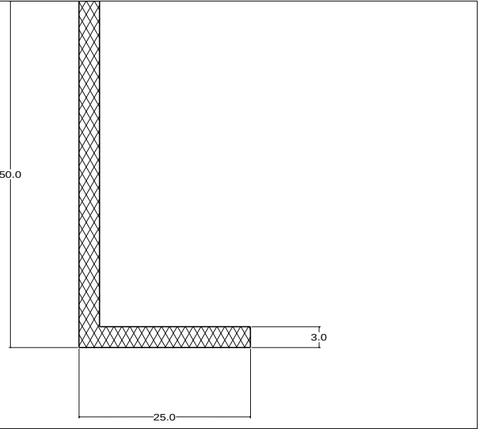
Die No: 4615 Category: L-Section
