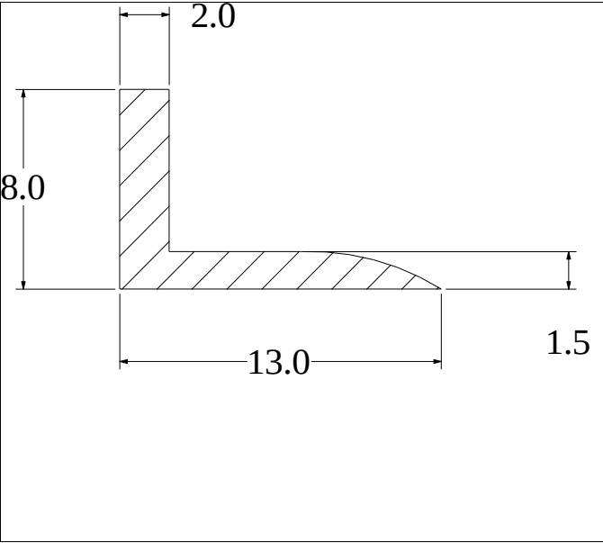
Die No: 1411 Category: L-Section
