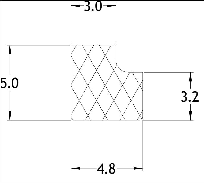
Die No: 7066 Category: L-Section
