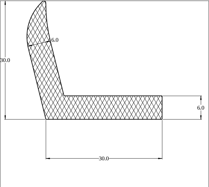
Die No: 5360 Category: L-Section
