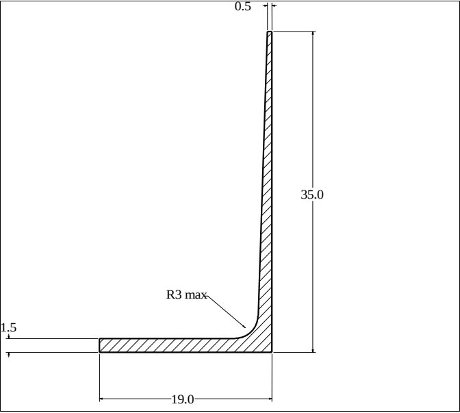
Die No: 719 Category: L-Section
