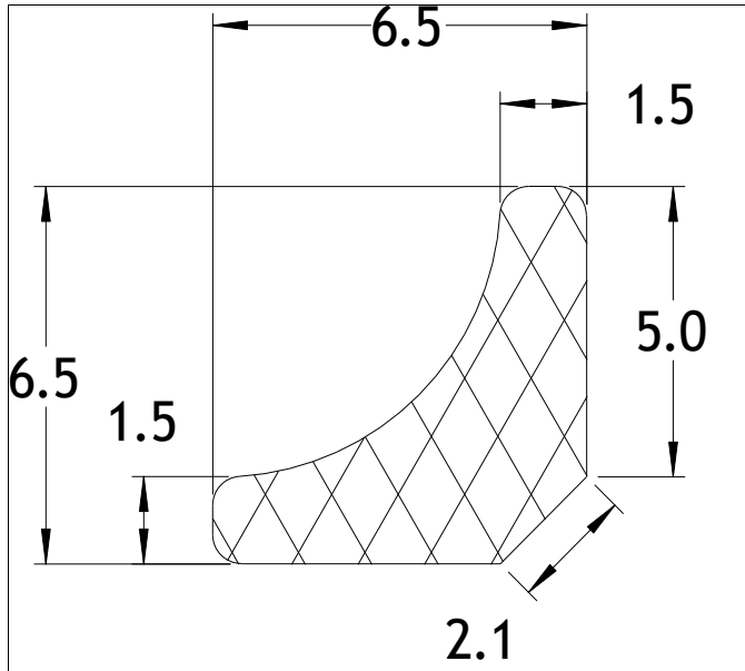
Die No: 7464 Category: L-Section
