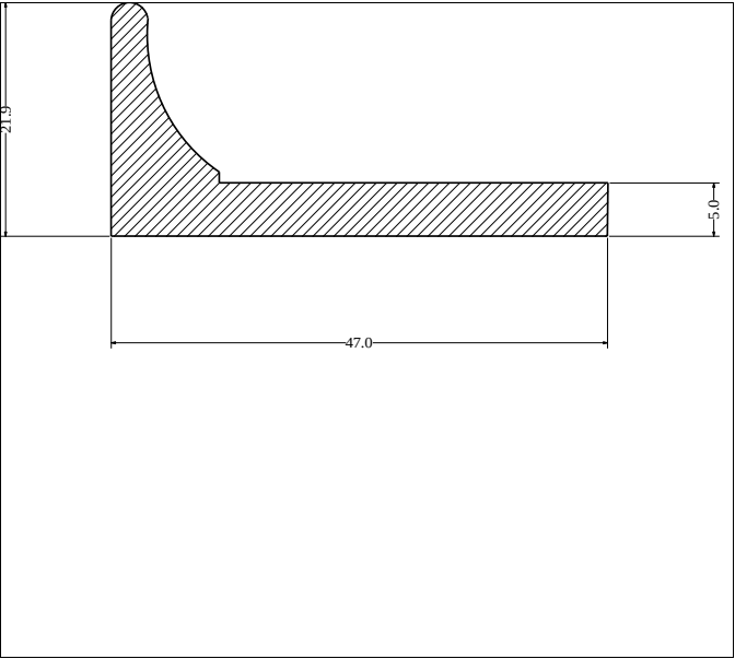
Die No: 404 Category: L-Section
