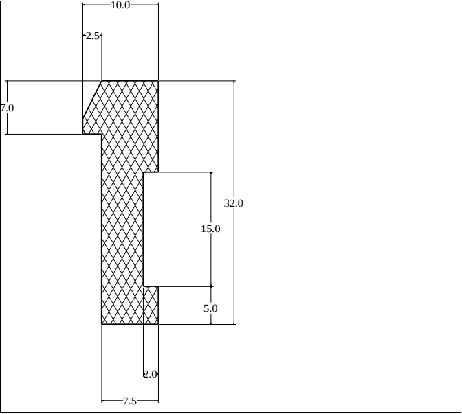
Die No: 3722 Category: L-Section
