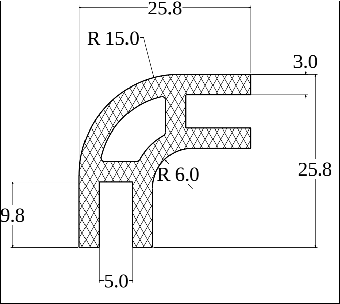
Die No: 2507 Category: L-Section
