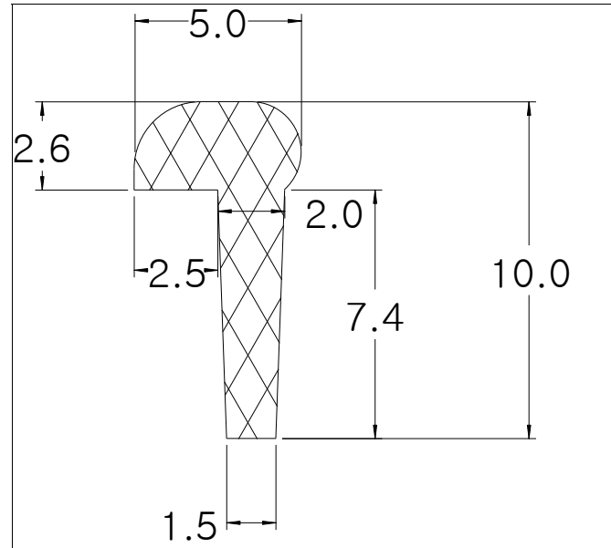
Die No: 8842 Category: L-Section
