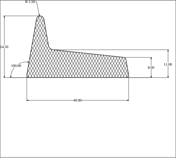
Die No: 3564 Category: L-Section
