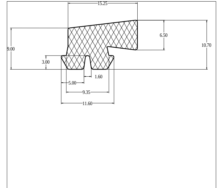
Die No: 9182 Category: L-Section
