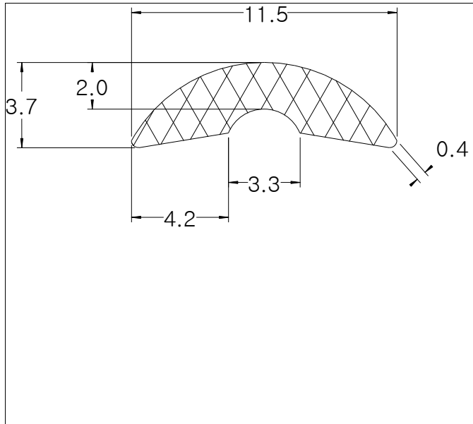
Die No: 8839 Category: L-Section
