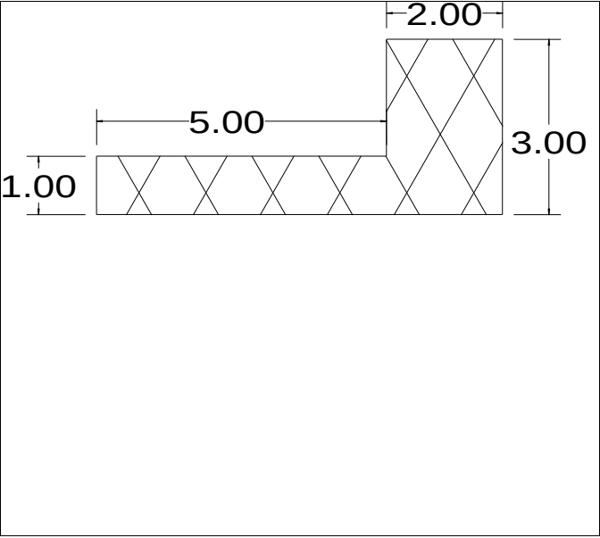
Die No: 5642 Category: L-Section
