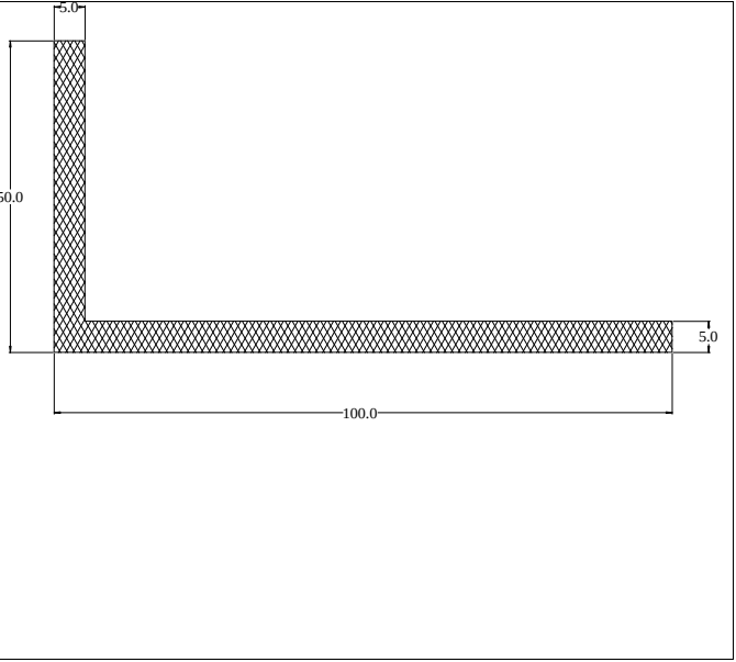
Die No: 4991 Category: L-Section
