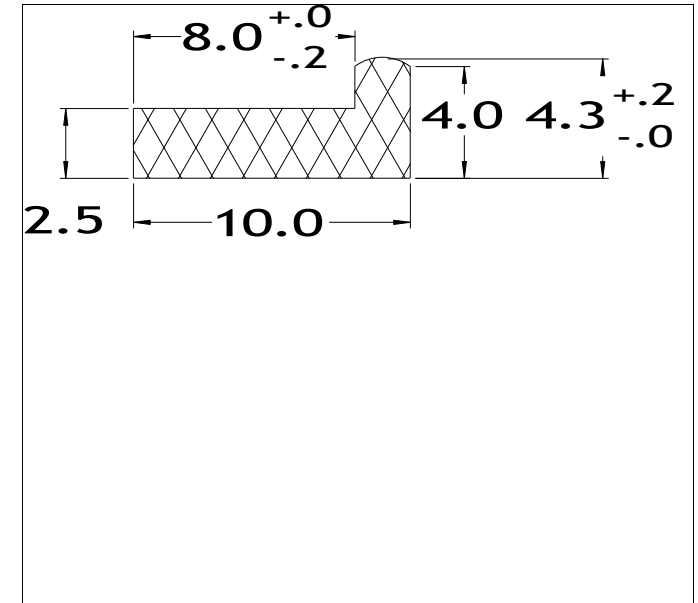
Die No: 7804 Category: L-Section
