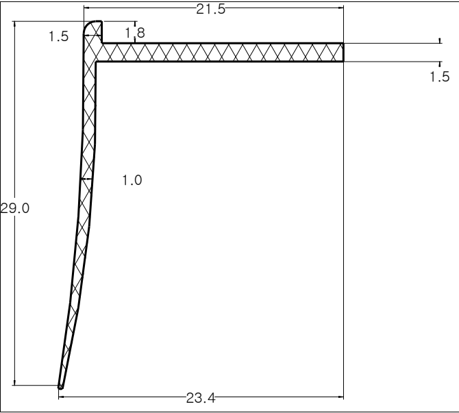
Die No: 7971 Category: L-Section
