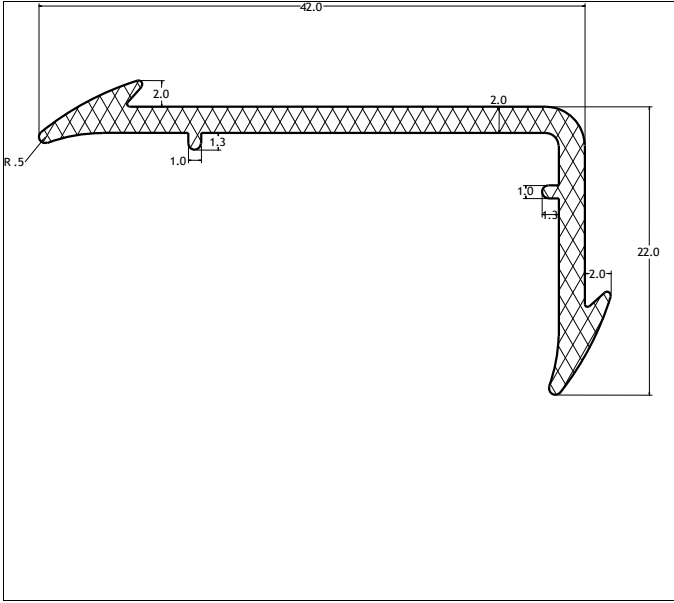
Die No: 7354 Category: L-Section
