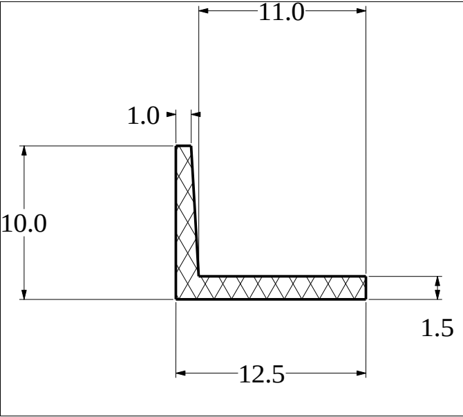
Die No: 3476 Category: L-Section
