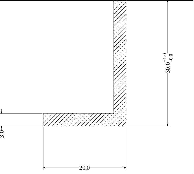
Die No: 409 Category: L-Section
