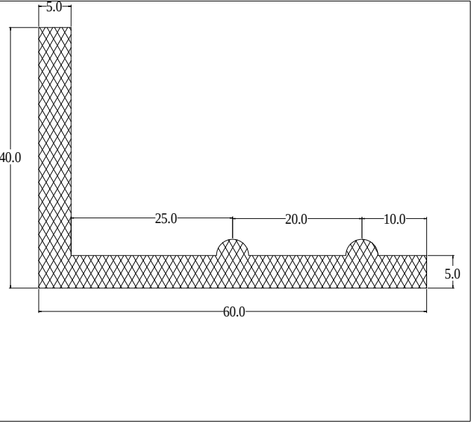
Die No: 9398 Category: L-Section
