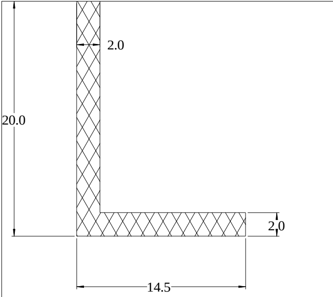
Die No: 5501 Category: L-Section
