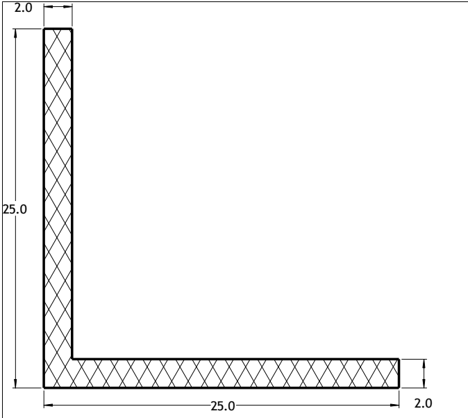
Die No: 6516 Category: L-Section
