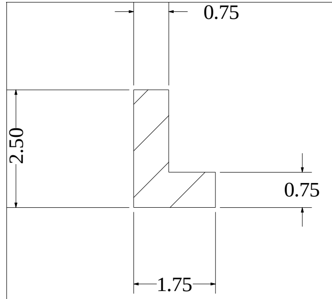
Die No: 1722 Category: L-Section
