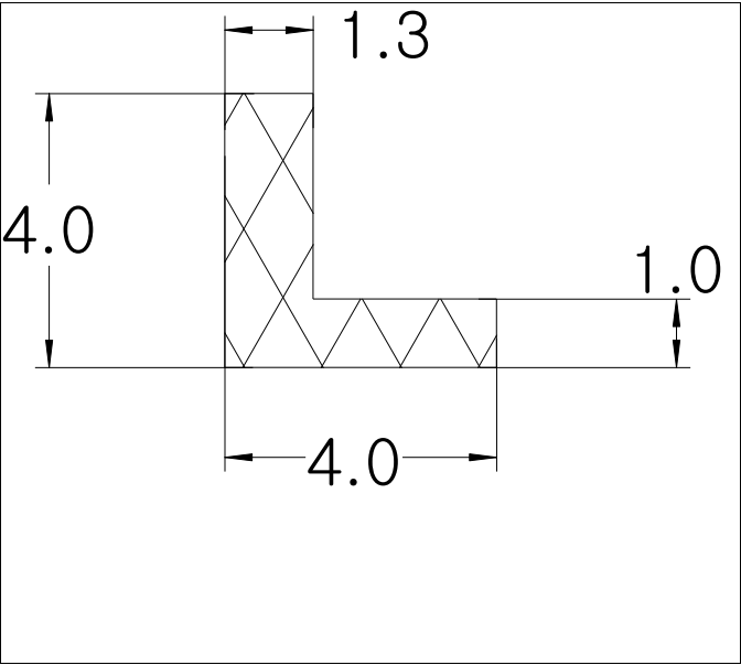
Die No: 7929 Category: L-Section
