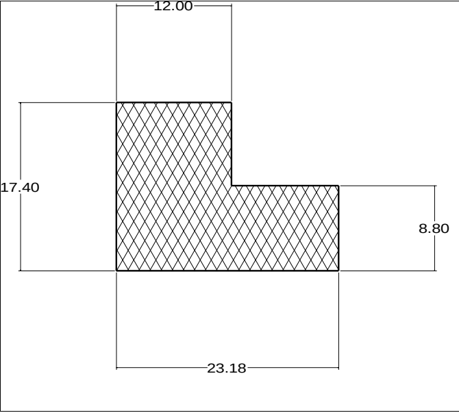
Die No: 4242 Category: L-Section
