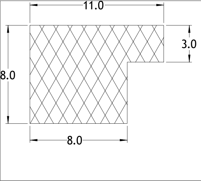
Die No: 6303 Category: L-Section
