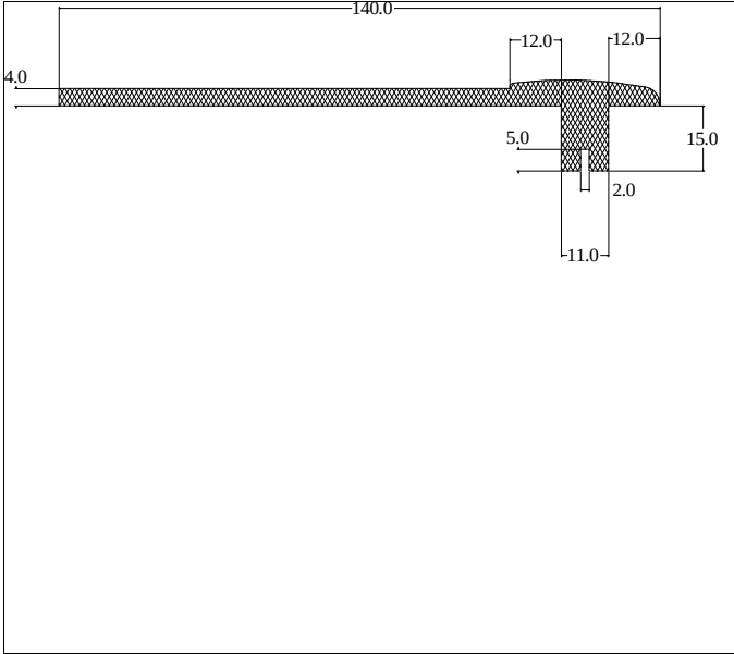
Die No: 1997 Category: L-Section
