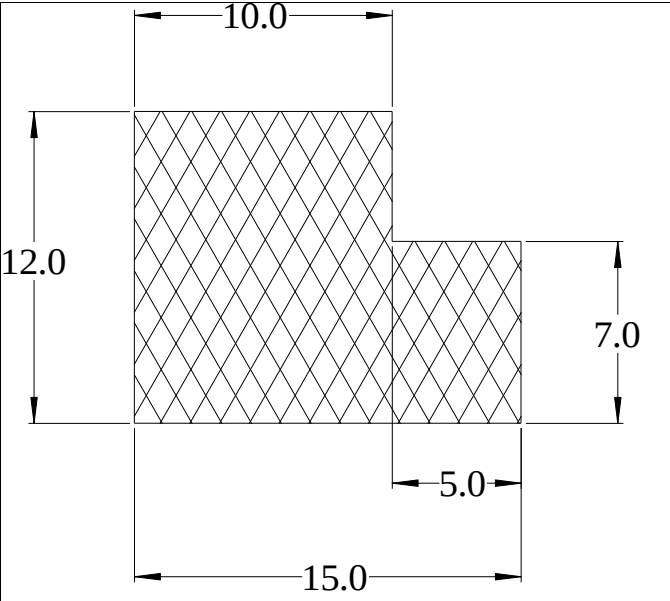
Die No: 5458 Category: L-Section
