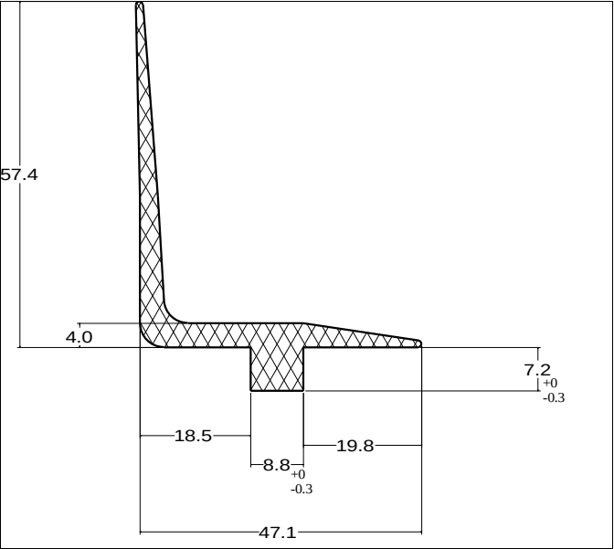
Die No: 4591 Category: L-Section
