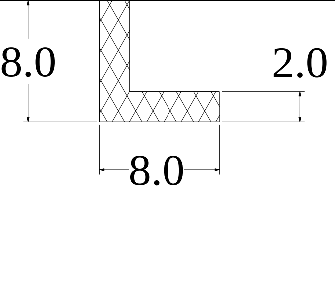
Die No: 2348 Category: L-Section
