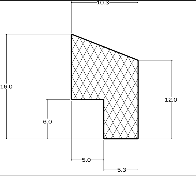
Die No: 4814 Category: L-Section
