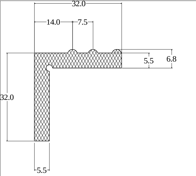
Die No: 2680 Category: L-Section
