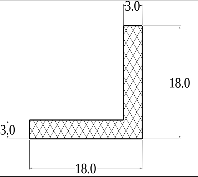
Die No: 9615 Category: L-Section
