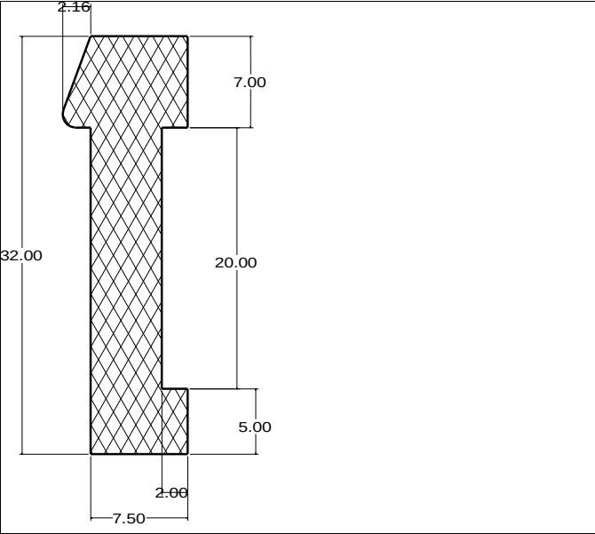
Die No: 4023 Category: L-Section
