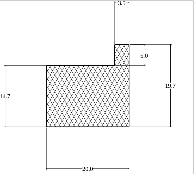
Die No: 3903 Category: L-Section
