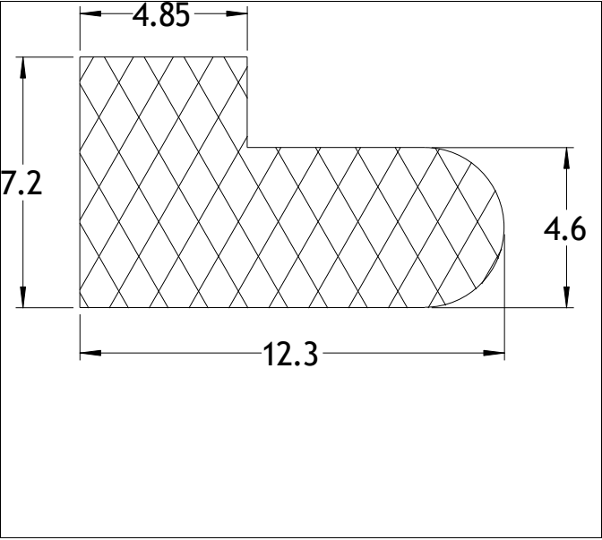
Die No: 7005 Category: L-Section
