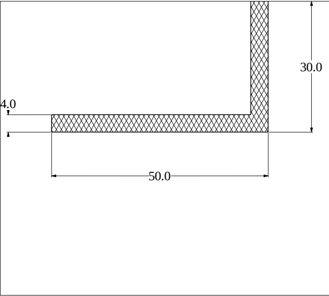
Die No: 2802 Category: L-Section
