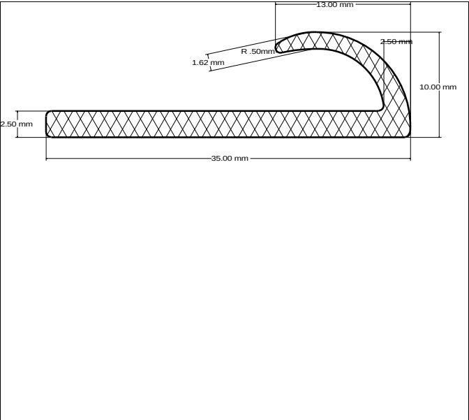
Die No: 4017 Category: L-Section
