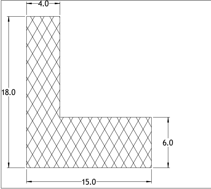
Die No: 6746 Category: L-Section
