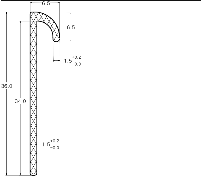
Die No: 8455 Category: L-Section
