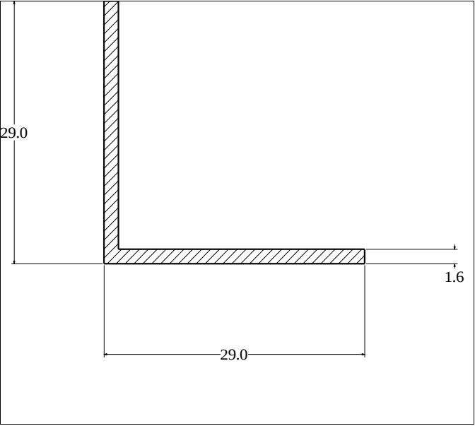
Die No: 751 Category: L-Section
