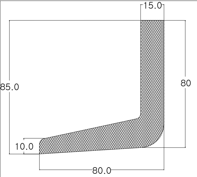
Die No: 8439 Category: L-Section
