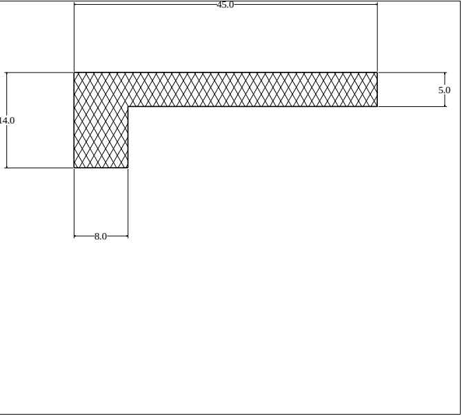
Die No: 3631 Category: L-Section
