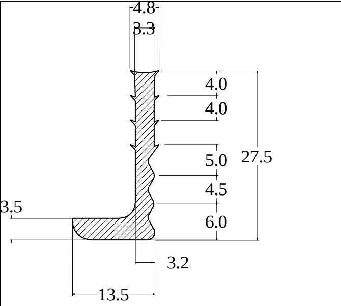
Die No: 1937 Category: L-Section
