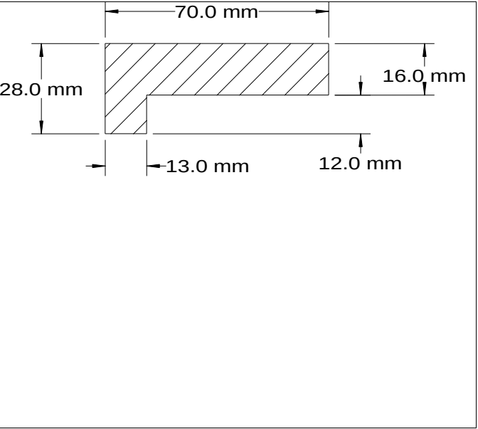
Die No: 3736 Category: L-Section
