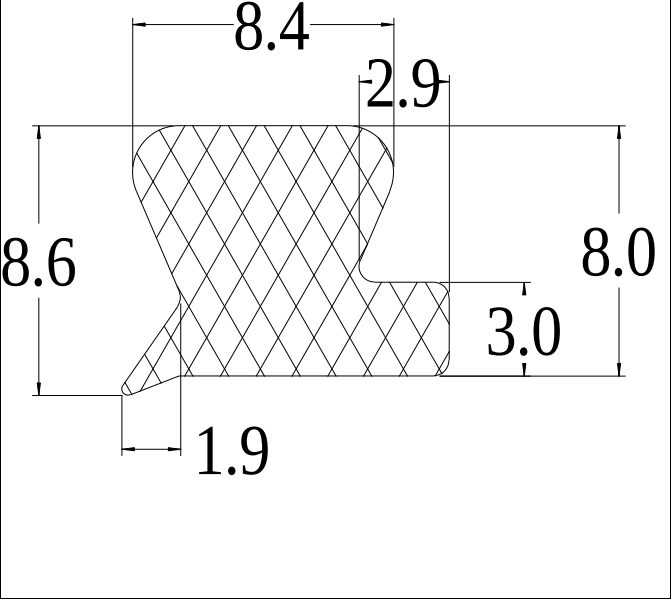
Die No: 9653 Category: L-Section
