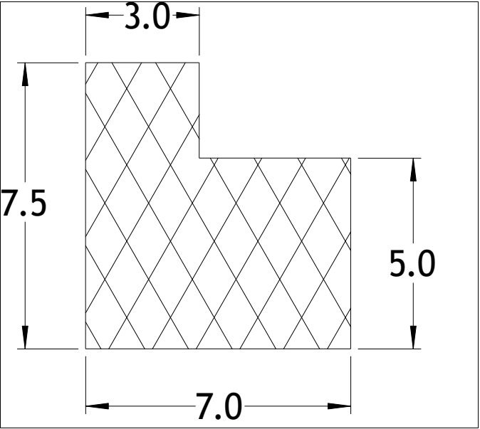
Die No: 6274 Category: L-Section
