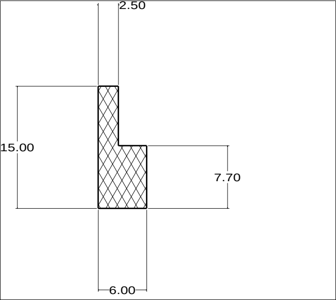
Die No: 4533 Category: L-Section
