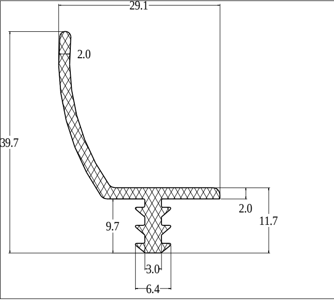
Die No: 9981 Category: L-Section
