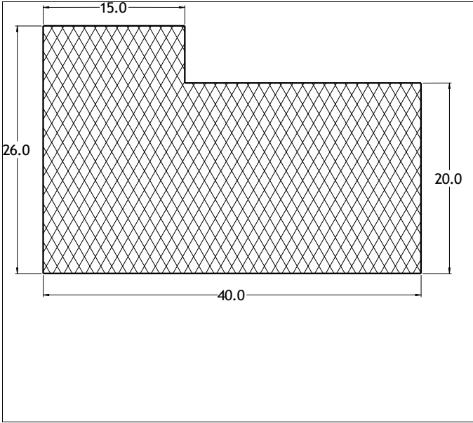
Die No: 7083 Category: L-Section
