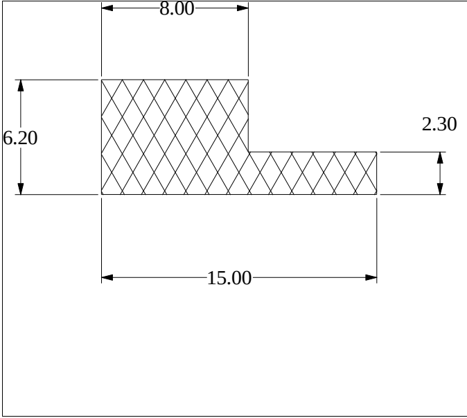
Die No: 3526 Category: L-Section
