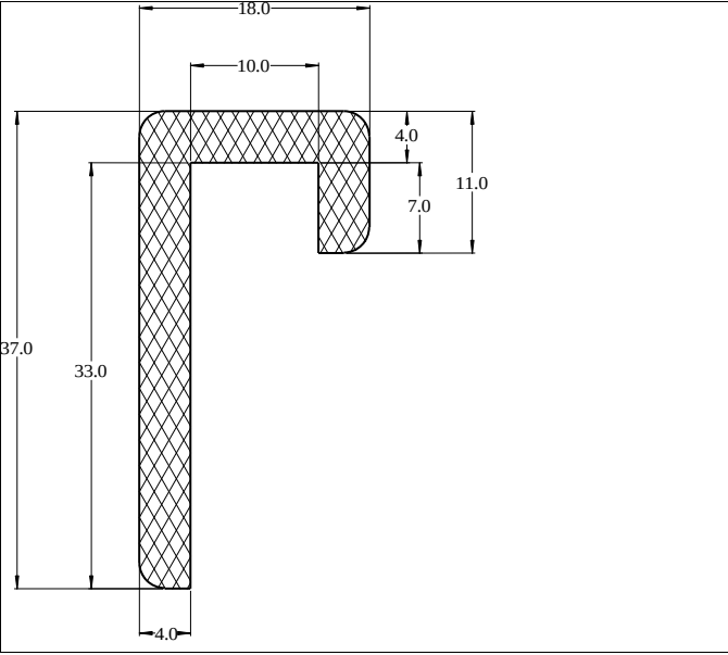
Die No: 4948 Category: L-Section
