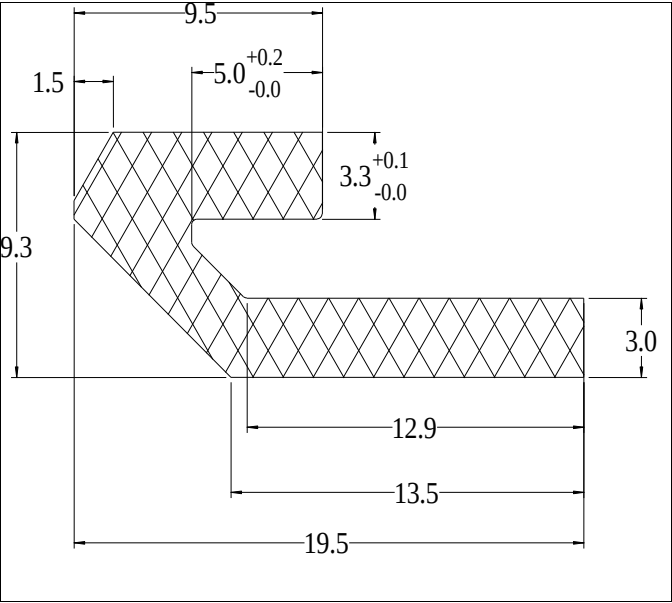
Die No: 9979 Category: L-Section
