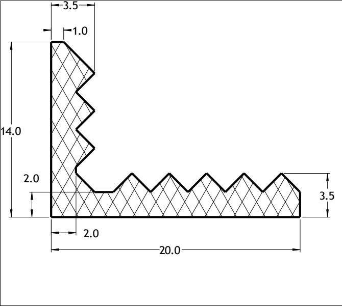
Die No: 6707 Category: L-Section
