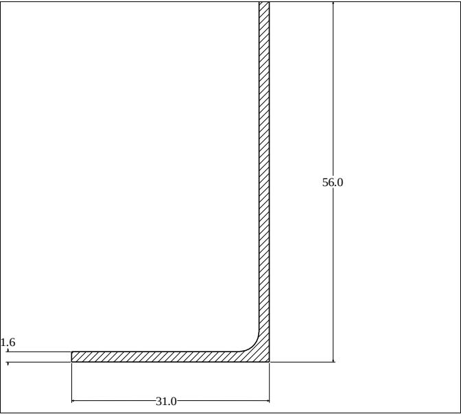
Die No: 1095 Category: L-Section
