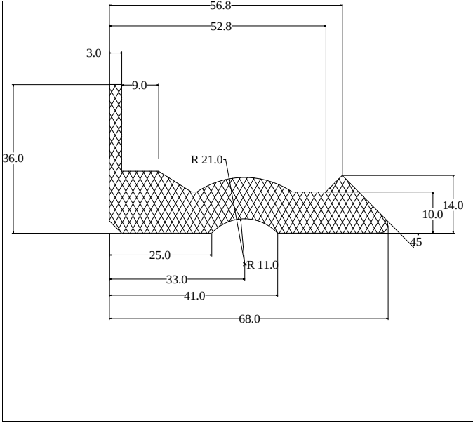
Die No: 2422 Category: L-Section
