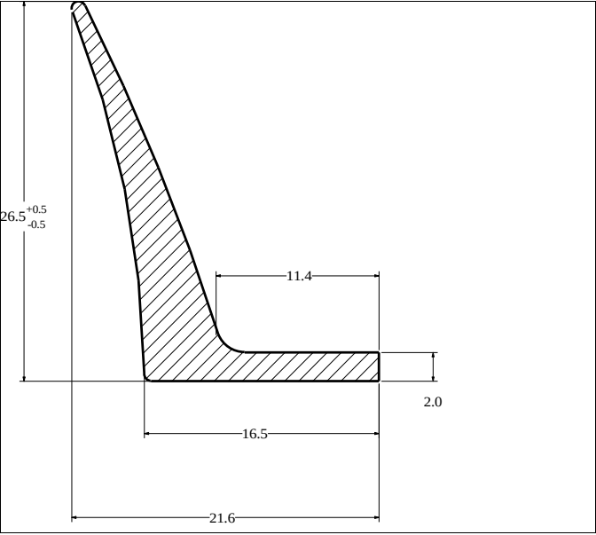
Die No: 403 Category: L-Section
