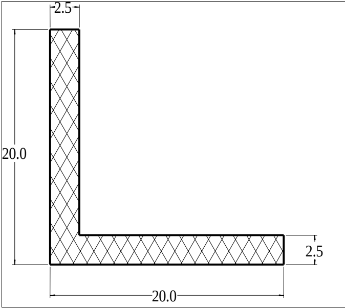
Die No: 9982 Category: L-Section
