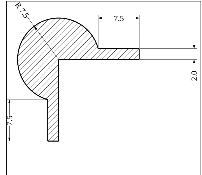
Die No: 1787 Category: L-Section
