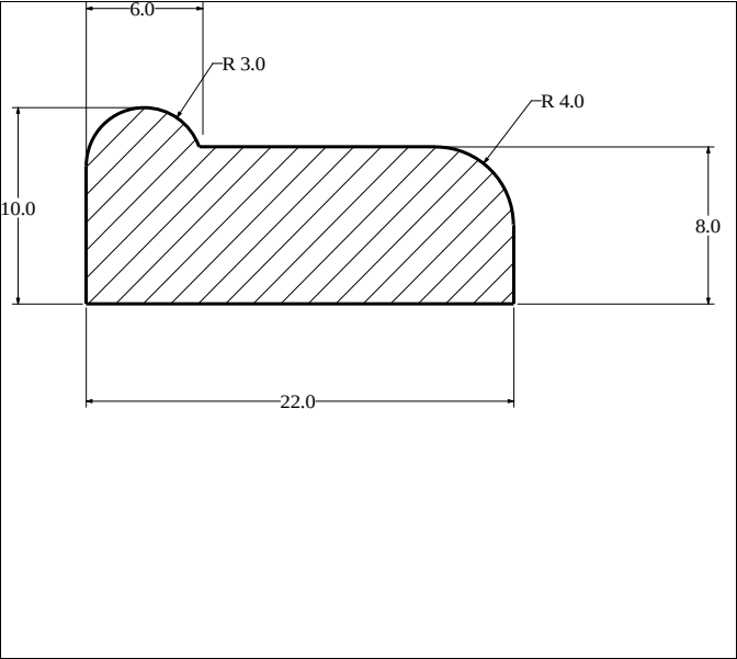
Die No: 1934 Category: L-Section
