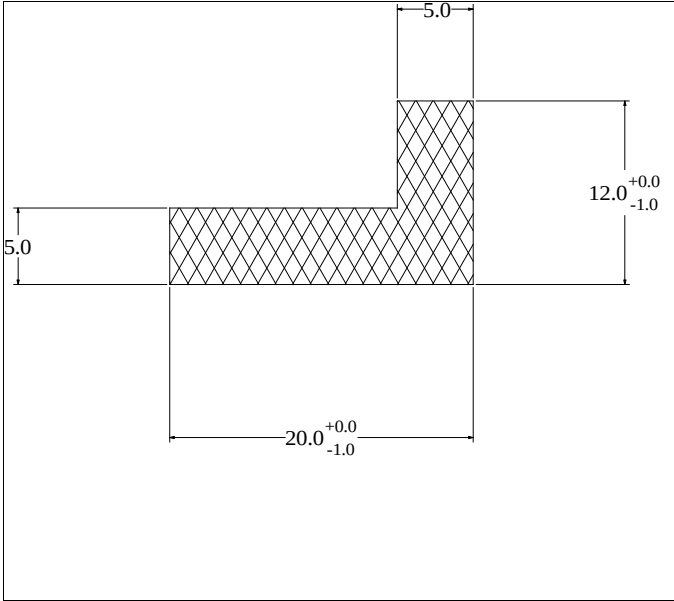
Die No: 2694 Category: L-Section
