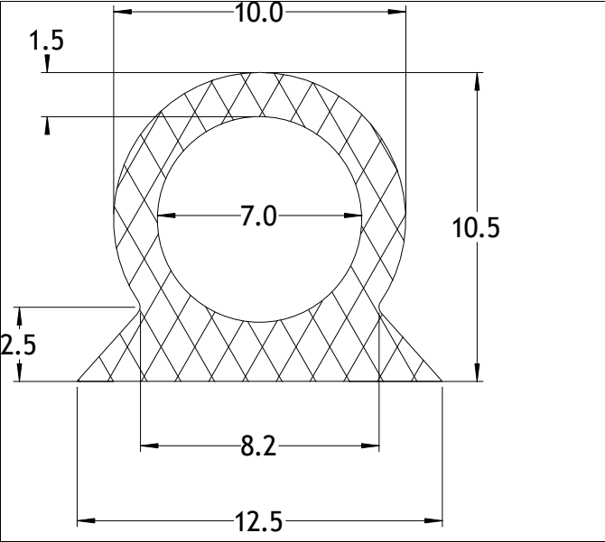
Die No: 7174 Category: Key-Hole
