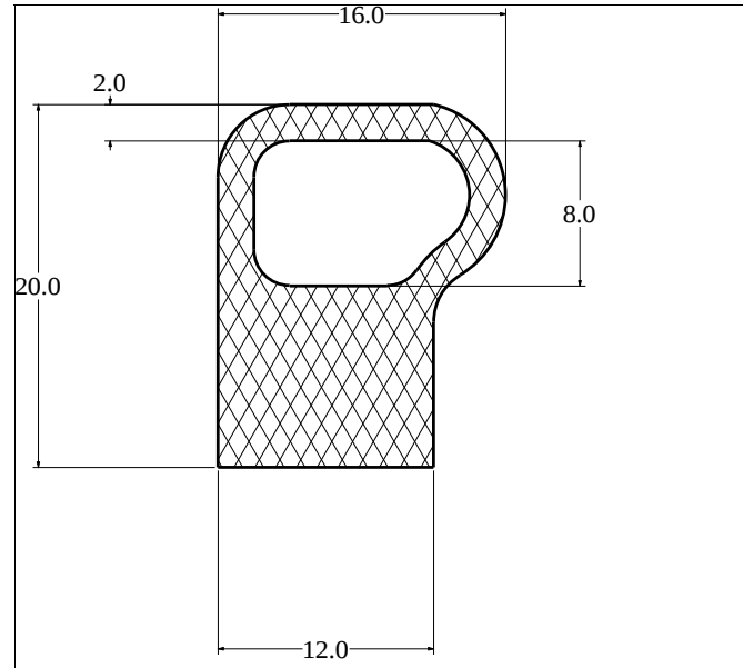
Die No: 3034 Category: Key-Hole
