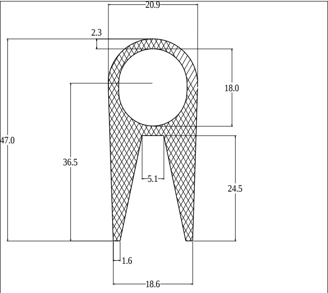
Die No: 9937 Category: Key-Hole
