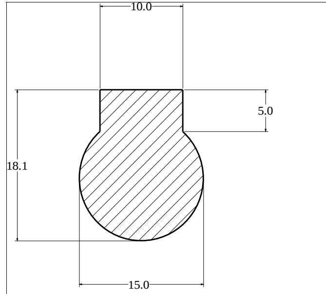
Die No: 1385 Category: Key-Hole
