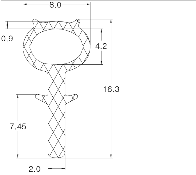
Die No: 8589 Category: Key-Hole
