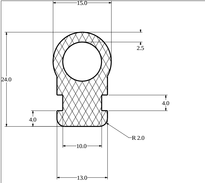
Die No: 2369 Category: Key-Hole
