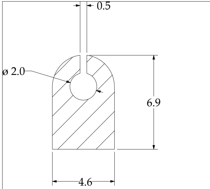
Die No: 1274 Category: Key-Hole
