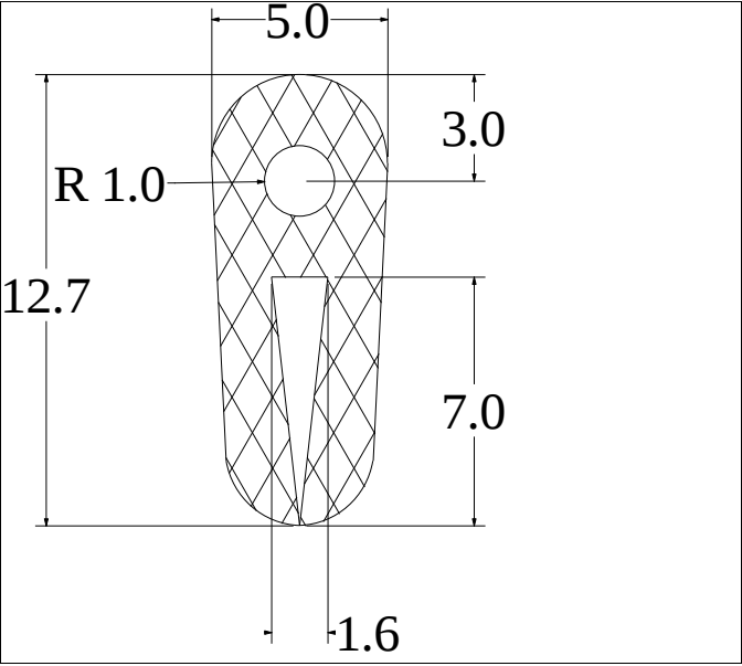
Die No: 3946 Category: Key-Hole
