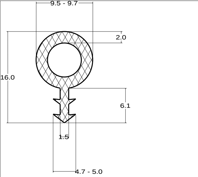
Die No: 4864 Category: Key-Hole
