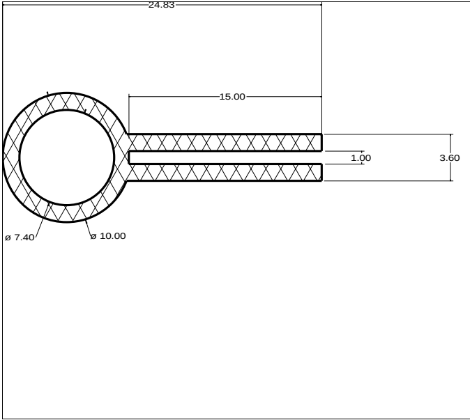
Die No: 4344 Category: Key-Hole
