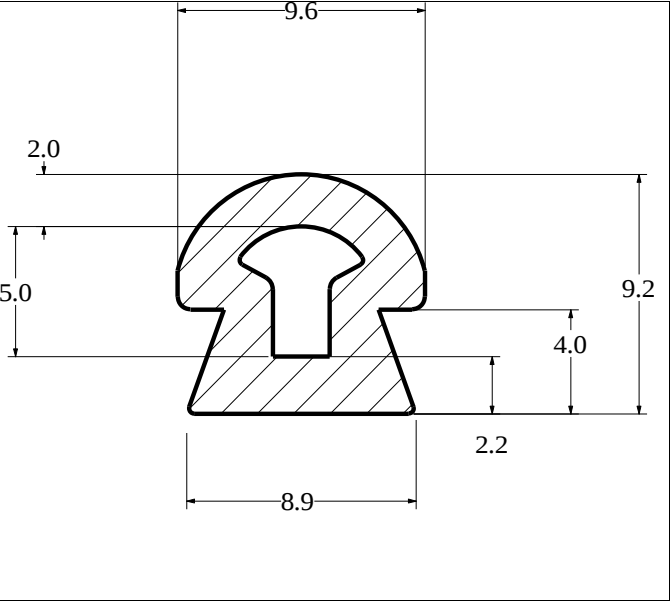
Die No: 1962 Category: Key-Hole
