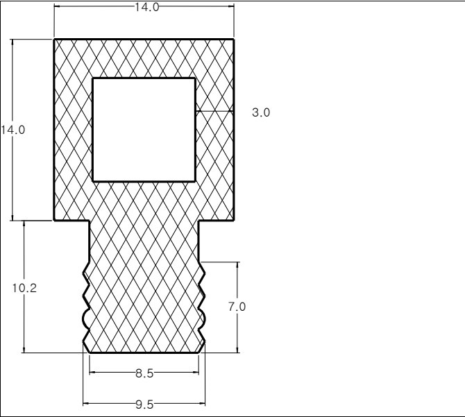
Die No: 8579 Category: Key-Hole
