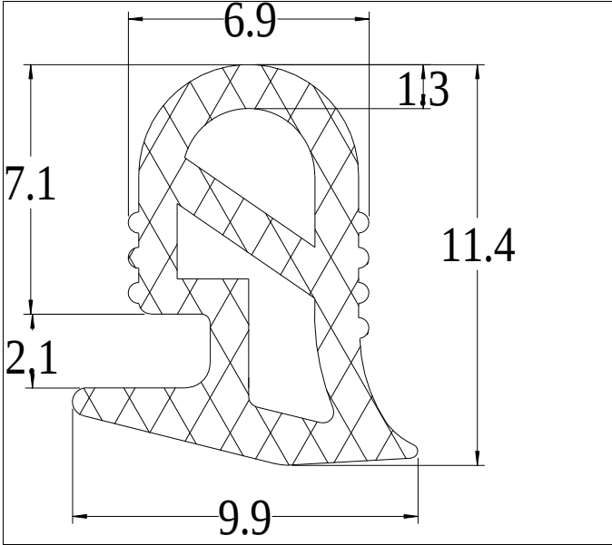
Die No: 9592 Category: Key-Hole
