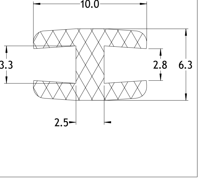
Die No: 7042 Category: H-section
