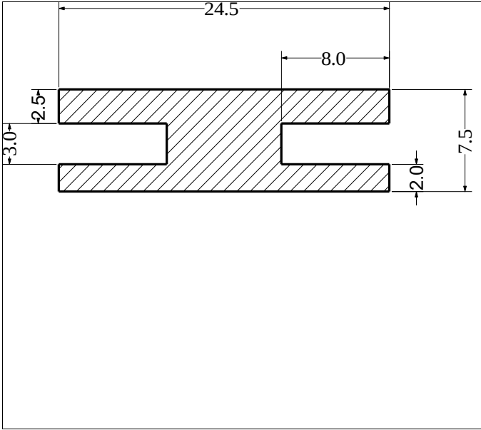
Die No: 564 Category: H-section
