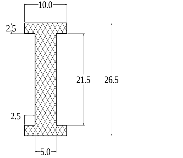
Die No: 9314 Category: H-section
