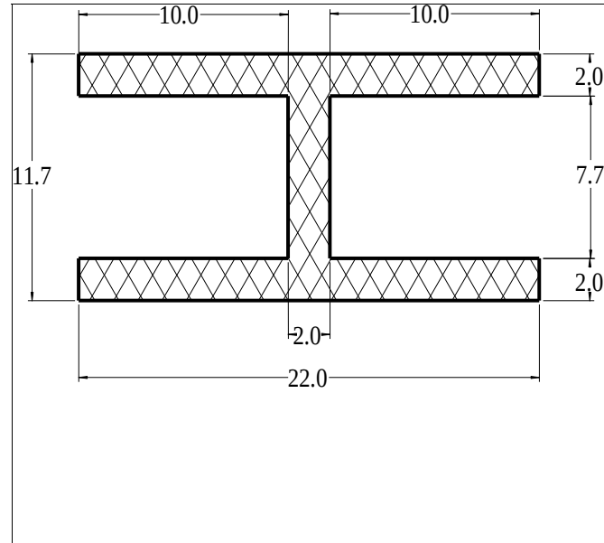
Die No: 9989 Category: H-section
