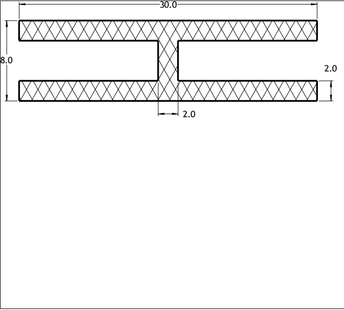
Die No: 6367 Category: H-section
