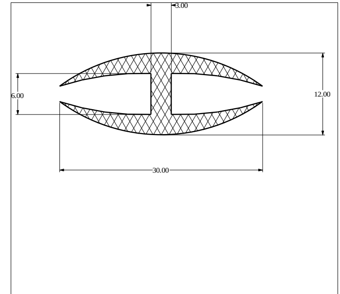
Die No: 3548 Category: H-section
