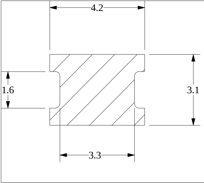
Die No: 1073 Category: H-section
