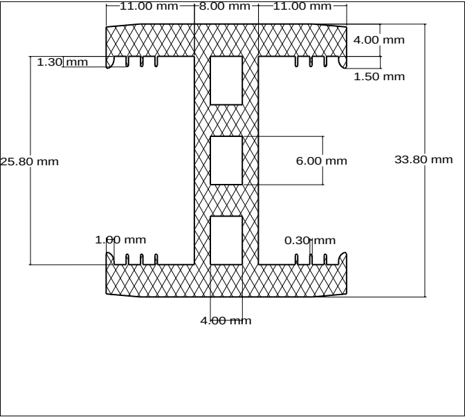
Die No: 3935 Category: H-section
