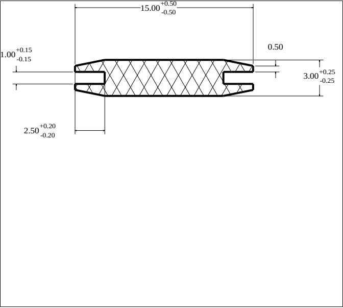
Die No: 3194 Category: H-section
