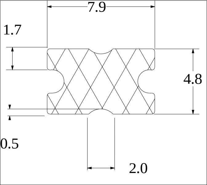
Die No: 2221 Category: H-section
