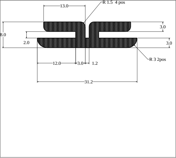
Die No: 2558 Category: H-section
