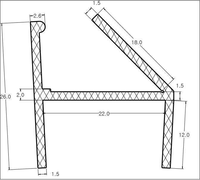
Die No: 8765 Category: H-section
