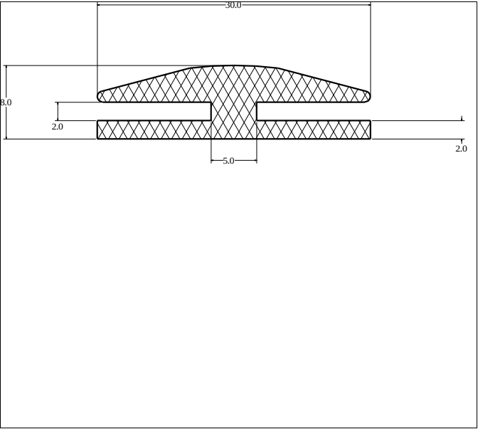
Die No: 3658 Category: H-section
