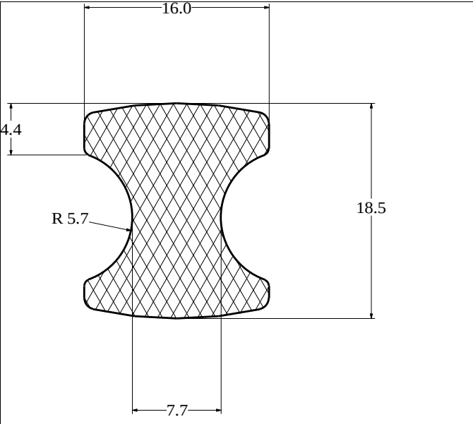
Die No: 2231 Category: H-section
