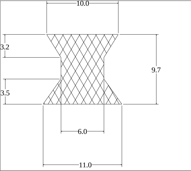
Die No: 3463 Category: H-section
