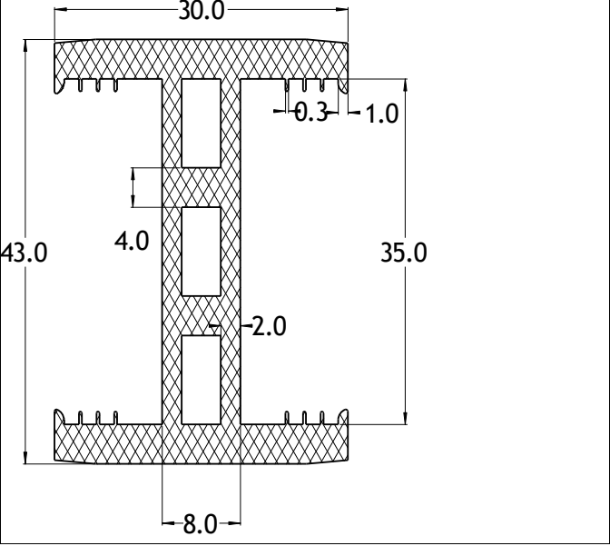
Die No: 6777 Category: H-section
