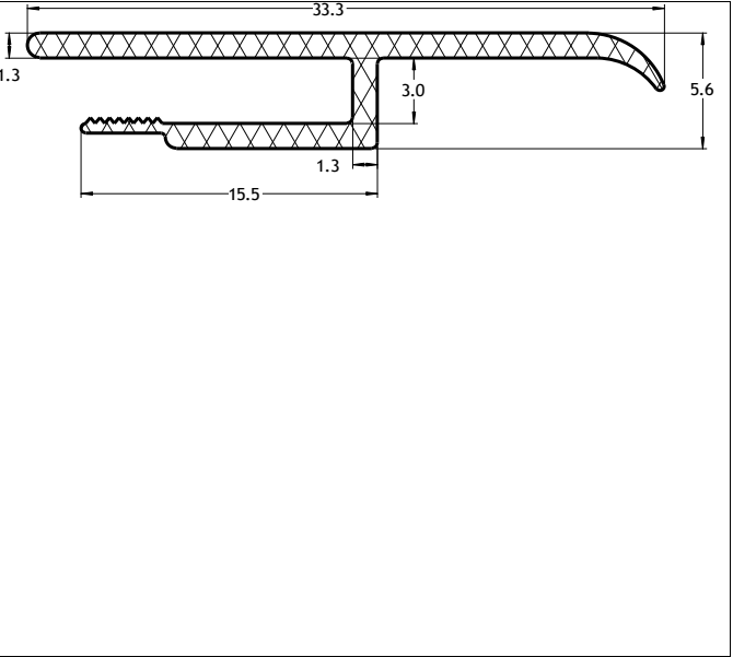
Die No: 6714 Category: H-section
