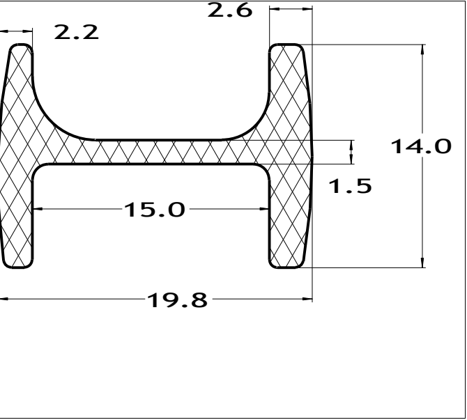
Die No: 7438 Category: H-section
