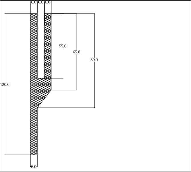
Die No: 4816 Category: H-section
