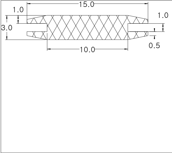
Die No: 8364 Category: H-section
