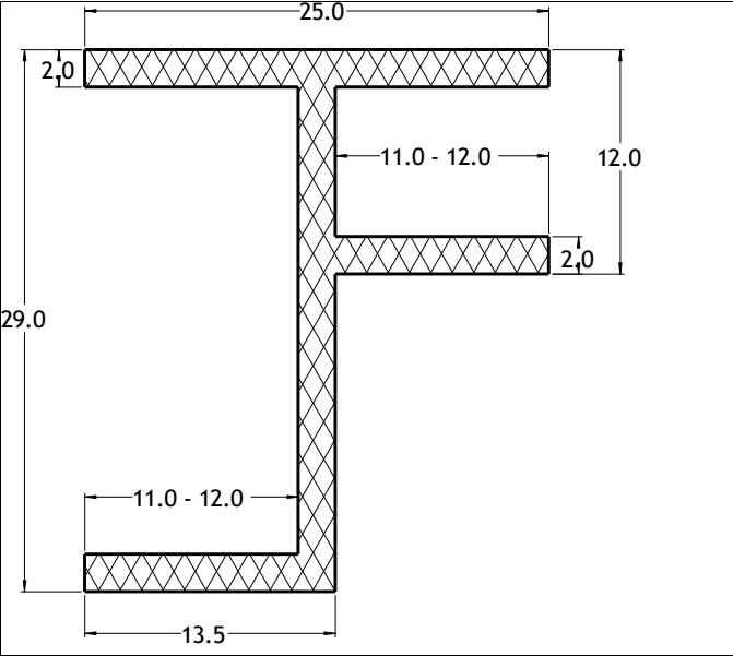
Die No: 6532 Category: H-section
