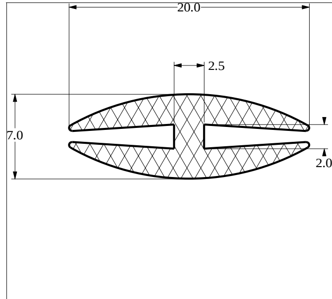
Die No: 3541 Category: H-section
