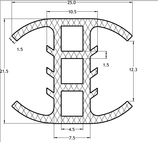
Die No: 6703 Category: H-section
