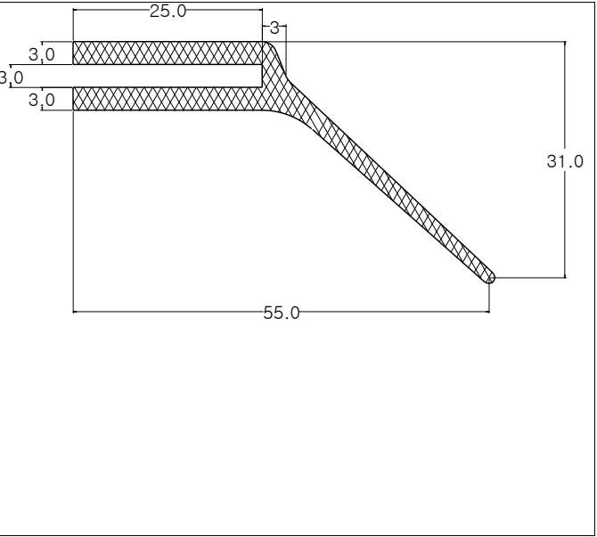
Die No: 8804 Category: H-section
