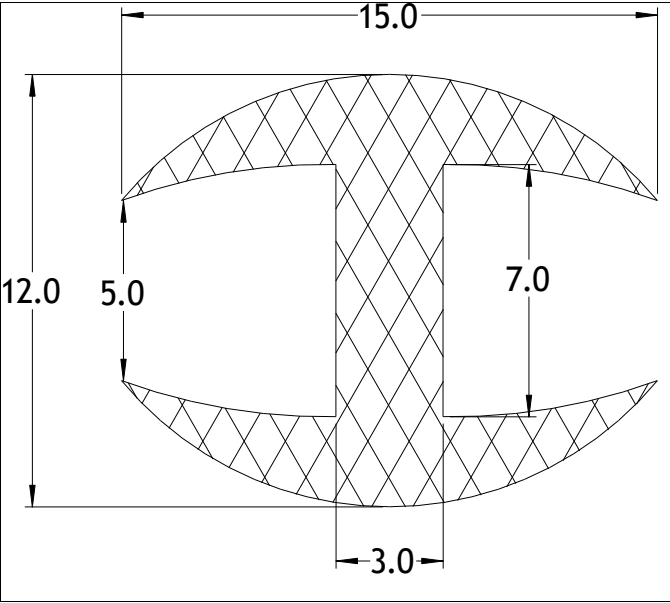
Die No: 6778 Category: H-section
