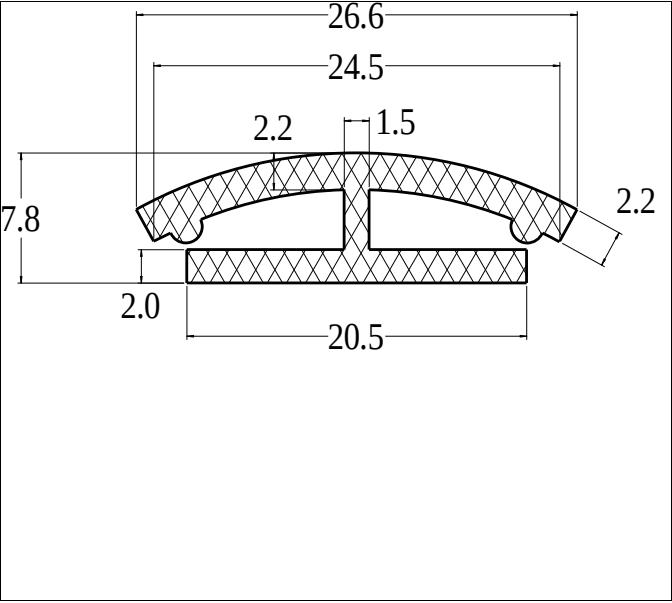
Die No: 8968 Category: H-section
