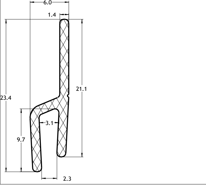
Die No: 6800 Category: H-section
