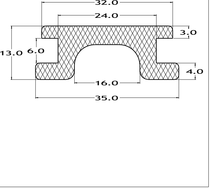
Die No: 7518 Category: H-section
