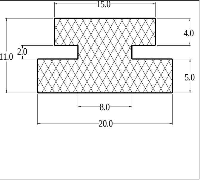
Die No: 9814 Category: H-section
