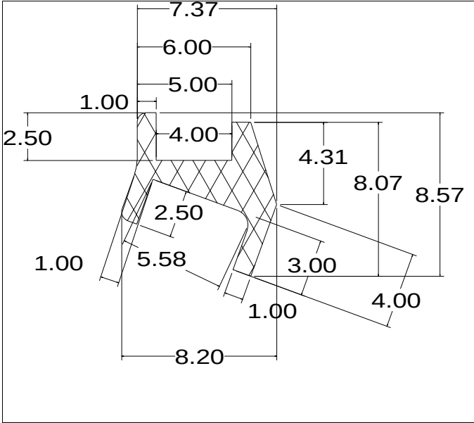
Die No: 5813 Category: H-section
