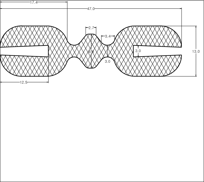
Die No: 8105 Category: H-section
