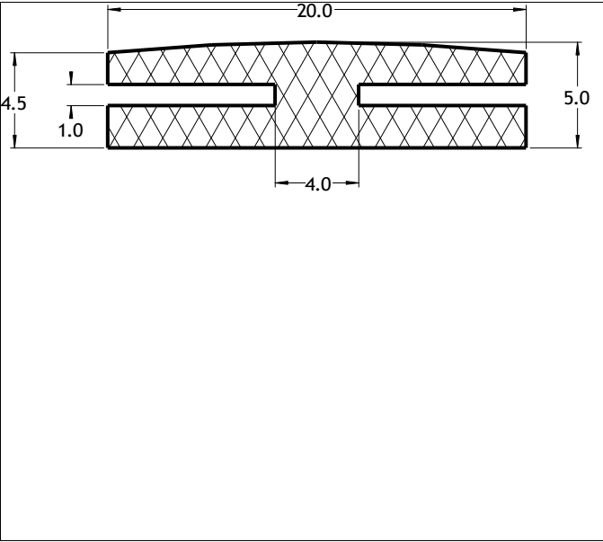
Die No: 6413 Category: H-section
