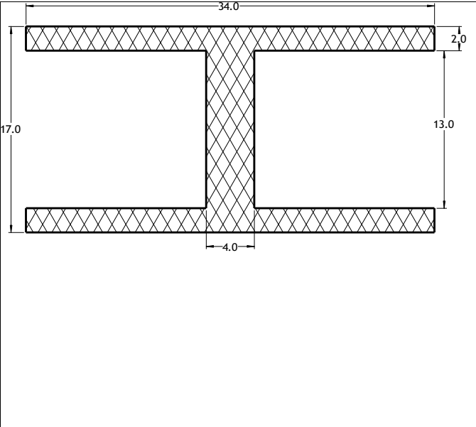
Die No: 6531 Category: H-section
