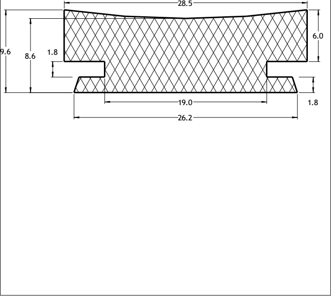
Die No: 6988 Category: H-section
