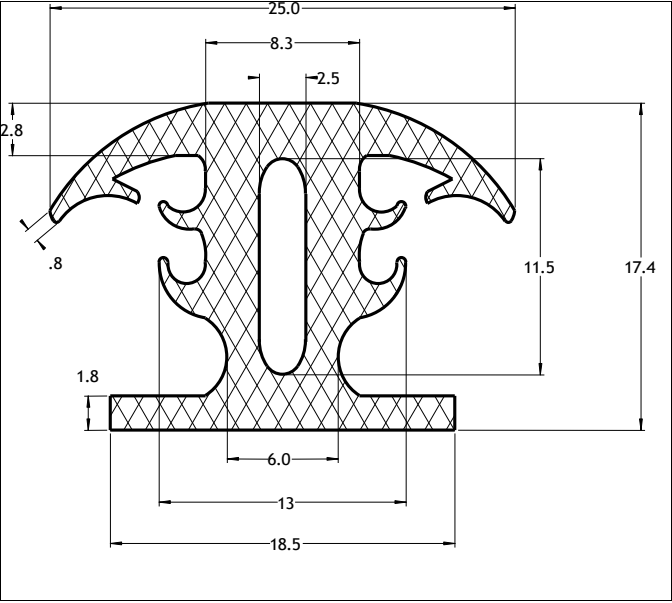
Die No: 6138 Category: H-section
