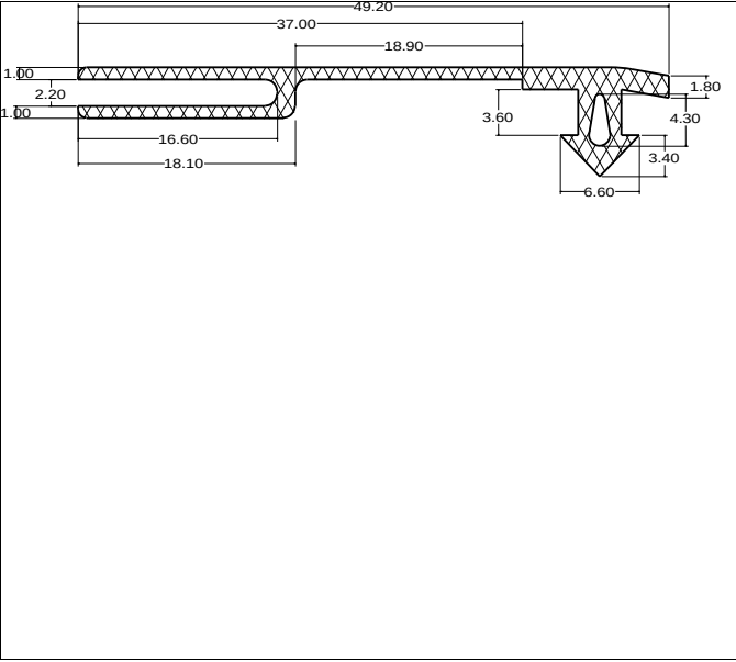
Die No: 4036 Category: H-section
