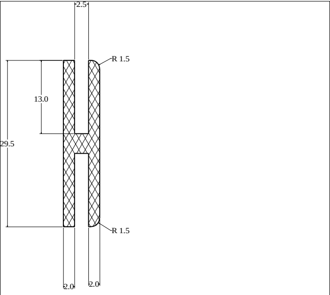
Die No: 3869 Category: H-section
