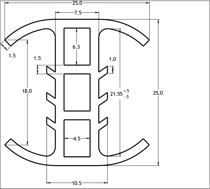
Die No: 6335 Category: H-section
