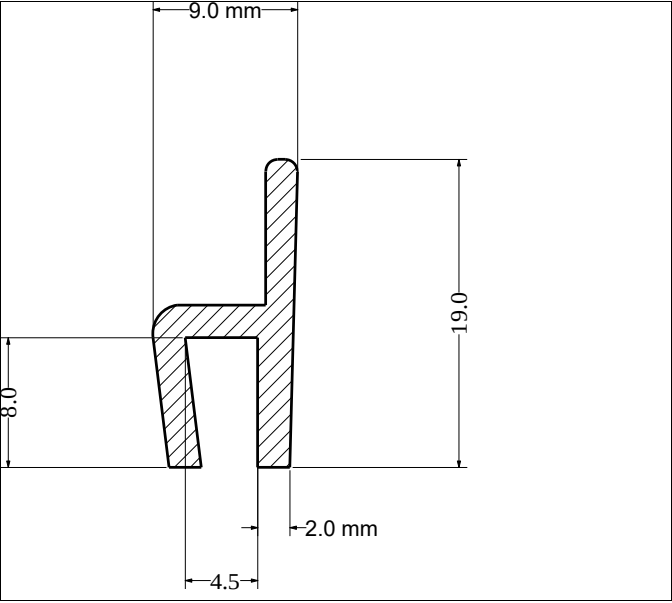
Die No: 260 Category: H-section
