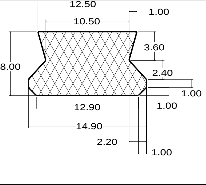
Die No: 5987 Category: T-Section
