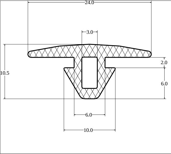
Die No: 3731 Category: T-Section
