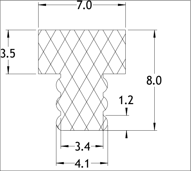
Die No: 6361 Category: T-Section
