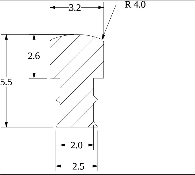
Die No: 1908 Category: T-Section
