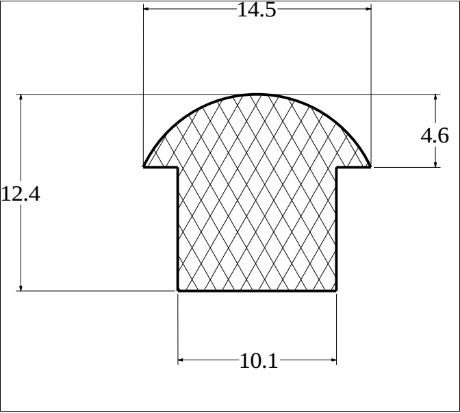
Die No: 2968 Category: T-Section
