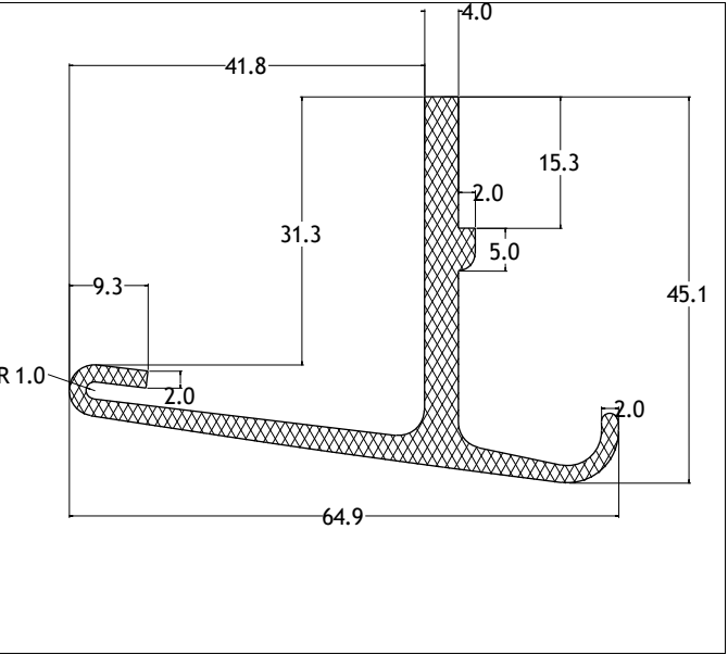
Die No: 7372 Category: T-Section
