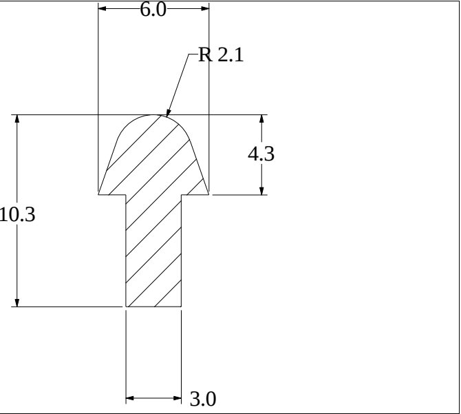
Die No: 2081 Category: T-Section
