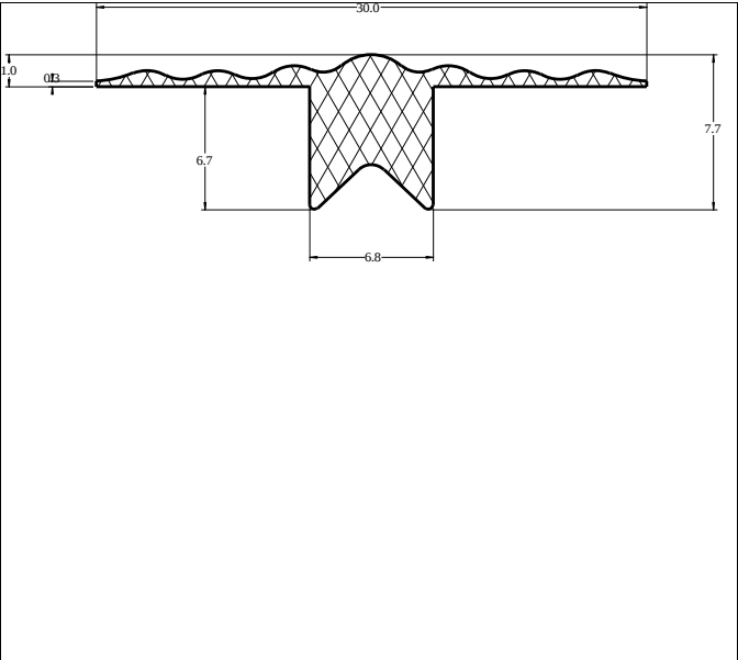
Die No: 5183 Category: T-Section
