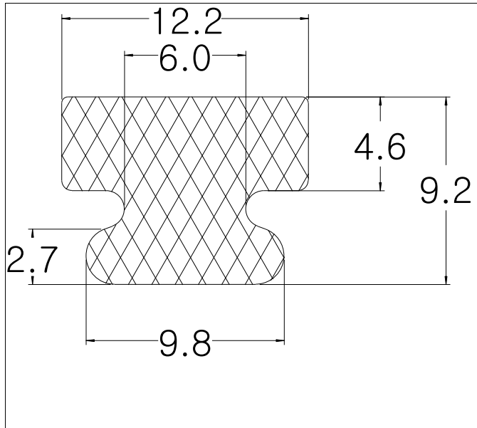
Die No: 8909 Category: T-Section
