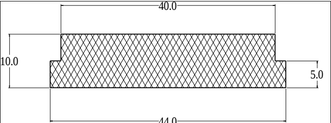
Die No: 9679 Category: T-Section
