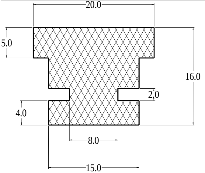
Die No: 9702 Category: T-Section
