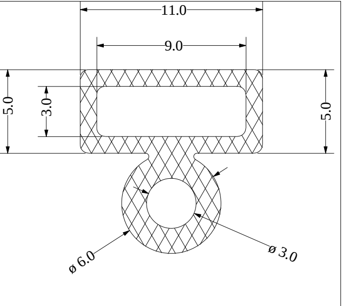
Die No: 1031 Category: T-Section
