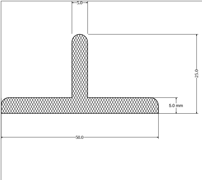
Die No: 645 Category: T-Section
