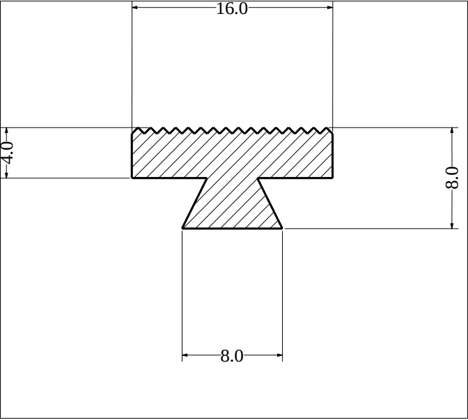
Die No: 175 Category: T-Section
