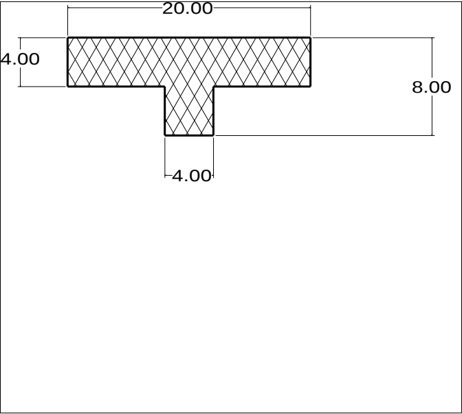
Die No: 4022 Category: T-Section
