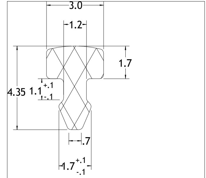
Die No: 6504 Category: T-Section
