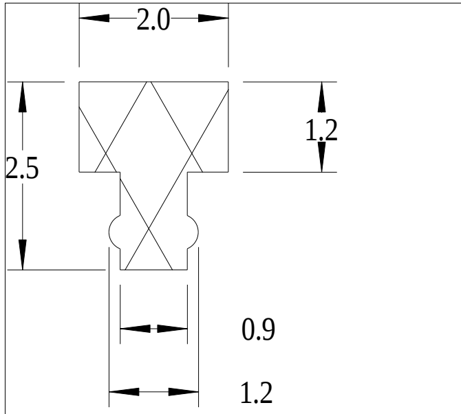
Die No: 9972 Category: T-Section
