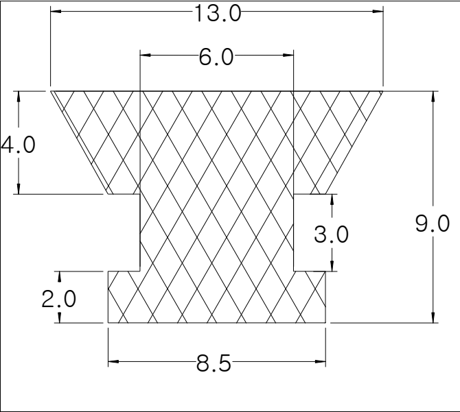
Die No: 8316 Category: T-Section
