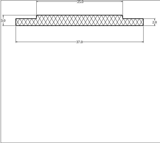
Die No: 5050 Category: T-Section
