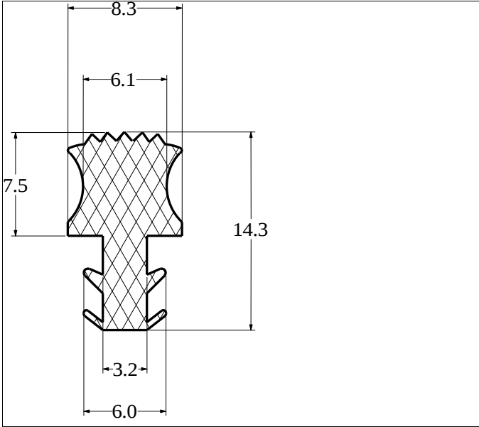
Die No: 2249 Category: T-Section
