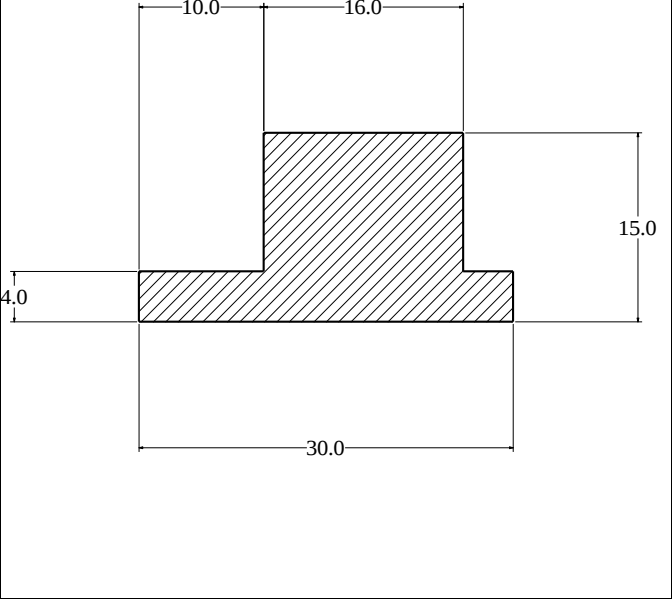
Die No: 1906 Category: T-Section
