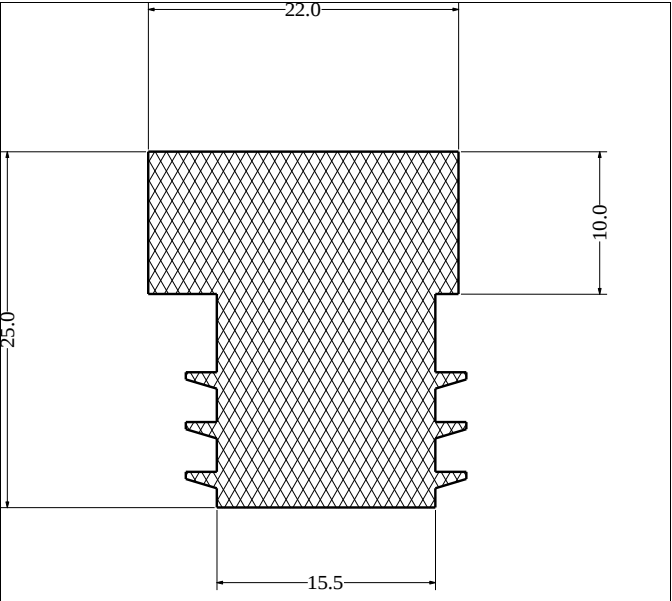
Die No: 1009 Category: T-Section
