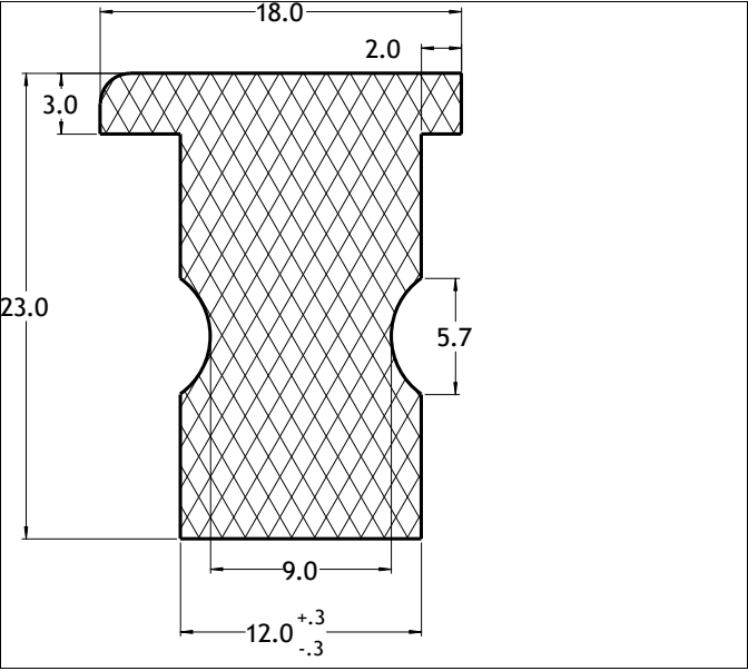
Die No: 7087 Category: T-Section
