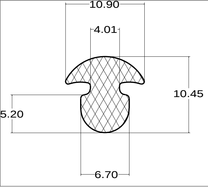
Die No: 4427 Category: T-Section
