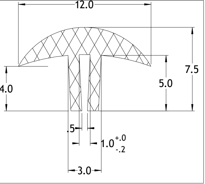
Die No: 7105 Category: T-Section
