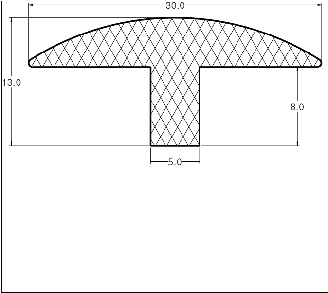
Die No: 7777 Category: T-Section
