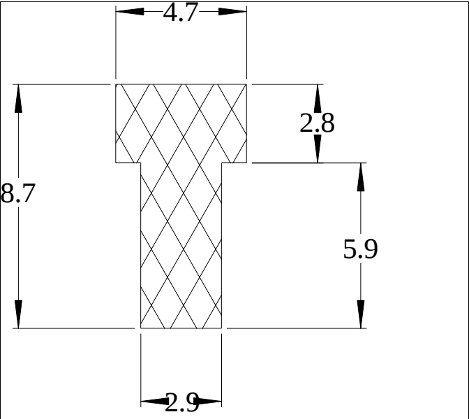
Die No: 4892 Category: T-Section
