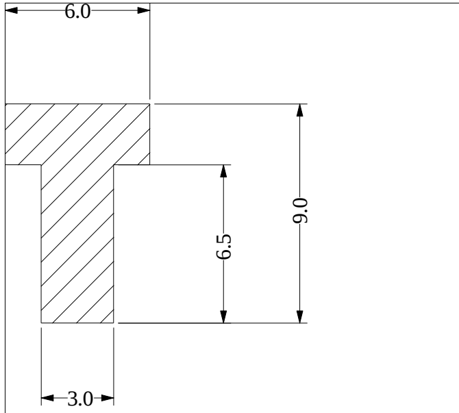
Die No: 1692 Category: T-Section
