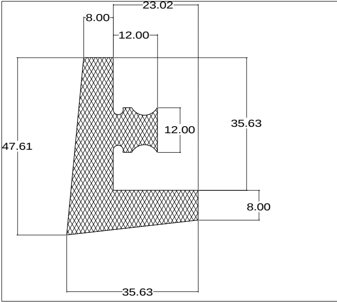
Die No: 4434 Category: T-Section
