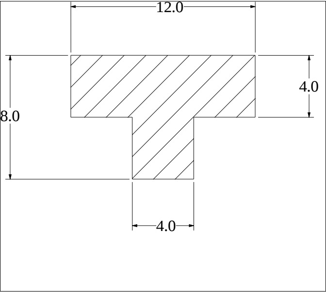
Die No: 1968 Category: T-Section
