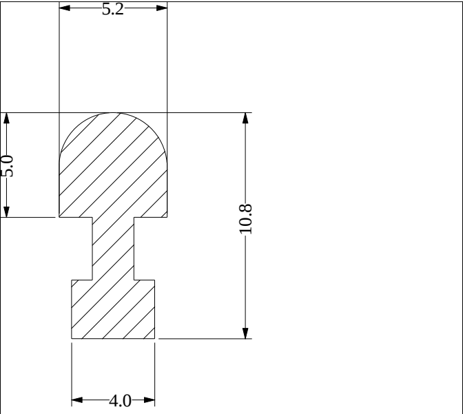
Die No: 618 Category: T-Section
