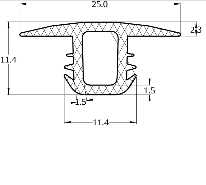
Die No: 5257 Category: T-Section
