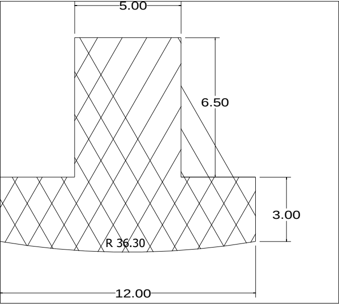
Die No: 5614 Category: T-Section
