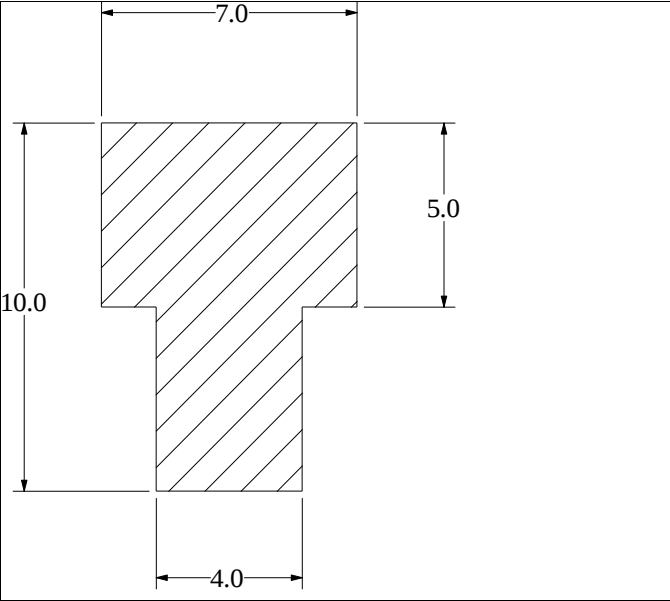
Die No: 1853 Category: T-Section
