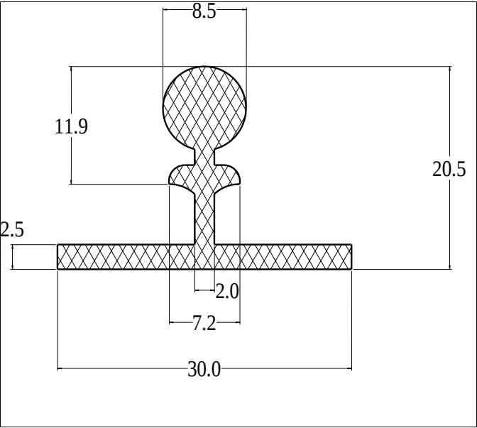
Die No: 9141 Category: T-Section
