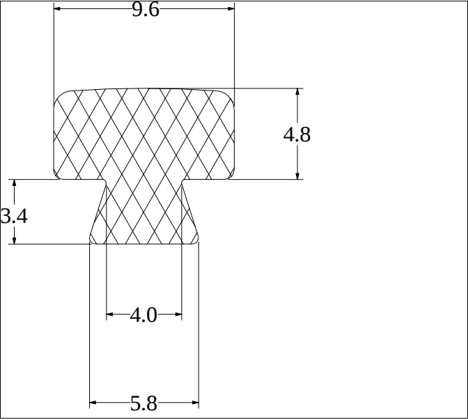
Die No: 3349 Category: T-Section
