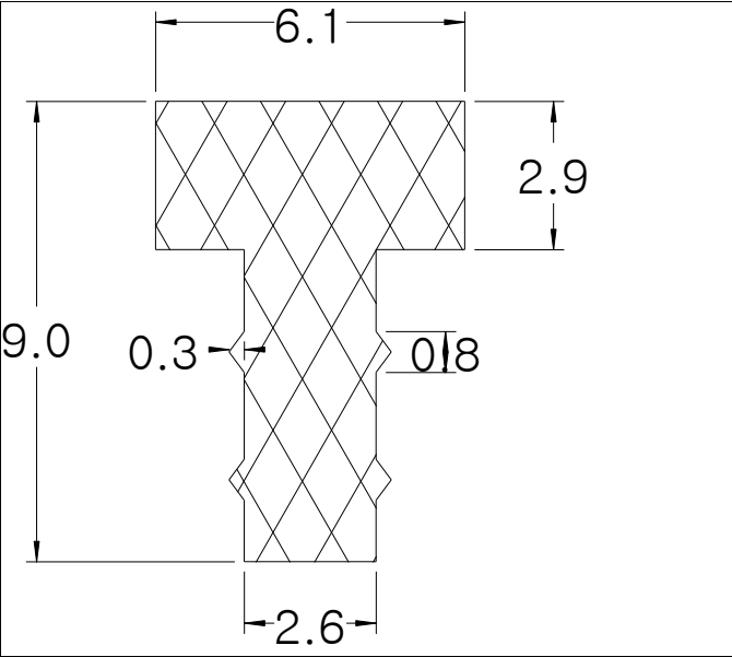
Die No: 7867 Category: T-Section
