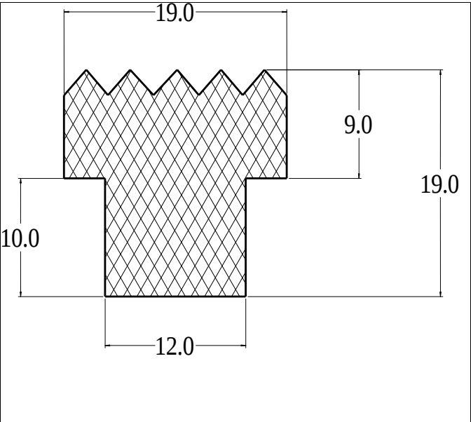
Die No: 9856 Category: T-Section
