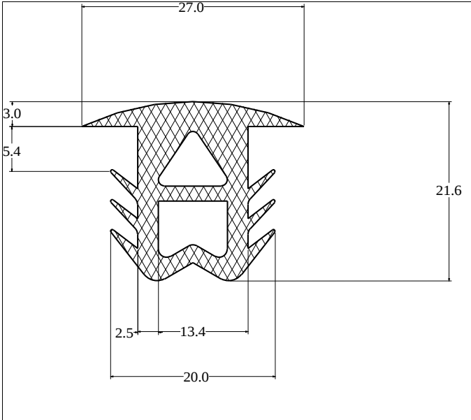
Die No: 2624 Category: T-Section
