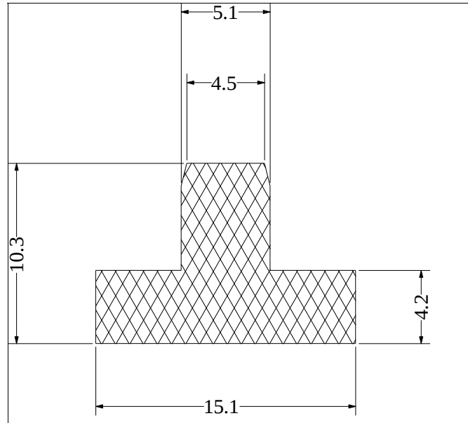
Die No: 1705 Category: T-Section
