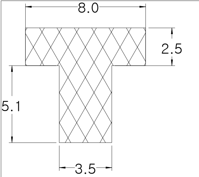
Die No: 8327 Category: T-Section
