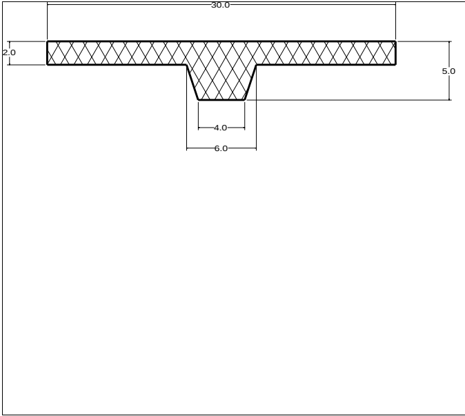
Die No: 5276 Category: T-Section
