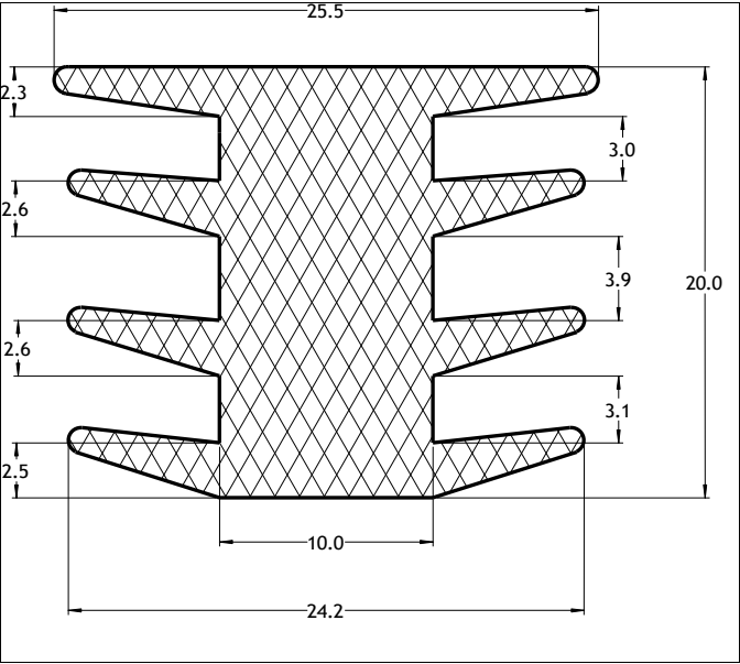
Die No: 7195 Category: T-Section
