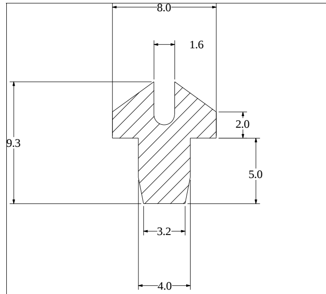
Die No: 1202 Category: T-Section
