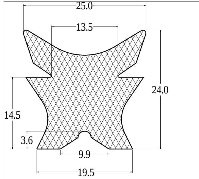
Die No: 9505 Category: T-Section
