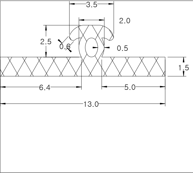
Die No: 8090 Category: T-Section
