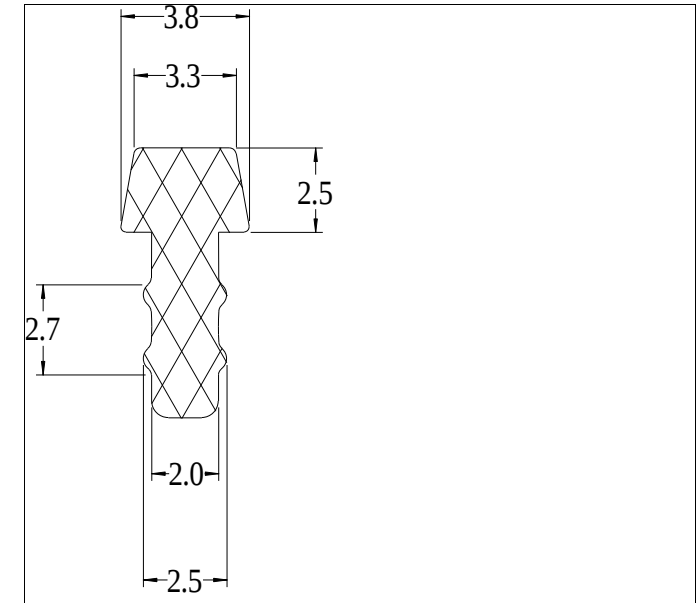
Die No: 9572 Category: T-Section
