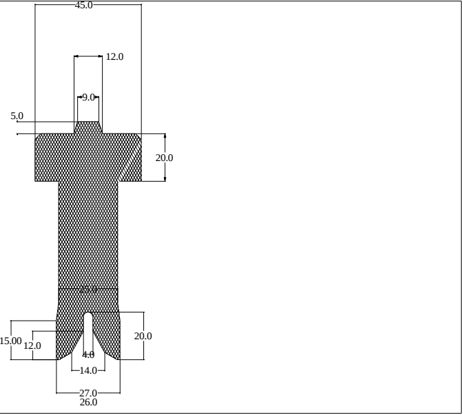
Die No: 3223 Category: T-Section
