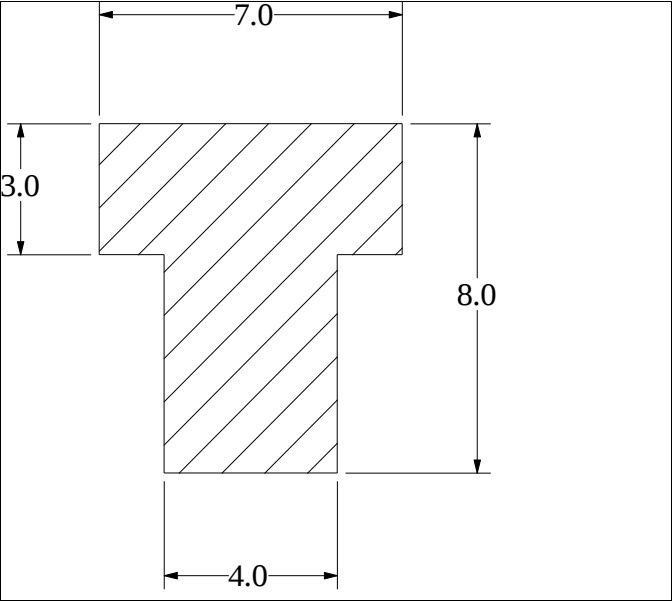
Die No: 1852 Category: T-Section
