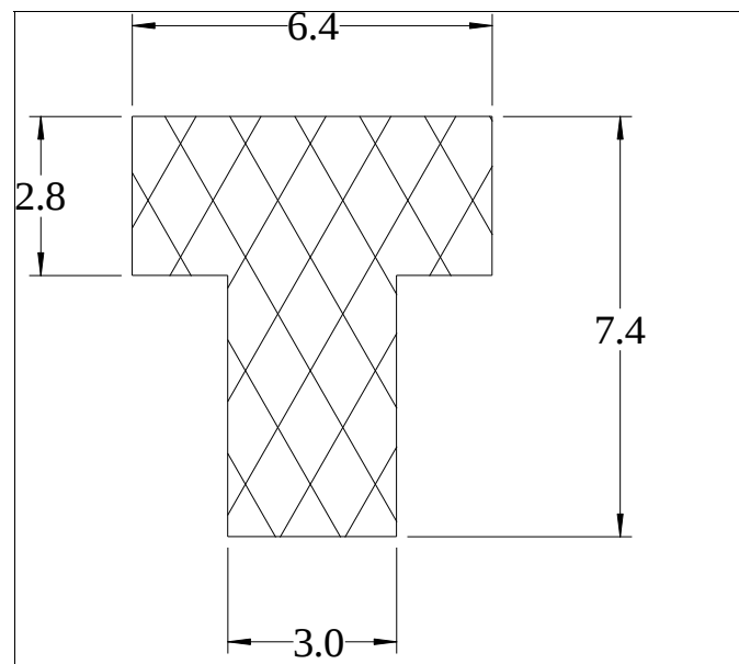
Die No: 5447 Category: T-Section
