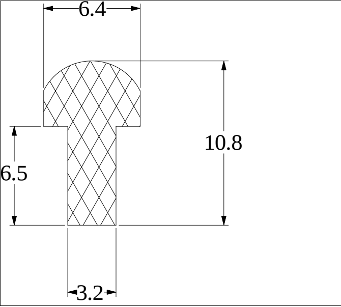
Die No: 2383 Category: T-Section
