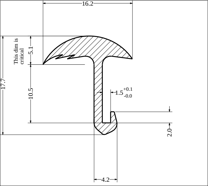
Die No: 1472 Category: T-Section
