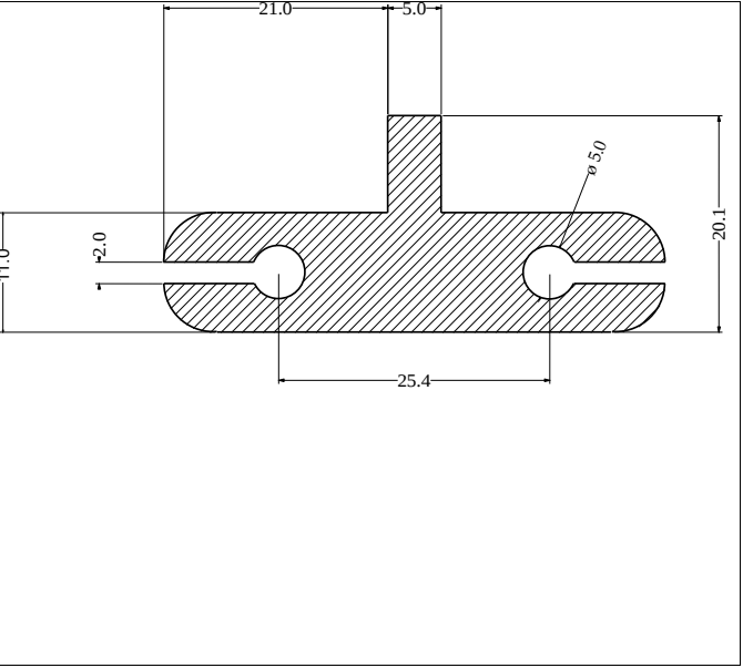
Die No: 576 Category: T-Section
