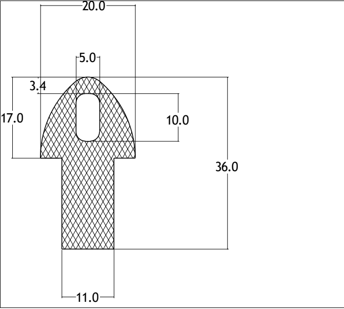
Die No: 6018 Category: T-Section
