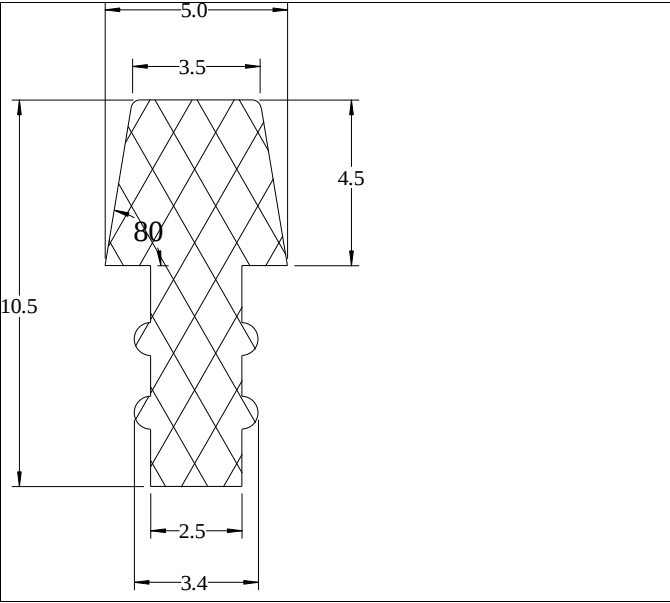
Die No: 5302 Category: T-Section
