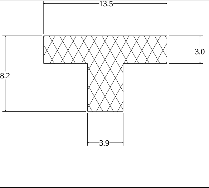
Die No: 3258 Category: T-Section
