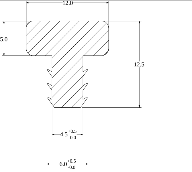
Die No: 2053 Category: T-Section
