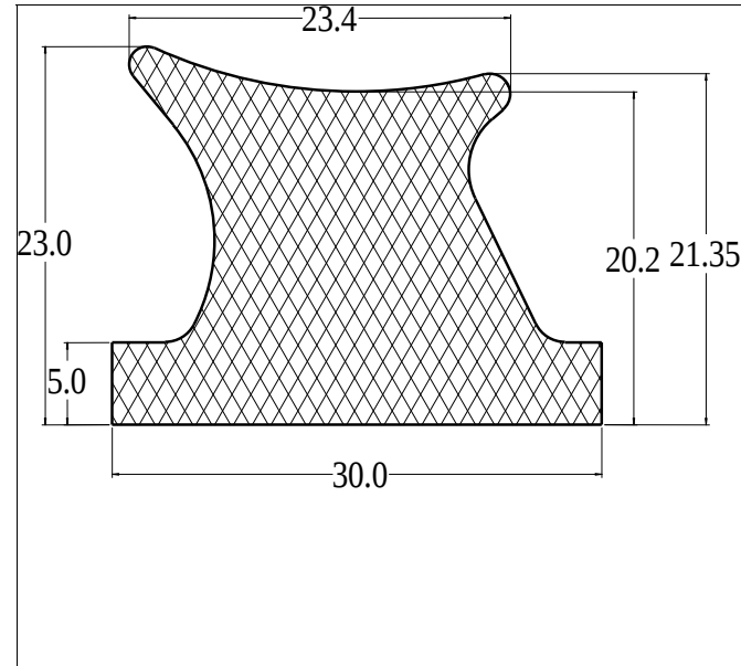
Die No: 9571 Category: T-Section
