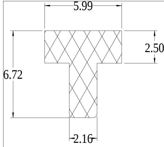
Die No: 9494 Category: T-Section
