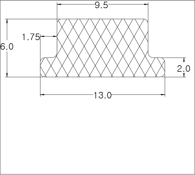
Die No: 8068 Category: T-Section
