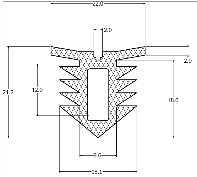
Die No: 2296 Category: T-Section
