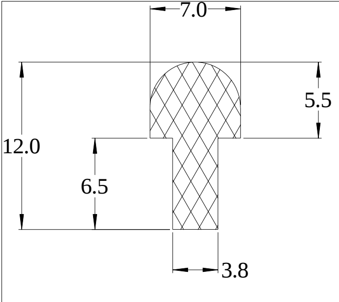
Die No: 6572 Category: T-Section
