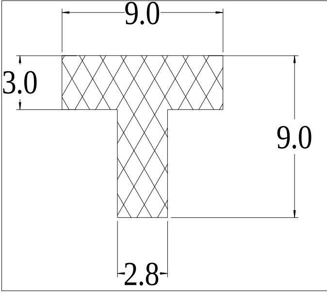
Die No: 9382 Category: T-Section
