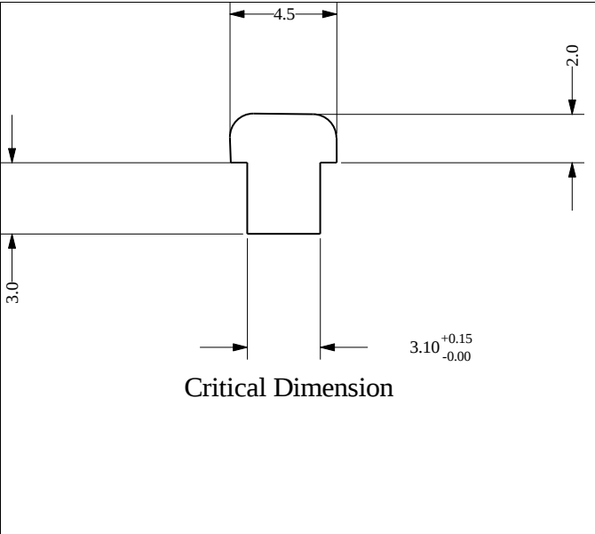
Die No: 619 Category: T-Section
