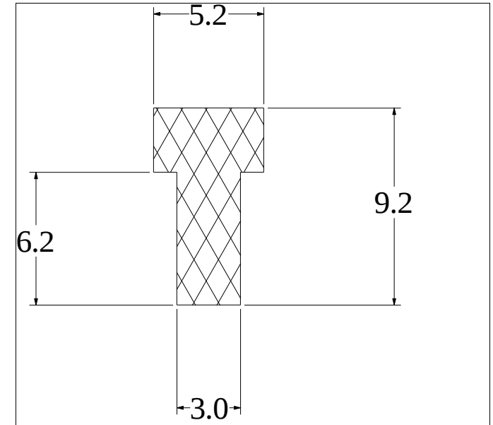
Die No: 3016 Category: T-Section
