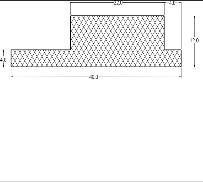
Die No: 9374 Category: T-Section
