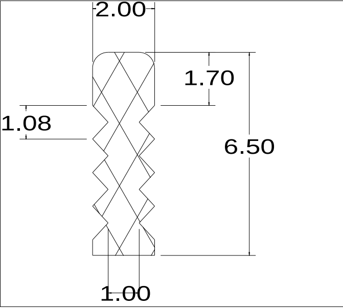
Die No: 3949 Category: T-Section
