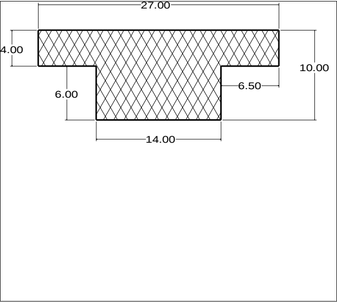
Die No: 5816 Category: T-Section
