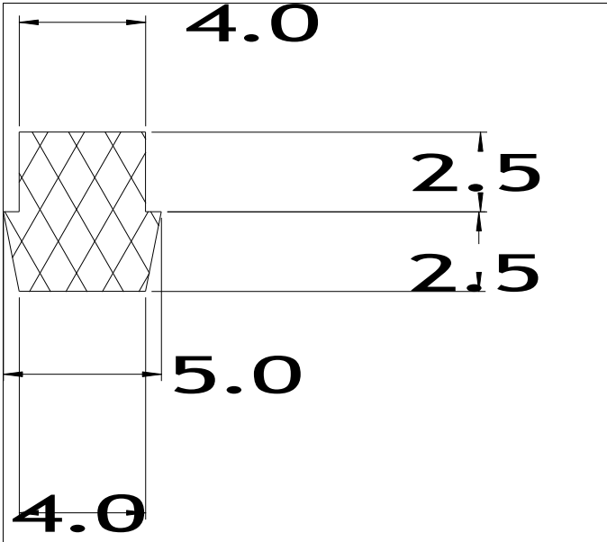
Die No: 7502 Category: T-Section
