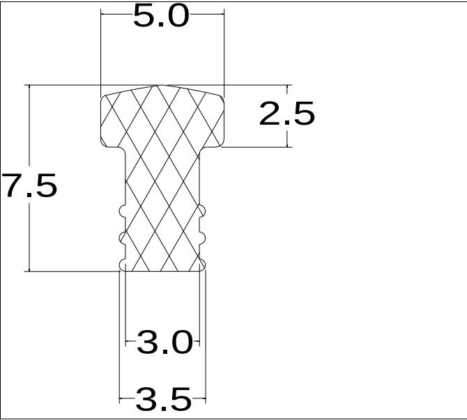
Die No: 4586 Category: T-Section
