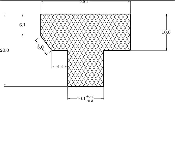
Die No: 7679 Category: T-Section
