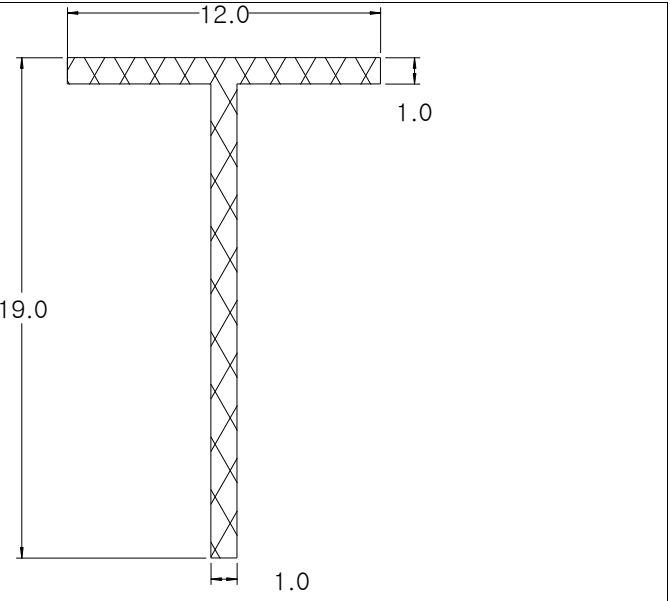
Die No: 8165 Category: T-Section
