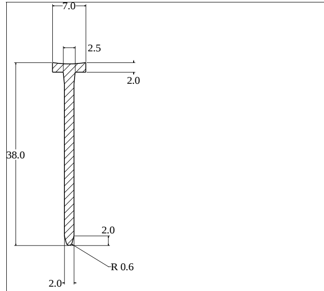
Die No: 2323 Category: T-Section
