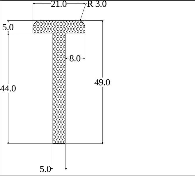
Die No: 3494 Category: T-Section
