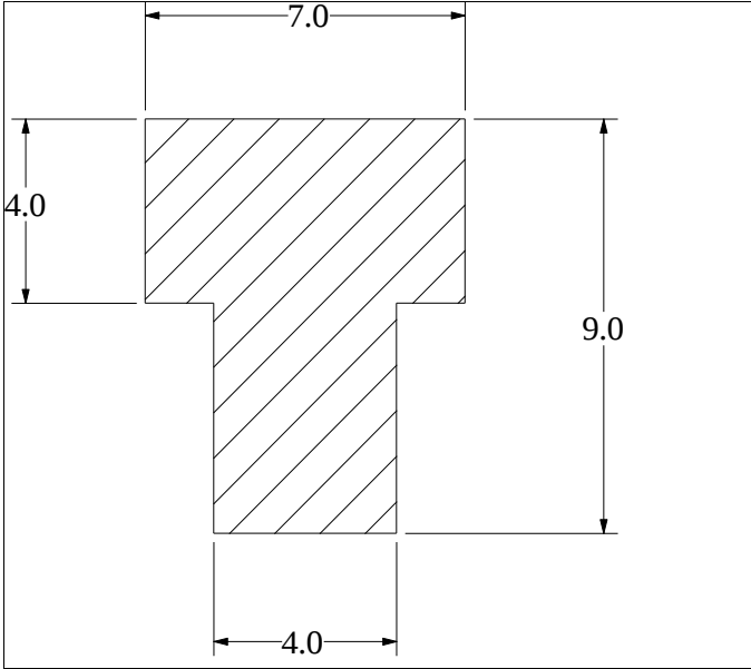
Die No: 1854 Category: T-Section
