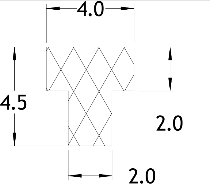
Die No: 6217 Category: T-Section
