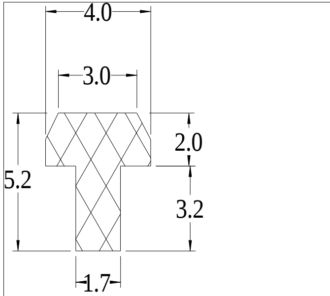
Die No: 9478 Category: T-Section
