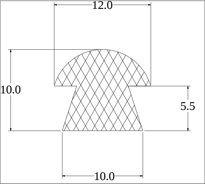
Die No: 2738 Category: T-Section
