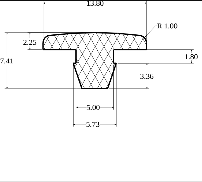
Die No: 3656 Category: T-Section
