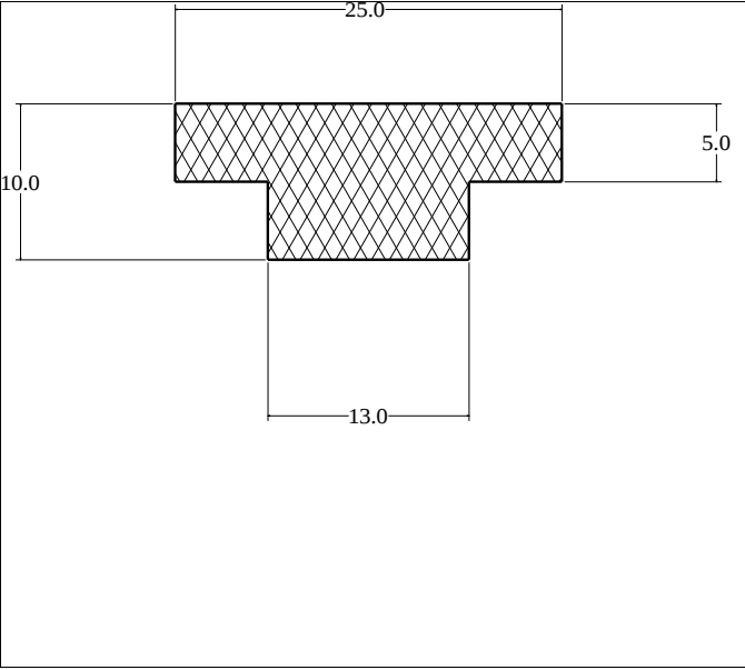
Die No: 3089 Category: T-Section
