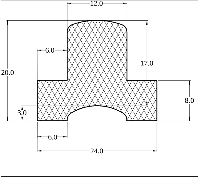
Die No: 5405 Category: T-Section
