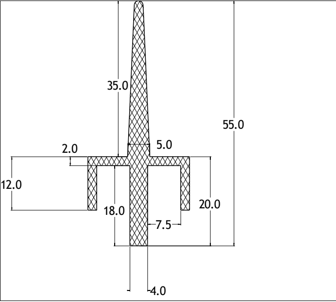
Die No: 7338 Category: T-Section
