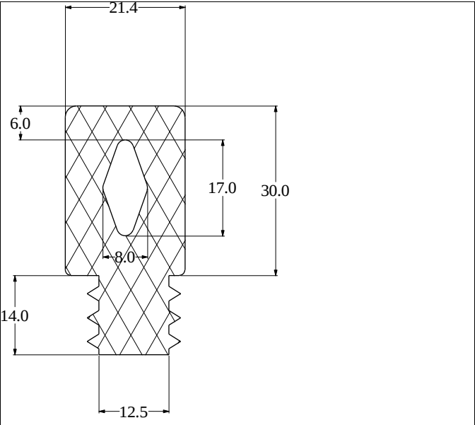
Die No: 2810 Category: T-Section
