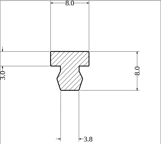
Die No: 305 Category: T-Section
