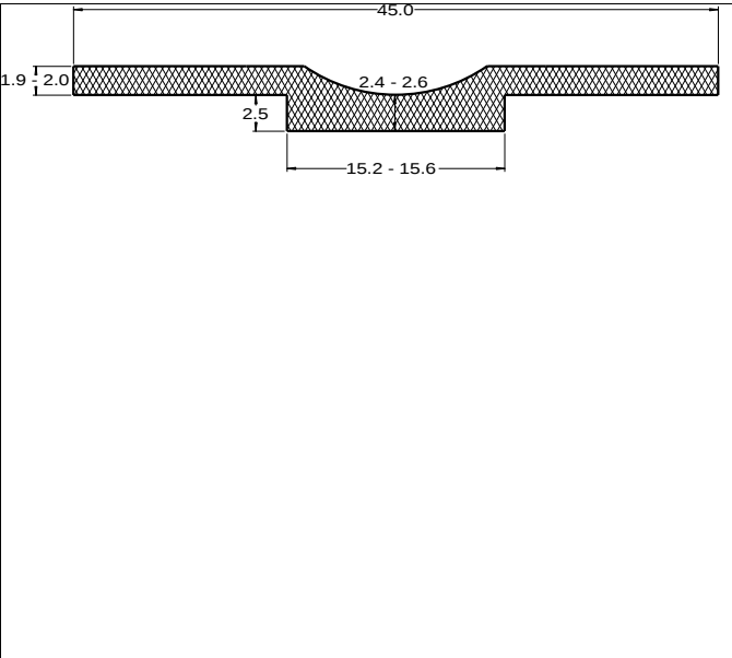
Die No: 7499 Category: T-Section
