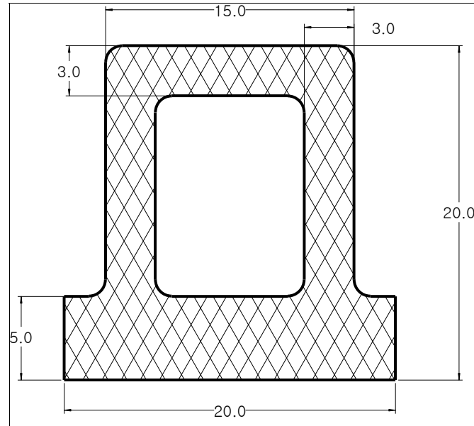
Die No: 8529 Category: T-Section
