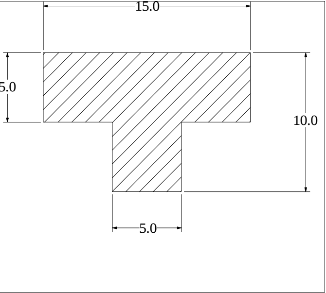
Die No: 1936 Category: T-Section
