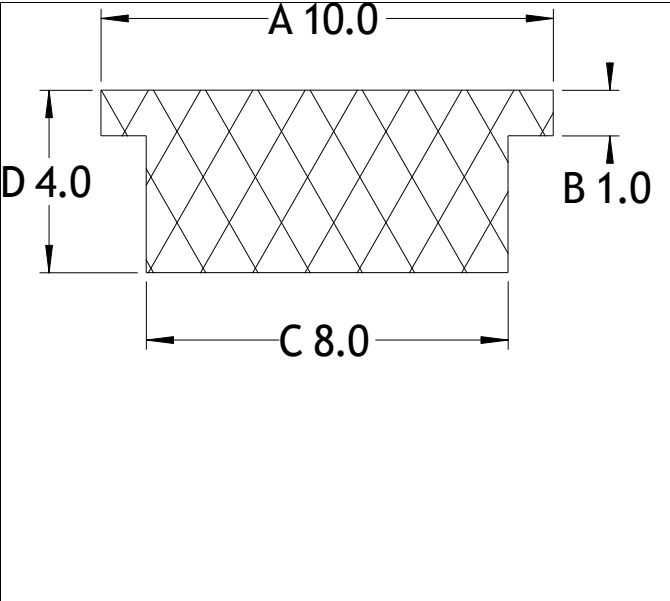
Die No: 6947 Category: T-Section
