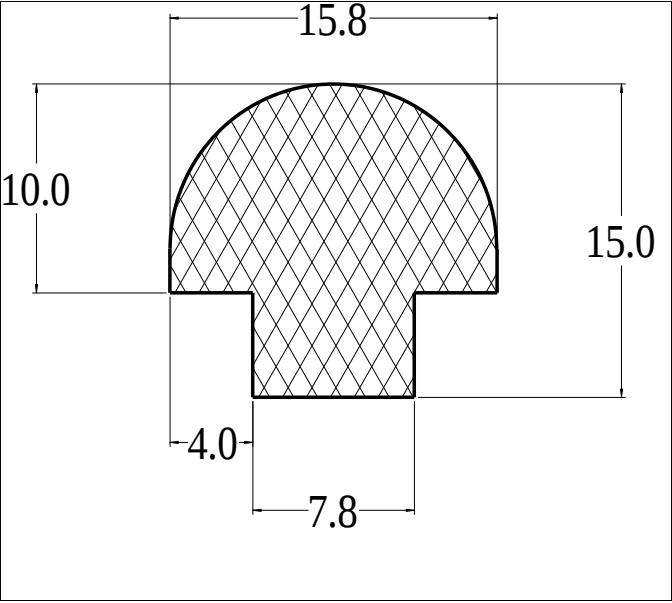
Die No: 6680 Category: T-Section
