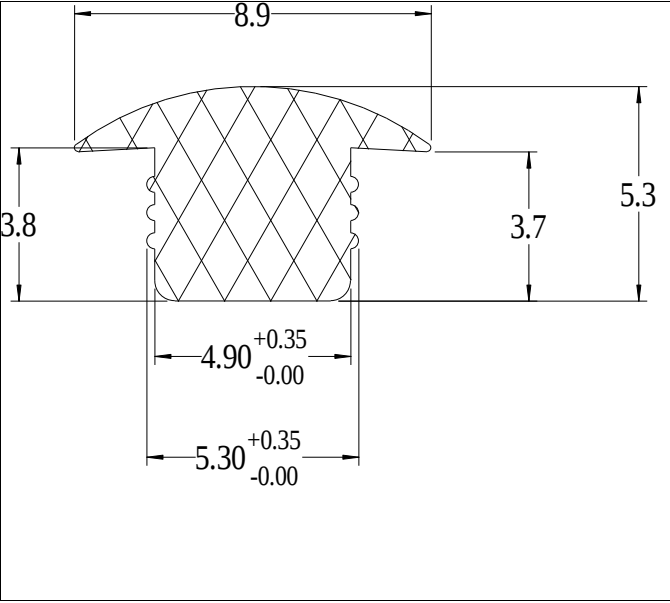
Die No: 9160 Category: T-Section
