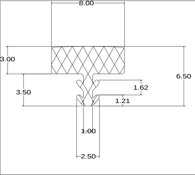
Die No: 4503 Category: T-Section
