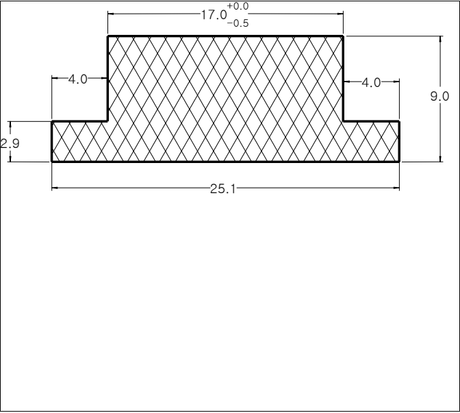
Die No: 7955 Category: T-Section
