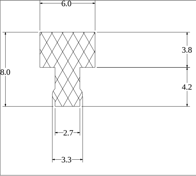
Die No: 3379 Category: T-Section
