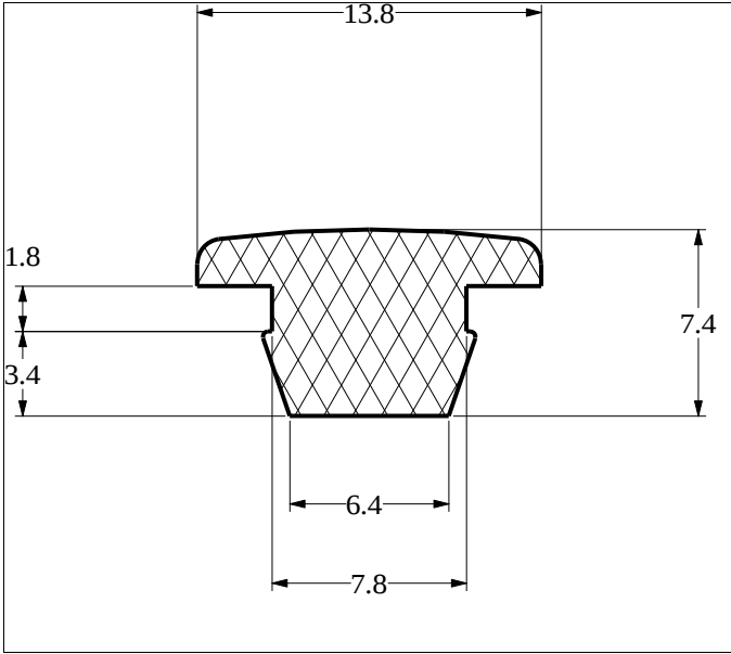
Die No: 3517 Category: T-Section
