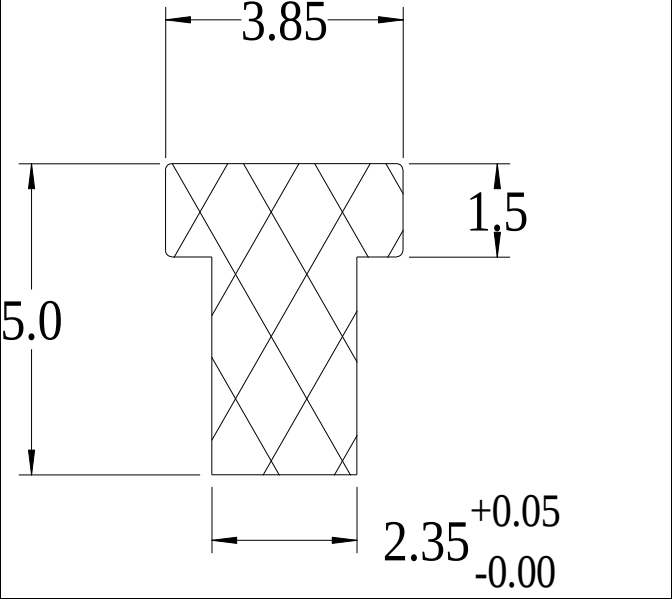
Die No: 9763 Category: T-Section
