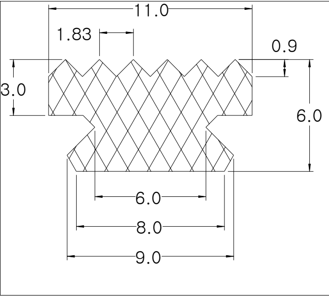
Die No: 8653 Category: T-Section
