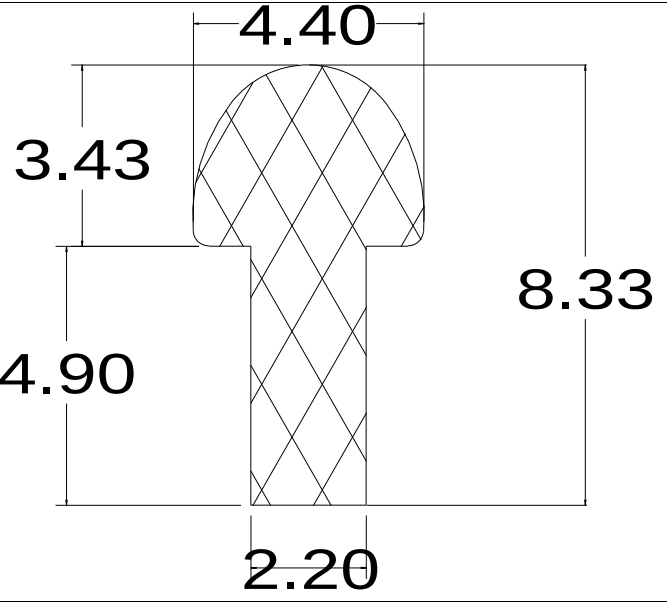
Die No: 4119 Category: T-Section
