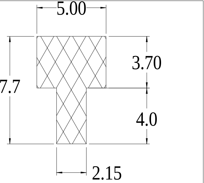
Die No: 9819 Category: T-Section
