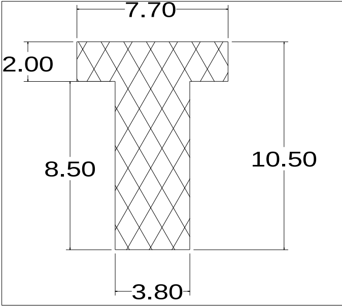
Die No: 5748 Category: T-Section
