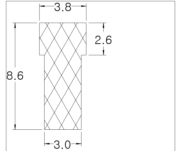
Die No: 8530 Category: T-Section
