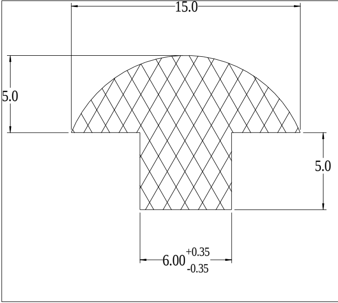
Die No: 9284 Category: T-Section
