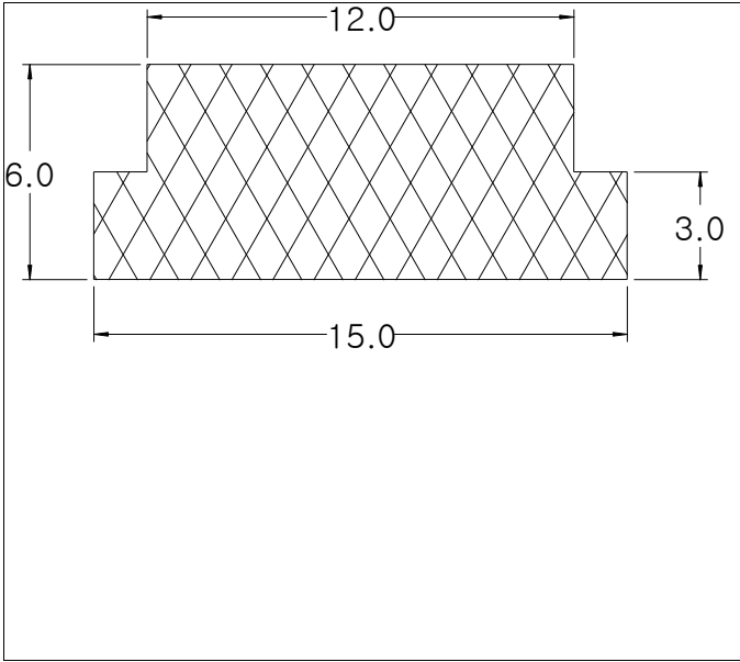
Die No: 8662 Category: T-Section
