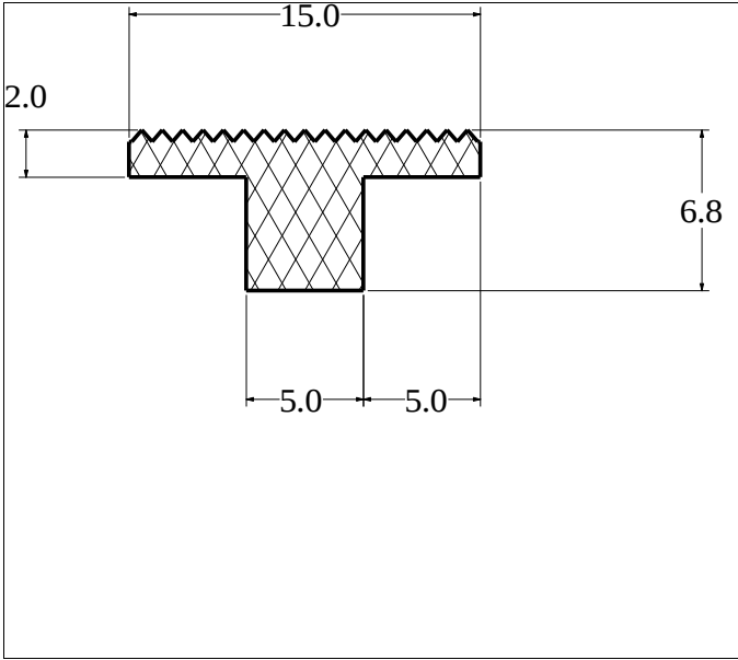
Die No: 2681 Category: T-Section
