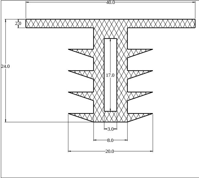
Die No: 5134 Category: T-Section
