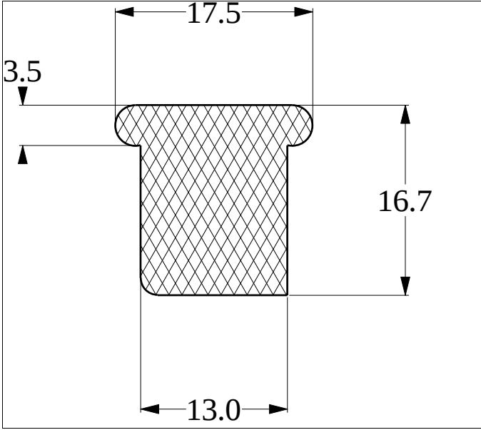
Die No: 3276 Category: T-Section
