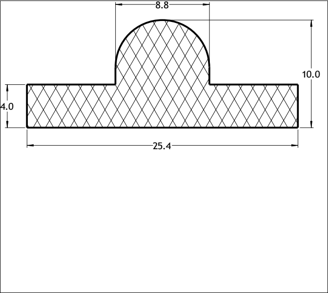
Die No: 6735 Category: T-Section
