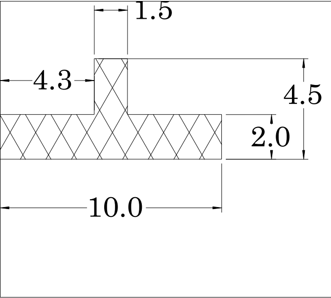
Die No: 7764 Category: T-Section
