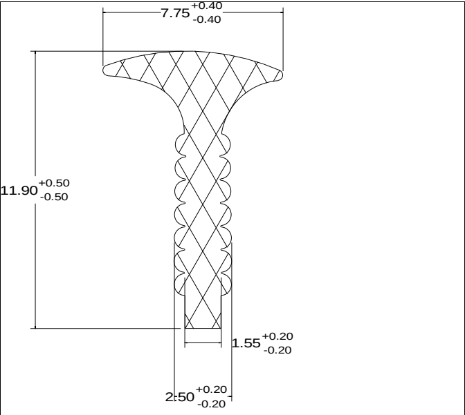
Die No: 7829 Category: T-Section
