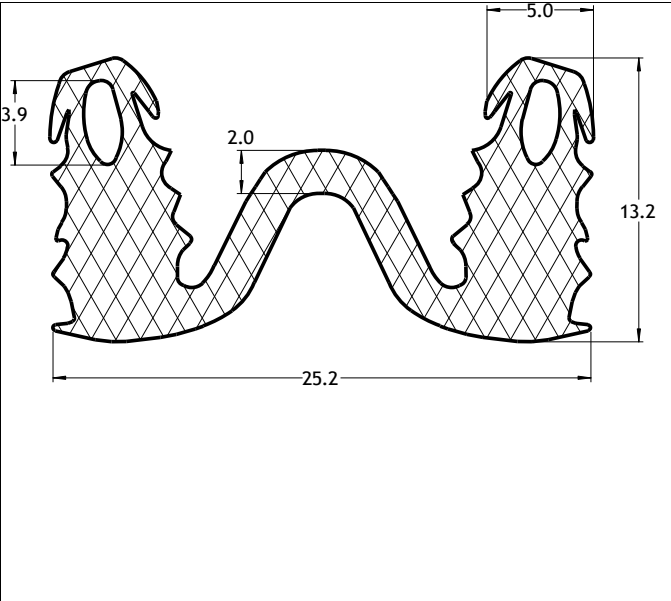
Die No: 6253 Category: T-Section
