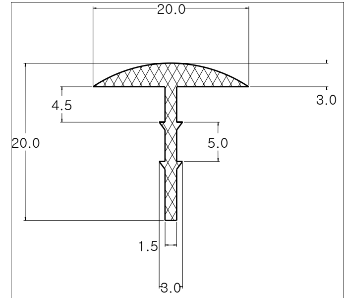
Die No: 8880 Category: T-Section
