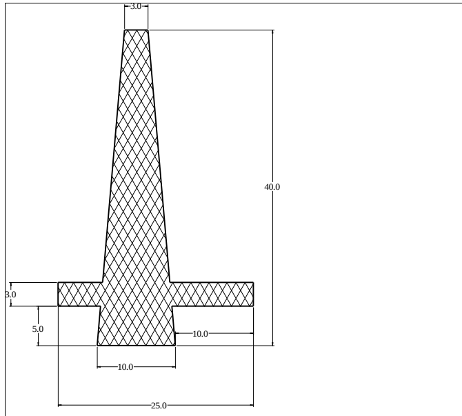
Die No: 5503 Category: T-Section
