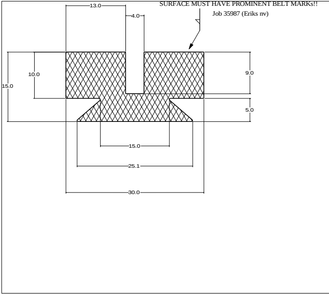
Die No: 4789 Category: T-Section
