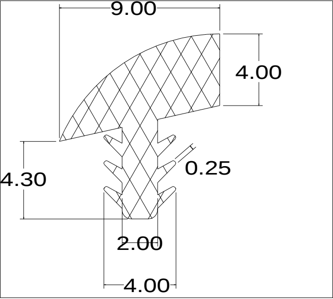
Die No: 7903 Category: T-Section
