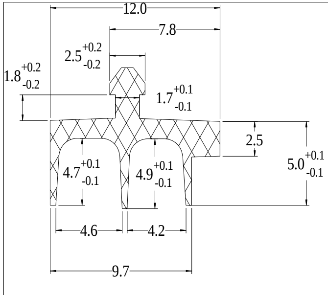
Die No: 9570 Category: T-Section
