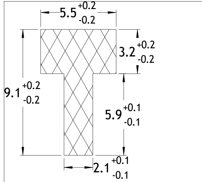
Die No: 7051 Category: T-Section
