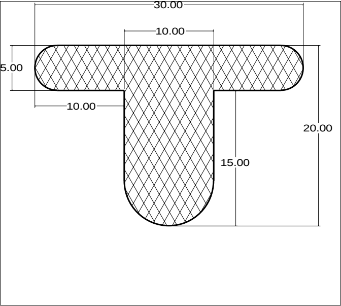
Die No: 5958 Category: T-Section
