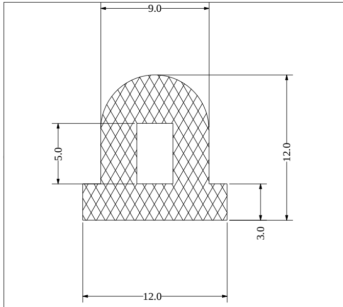
Die No: 784 Category: T-Section
