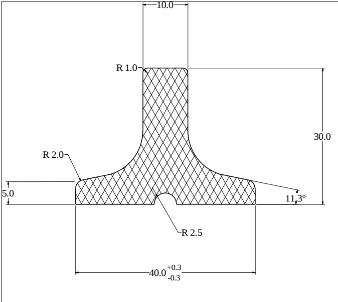
Die No: 3842 Category: T-Section
