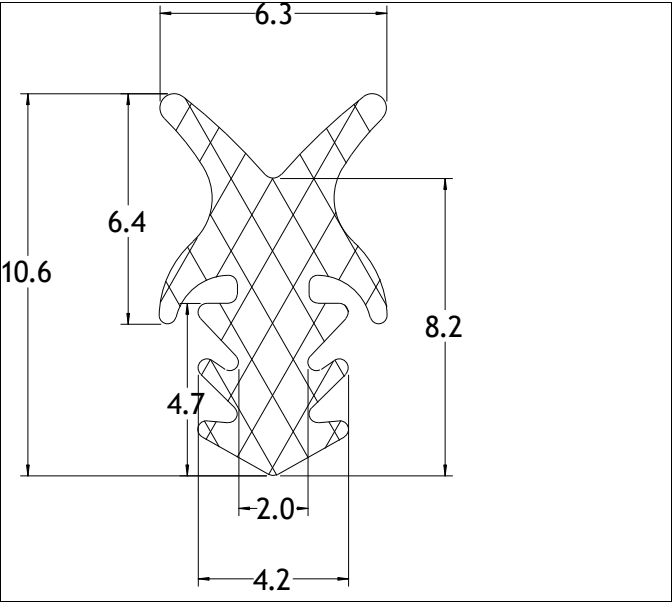
Die No: 7310 Category: T-Section
