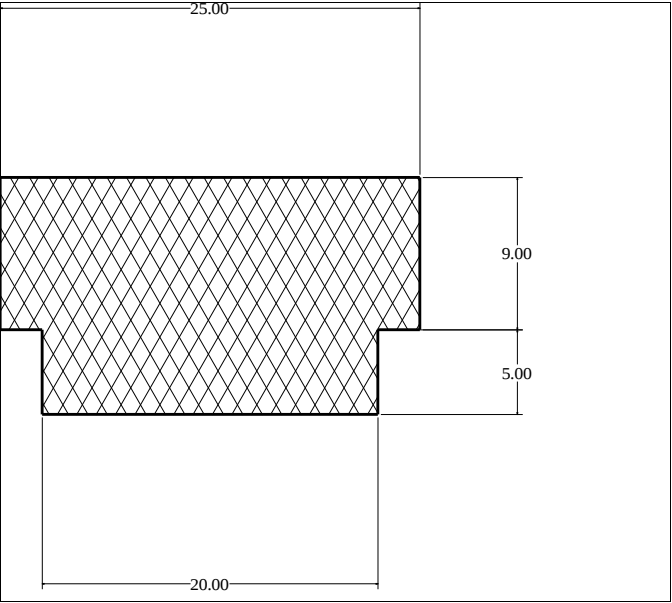
Die No: 3220 Category: T-Section
