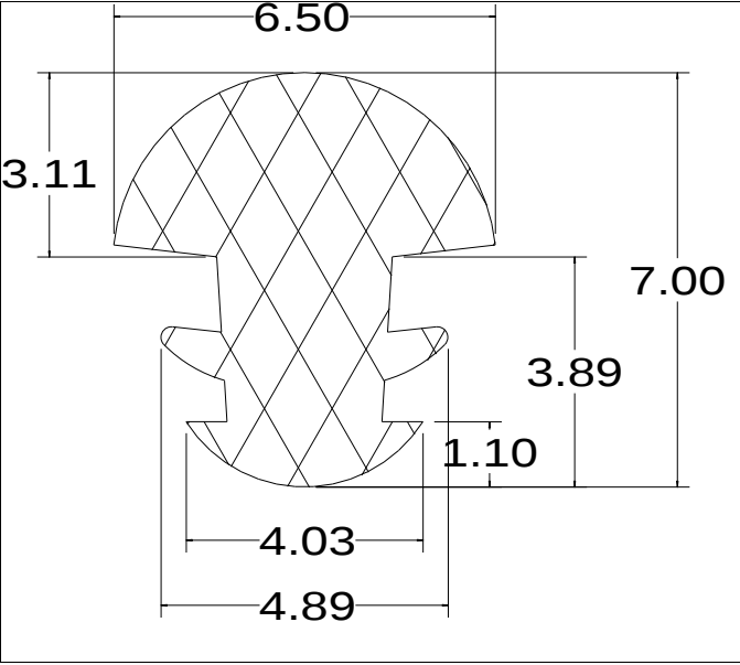
Die No: 4139 Category: T-Section
