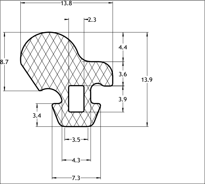
Die No: 7153 Category: T-Section
