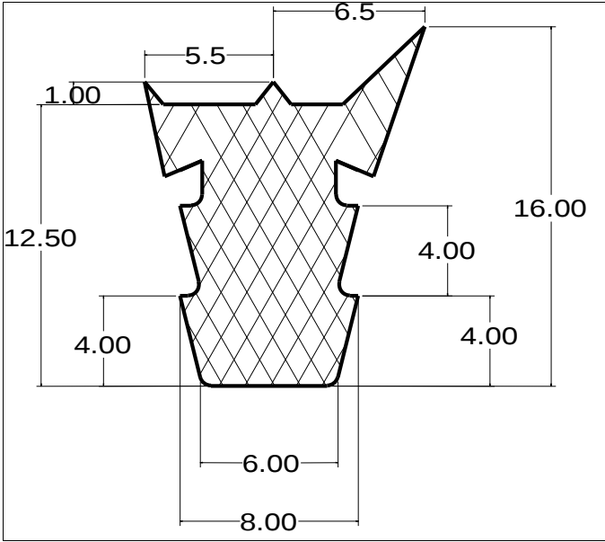
Die No: 4038 Category: T-Section
