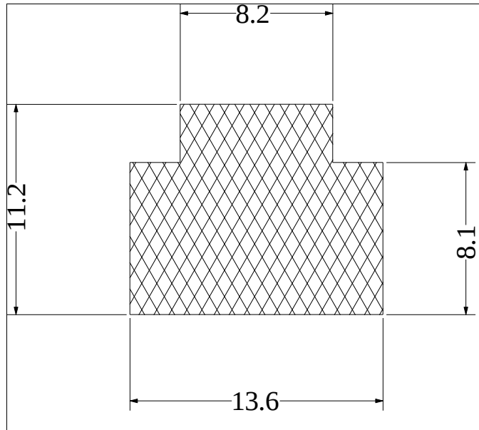
Die No: 1200 Category: T-Section
