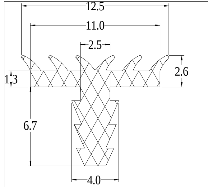
Die No: 9635 Category: T-Section
