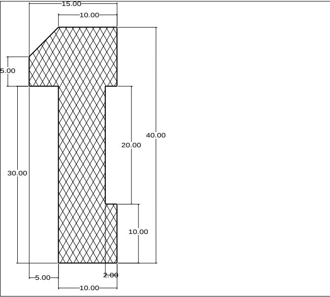
Die No: 4037 Category: T-Section
