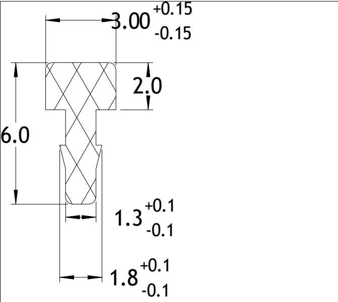
Die No: 6759 Category: T-Section
