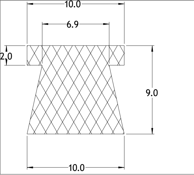
Die No: 7335 Category: T-Section
