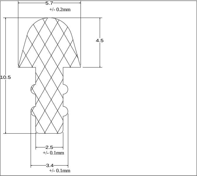
Die No: 5266 Category: T-Section
