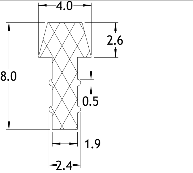
Die No: 6948 Category: T-Section
