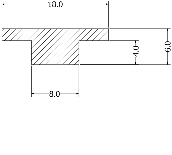
Die No: 407 Category: T-Section
