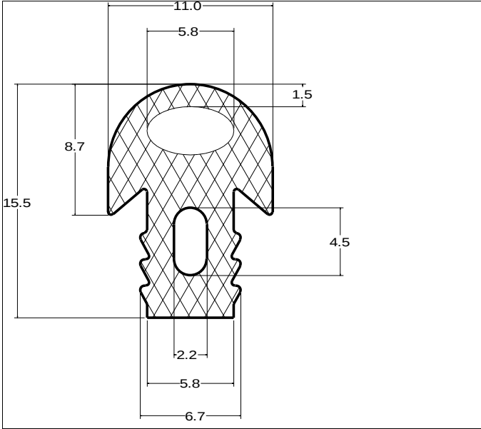
Die No: 4720 Category: T-Section
