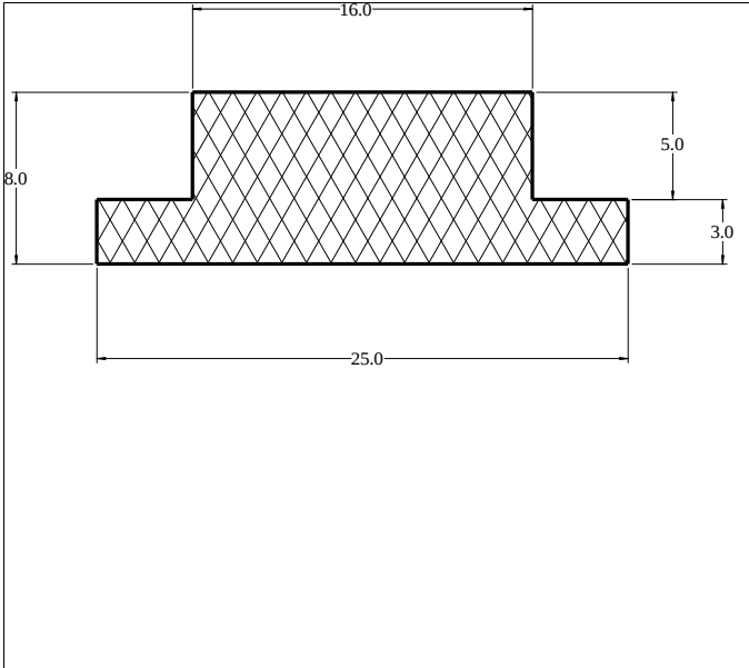
Die No: 4958 Category: T-Section
