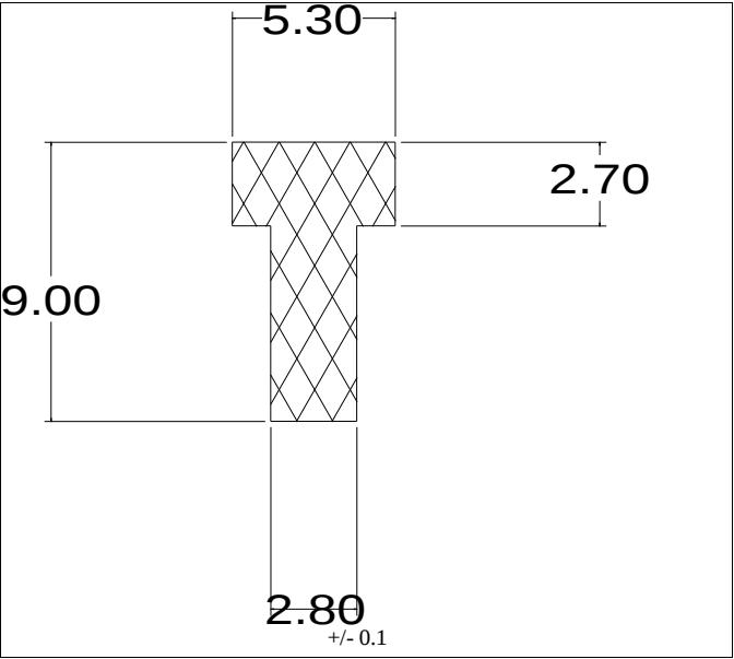
Die No: 4266 Category: T-Section
