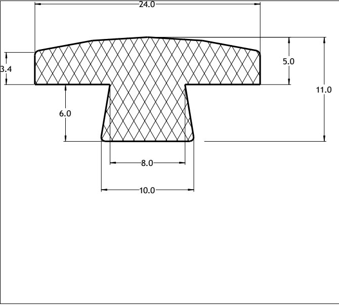
Die No: 7203 Category: T-Section
