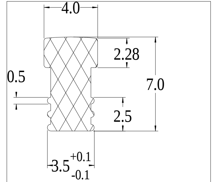
Die No: 9018 Category: T-Section
