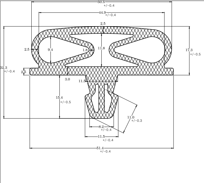
Die No: 7701 Category: T-Section
