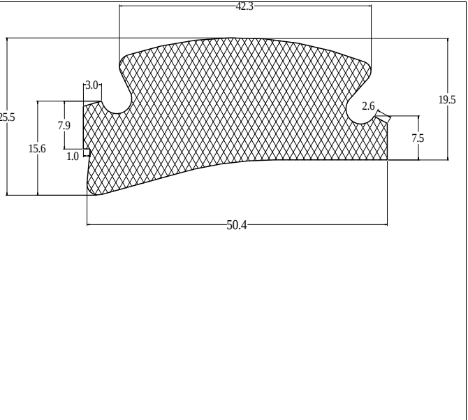
Die No: 9452 Category: T-Section
