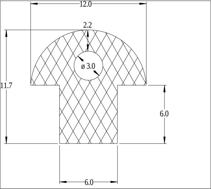
Die No: 9368 Category: T-Section
