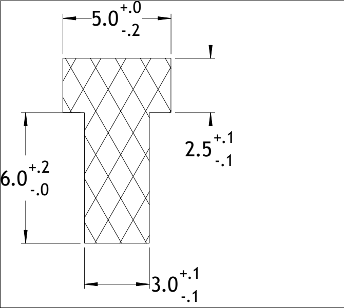
Die No: 7156 Category: T-Section
