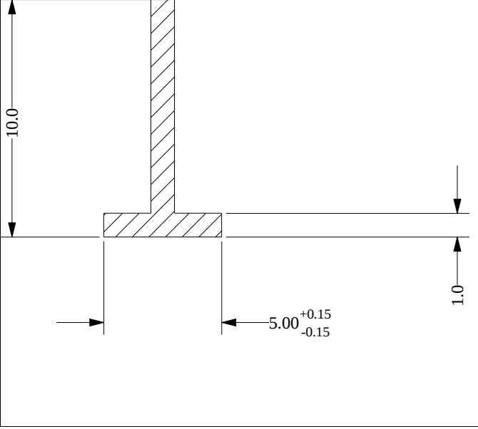
Die No: 1353 Category: T-Section
