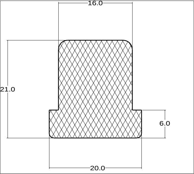
Die No: 5301 Category: T-Section
