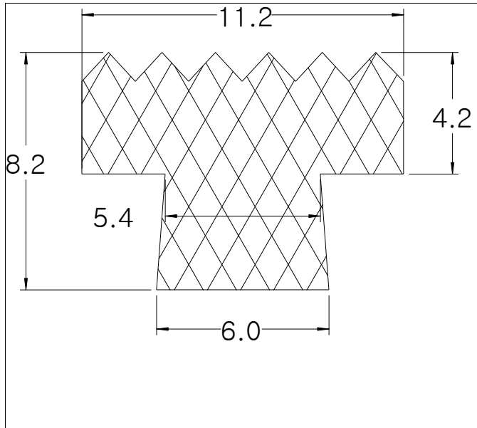
Die No: 8497 Category: T-Section
