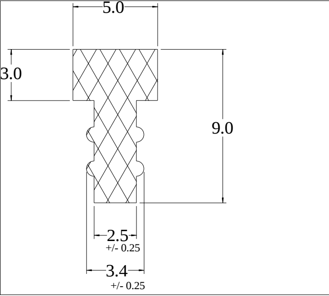
Die No: 5401 Category: T-Section
