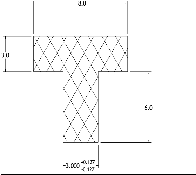
Die No: 6868 Category: T-Section
