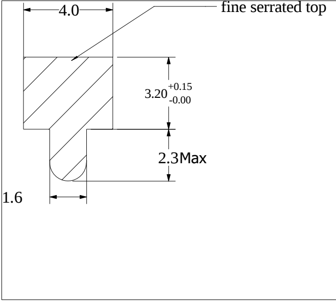
Die No: 2014 Category: T-Section
