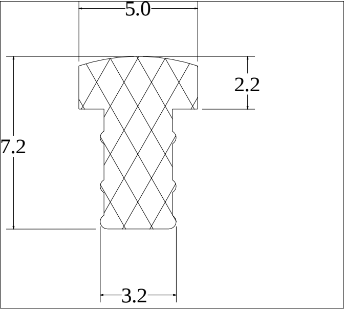
Die No: 3241 Category: T-Section
