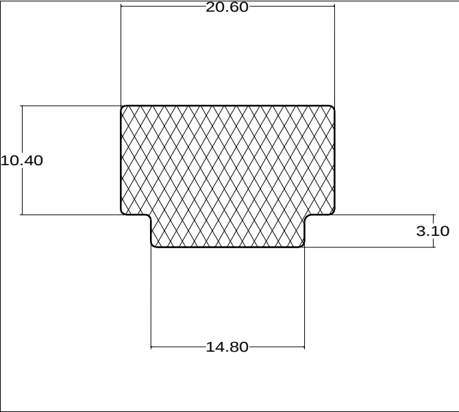
Die No: 4332 Category: T-Section
