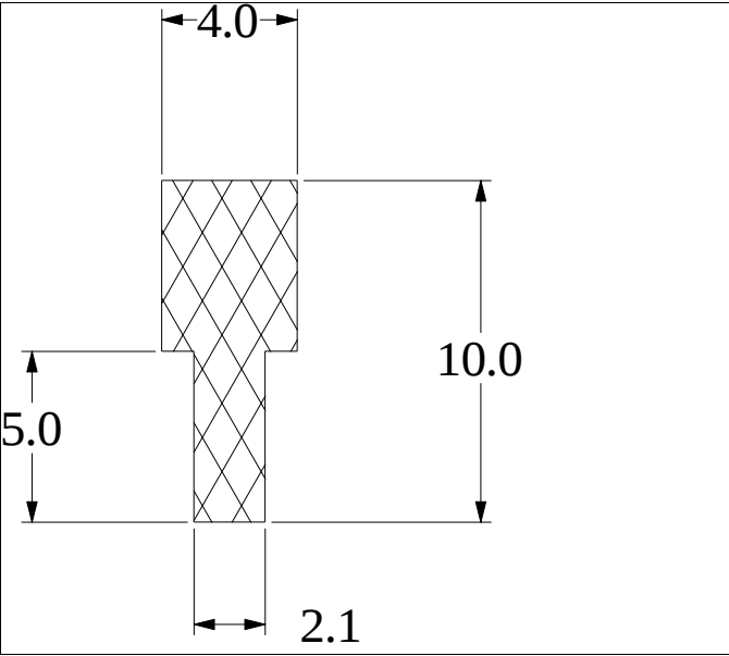
Die No: 3364 Category: T-Section
