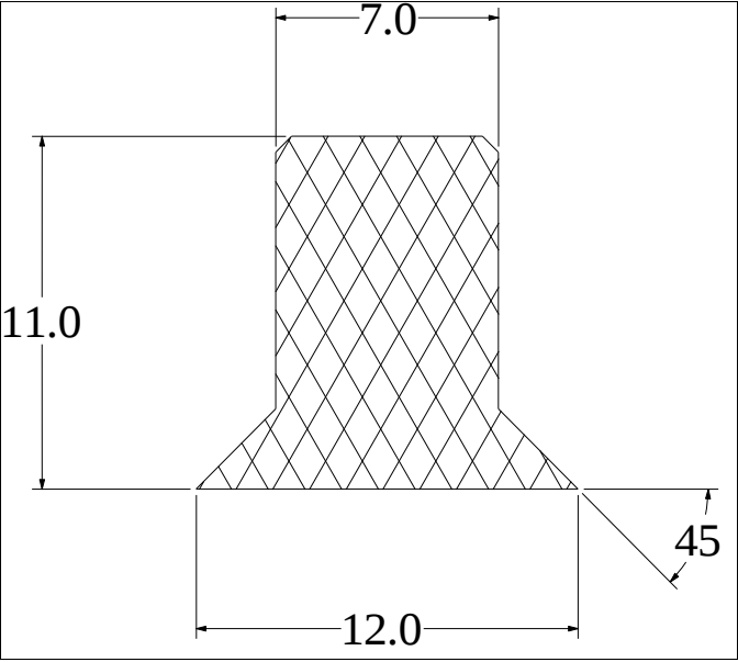
Die No: 3056 Category: T-Section
