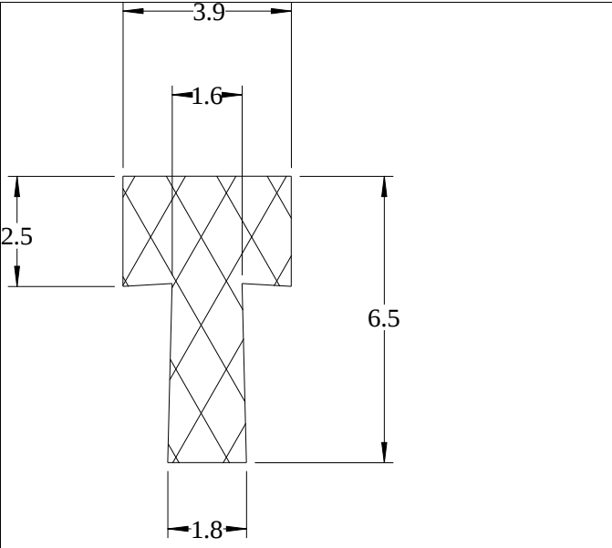
Die No: 4904 Category: T-Section
