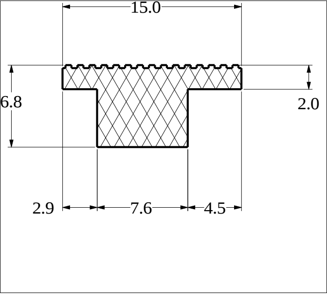
Die No: 2376 Category: T-Section
