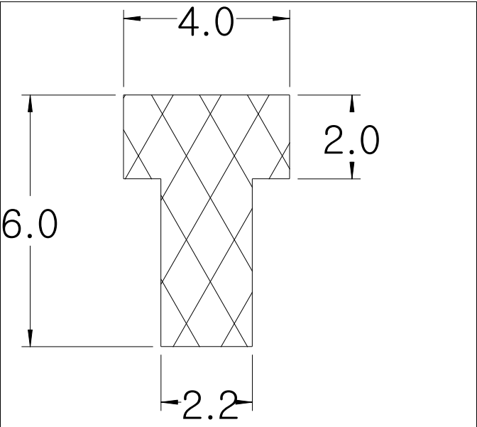
Die No: 8299 Category: T-Section
