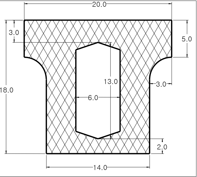
Die No: 8459 Category: T-Section
