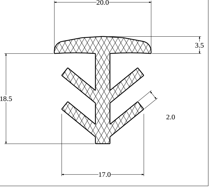
Die No: 2776 Category: T-Section
