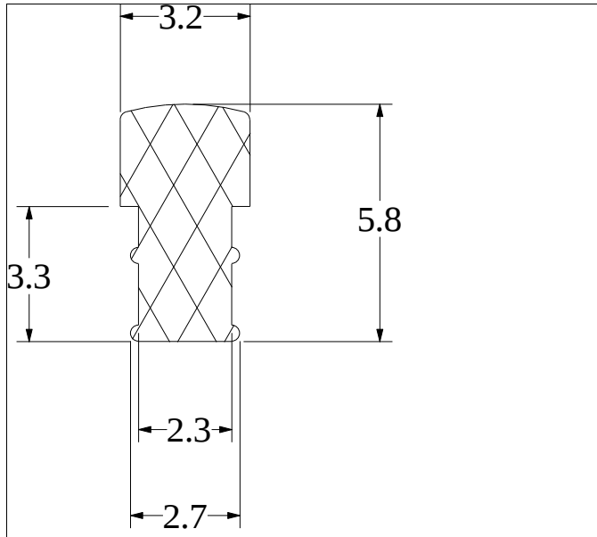
Die No: 3011 Category: T-Section
