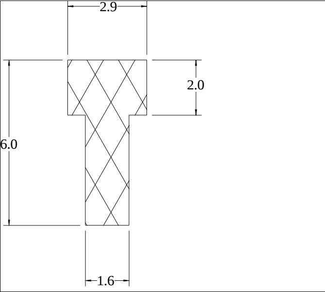
Die No: 4901 Category: T-Section
