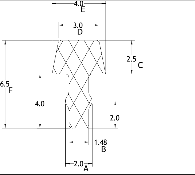
Die No: 6865 Category: T-Section
