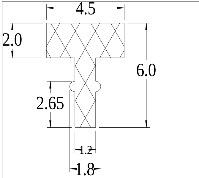
Die No: 9502 Category: T-Section
