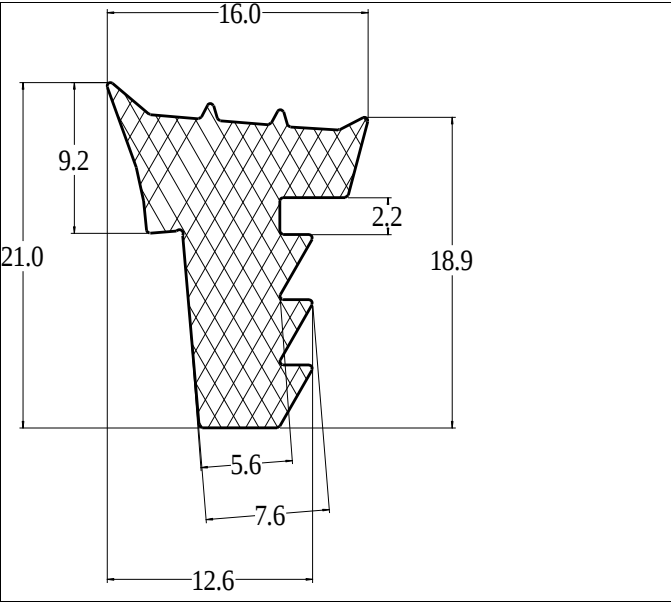
Die No: 9782 Category: T-Section
