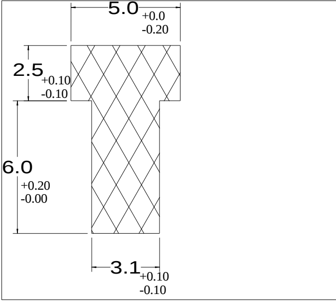
Die No: 7916 Category: T-Section
