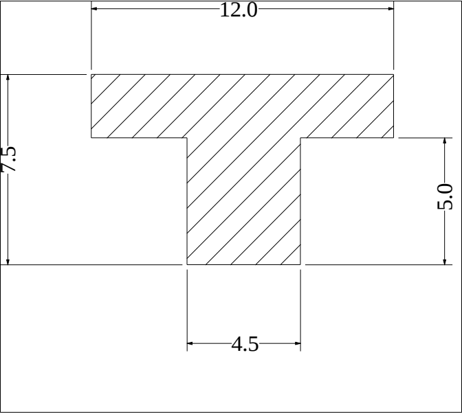
Die No: 567 Category: T-Section
