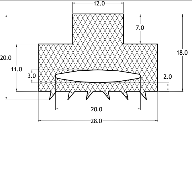
Die No: 6757 Category: T-Section
