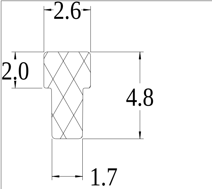
Die No: 9895 Category: T-Section
