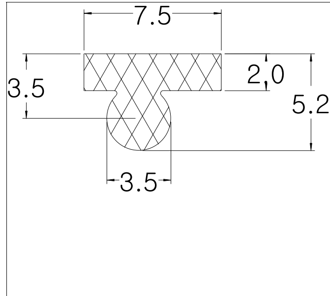
Die No: 8913 Category: T-Section
