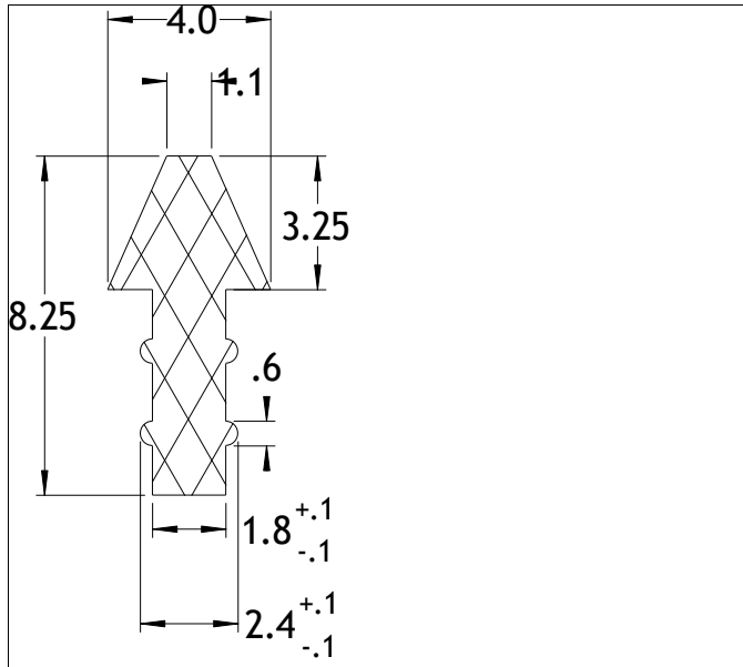
Die No: 6435 Category: T-Section
