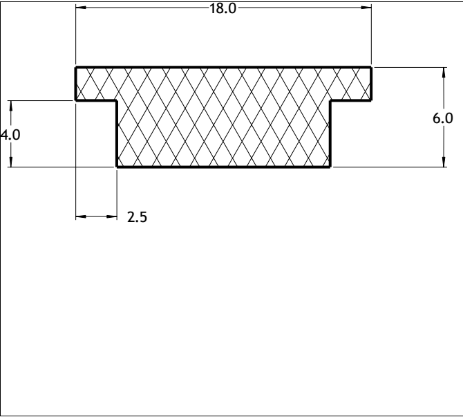
Die No: 6840 Category: T-Section
