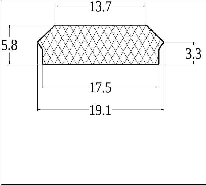
Die No: 9168 Category: T-Section
