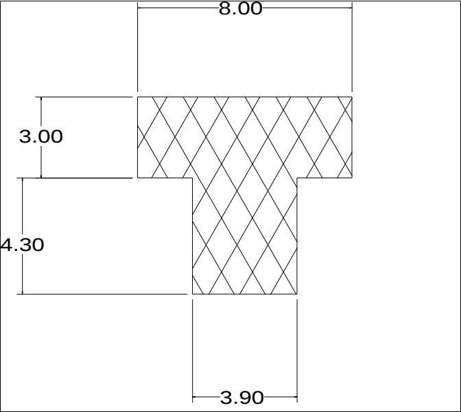
Die No: 4324 Category: T-Section
