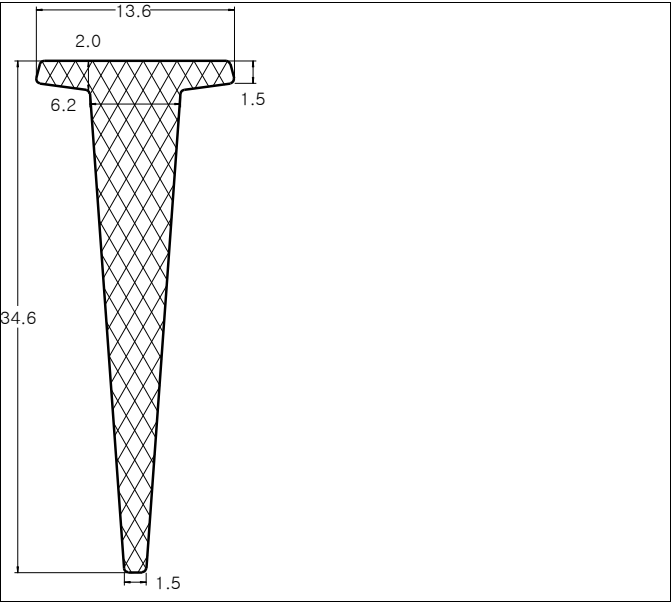
Die No: 7981 Category: T-Section
