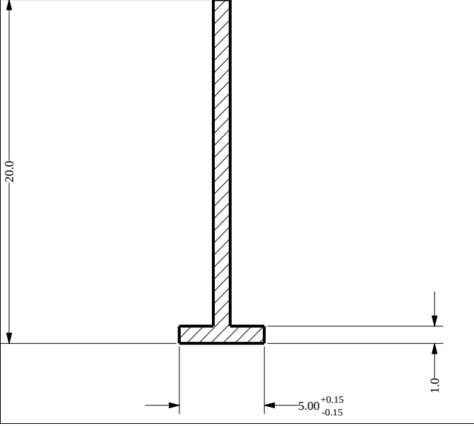
Die No: 1354 Category: T-Section
