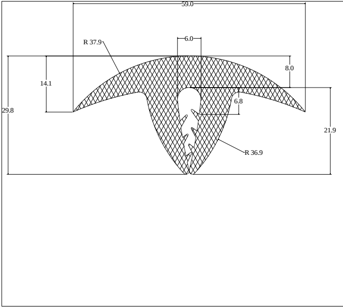
Die No: 3659 Category: T-Section
