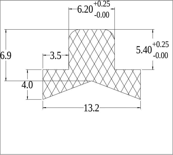
Die No: 9405 Category: T-Section
