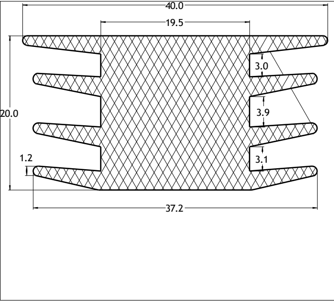
Die No: 7266 Category: T-Section
