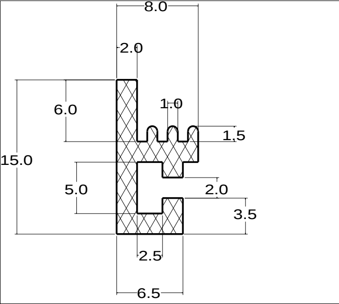
Die No: 4716 Category: T-Section
