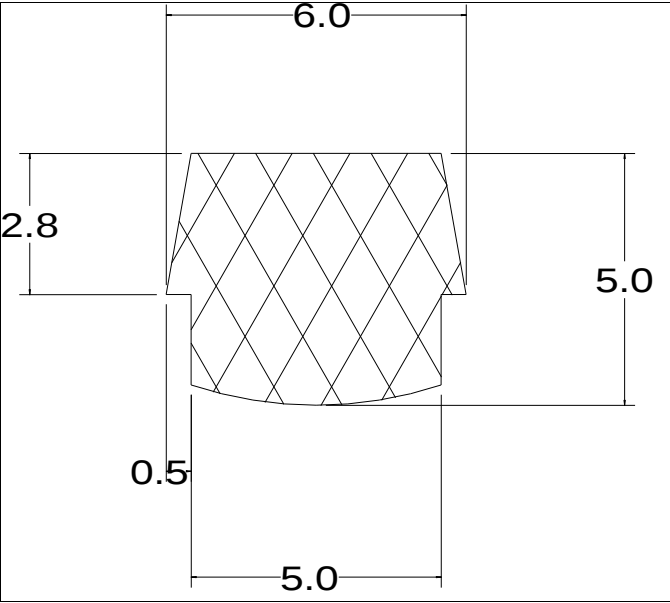
Die No: 4788 Category: T-Section
