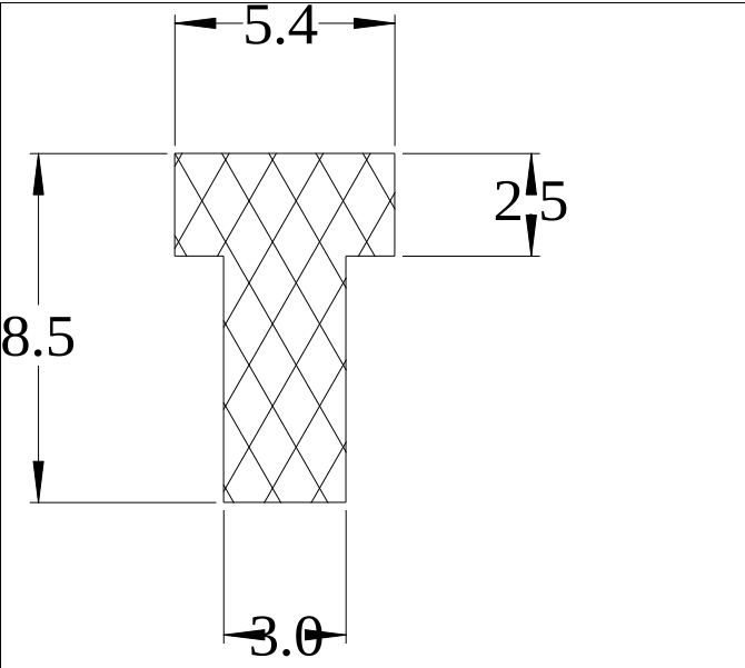
Die No: 4954 Category: T-Section
