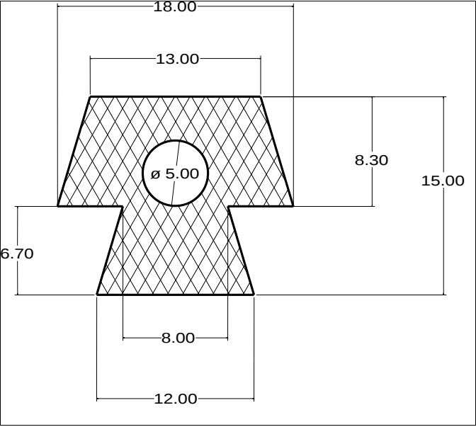
Die No: 5701 Category: T-Section
