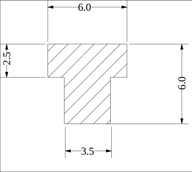
Die No: 1509 Category: T-Section
