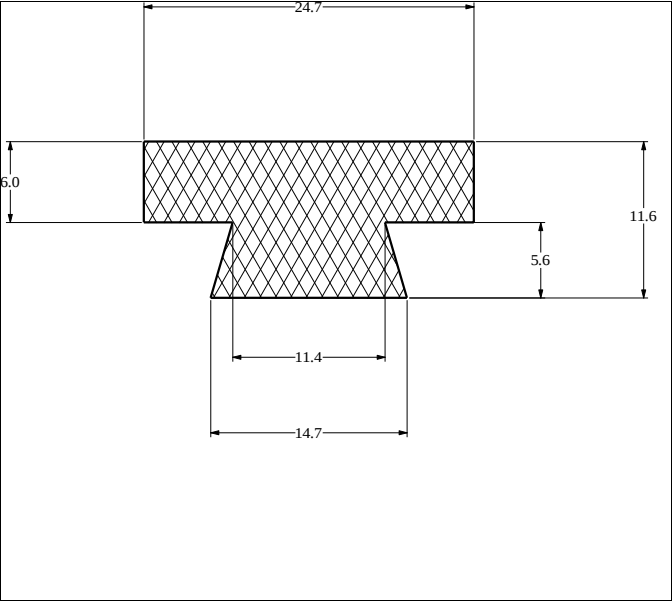
Die No: 3458 Category: T-Section
