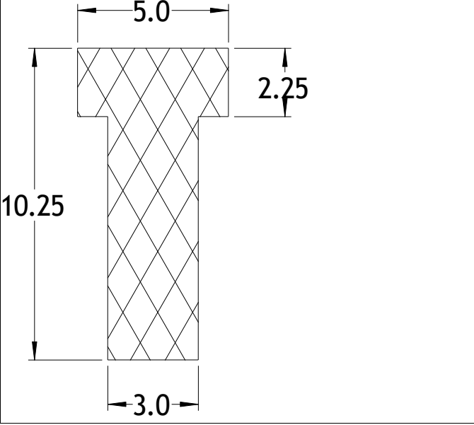
Die No: 7371 Category: T-Section
