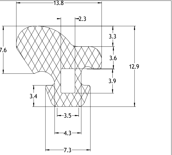
Die No: 7158 Category: T-Section
