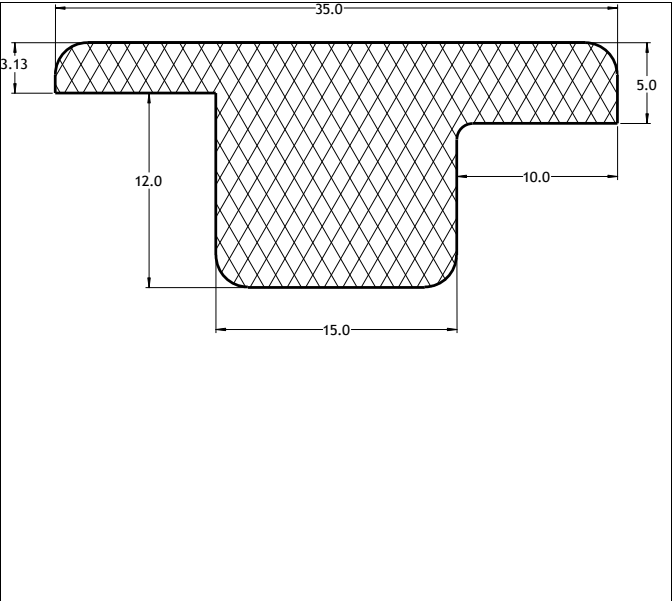
Die No: 7493 Category: T-Section
