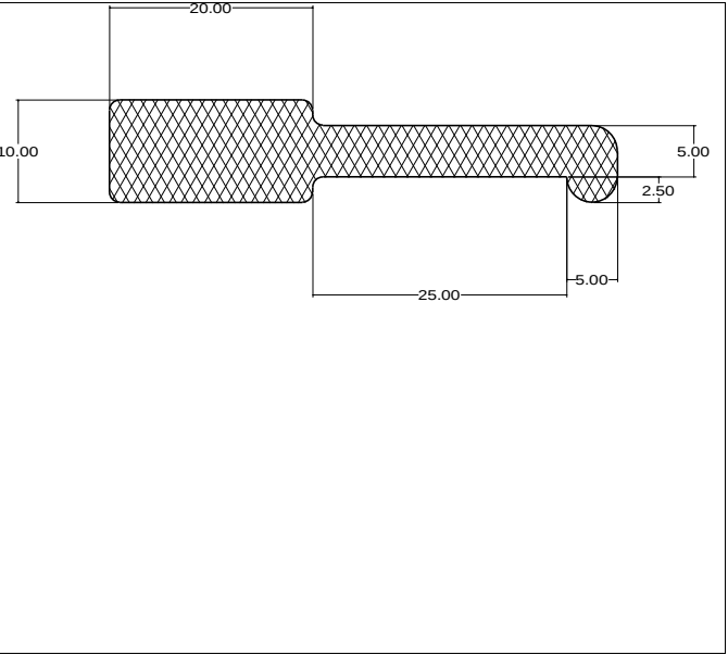
Die No: 4544 Category: T-Section
