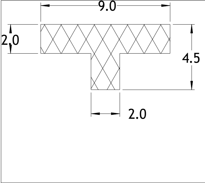
Die No: 6132 Category: T-Section
