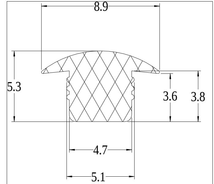
Die No: 9099 Category: T-Section
