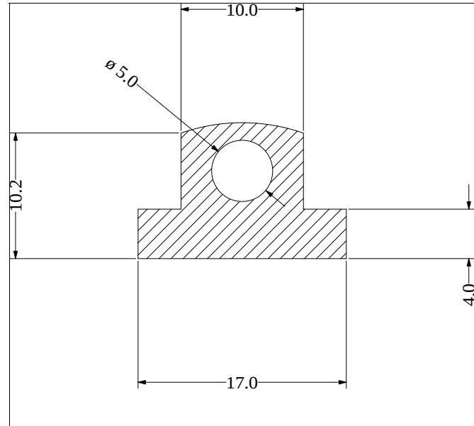
Die No: 856 Category: T-Section
