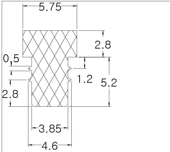
Die No: 8862 Category: T-Section
