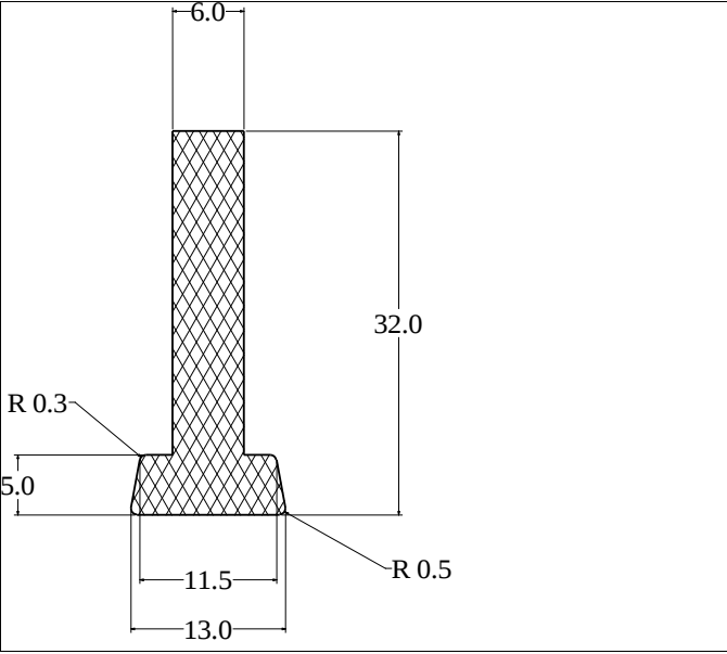
Die No: 2992 Category: T-Section
