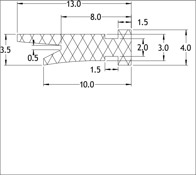
Die No: 6940 Category: T-Section
