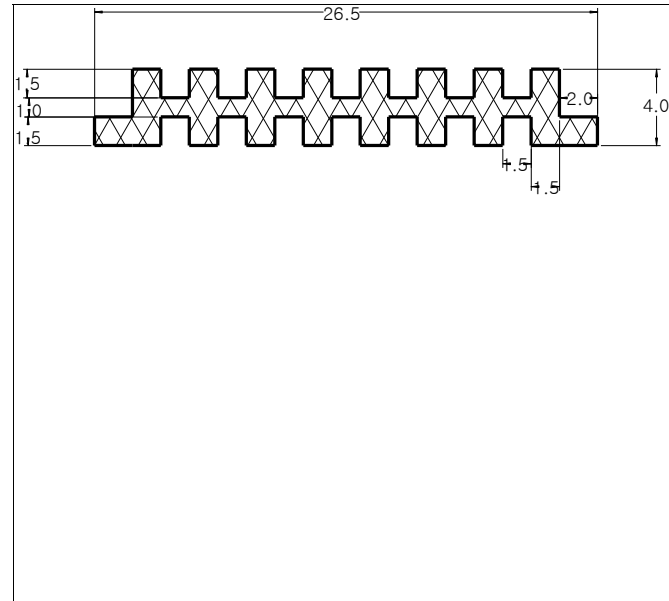
Die No: 7622 Category: T-Section
