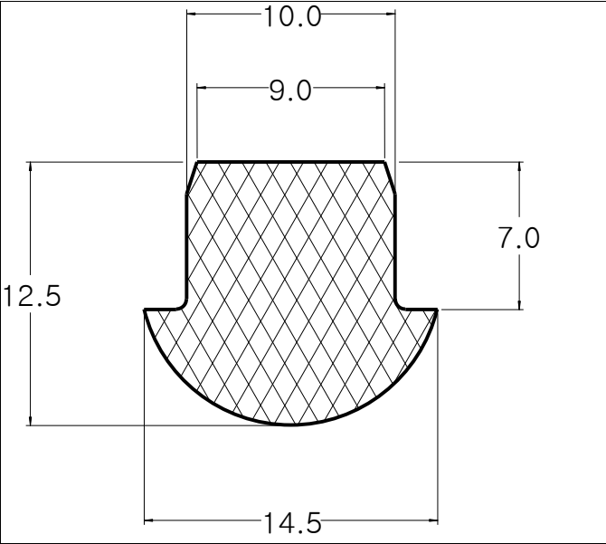
Die No: 8779 Category: T-Section
