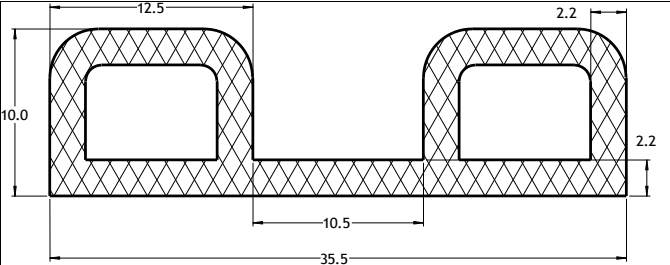
Die No: 6618 Category: P-Double
