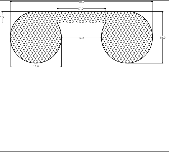
Die No: 7627 Category: P-Double
