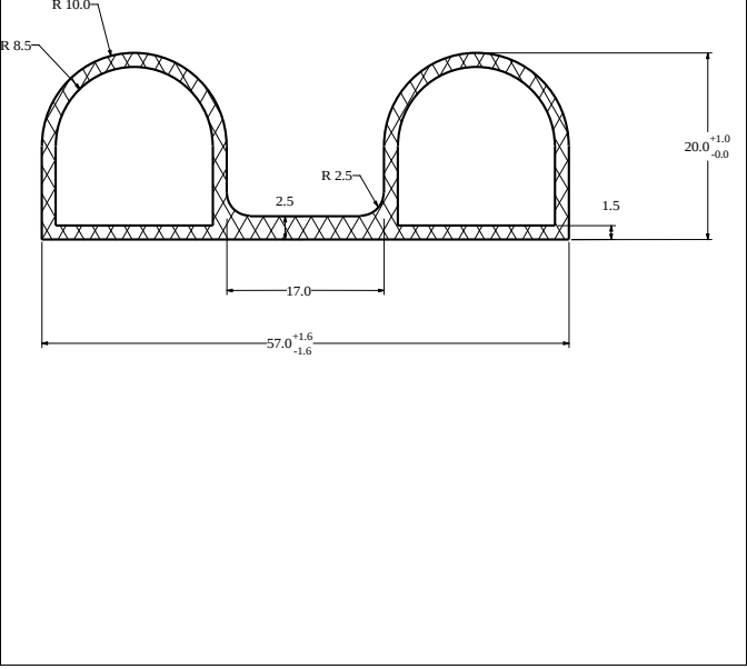
Die No: 2238 Category: P-Double
