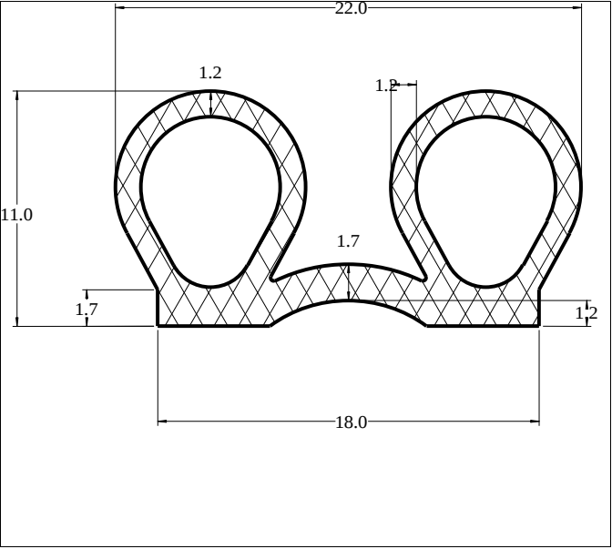
Die No: 5046 Category: P-Double
