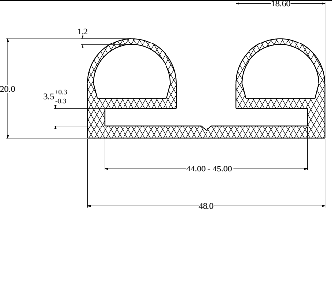
Die No: 3374 Category: P-Double
