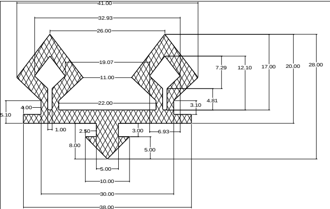
Die No: 5744 Category: P-Double
