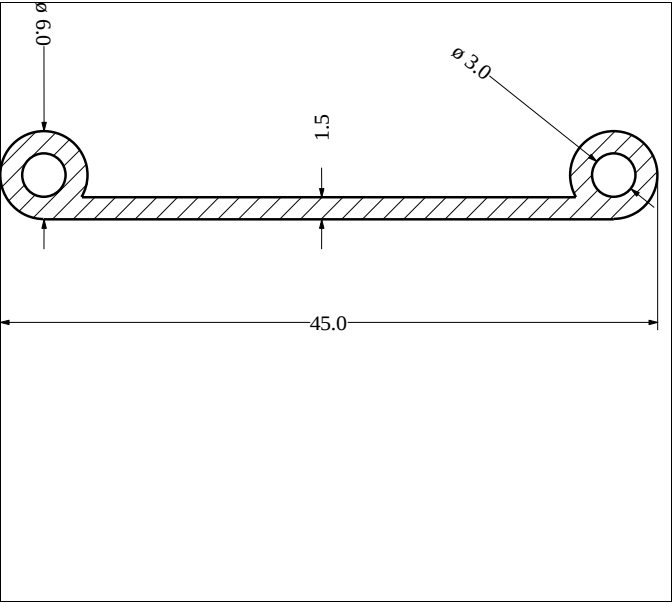
Die No: 1205 Category: P-Double
