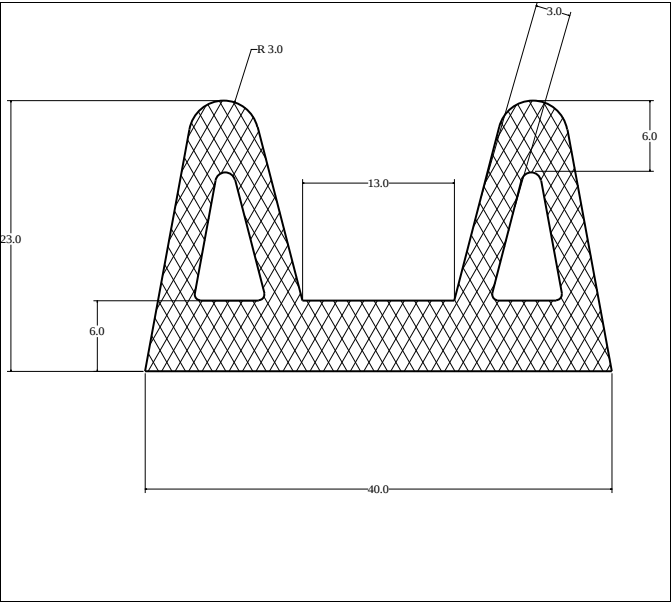
Die No: 3383 Category: P-Double
