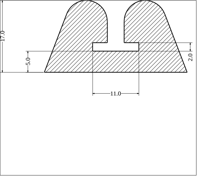
Die No: 490 Category: P-Double
