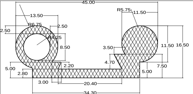
Die No: 5919 Category: P-Double
