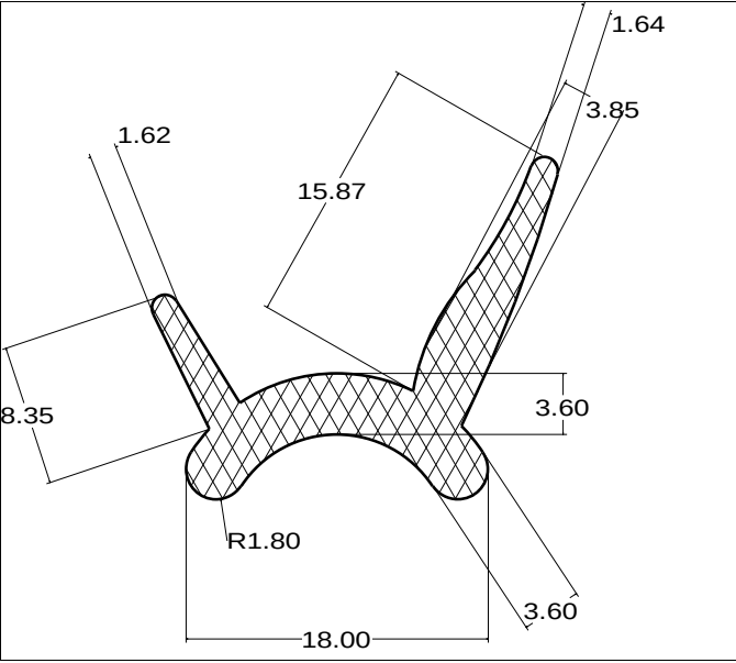
Die No: 4524 Category: Lip-Seal
