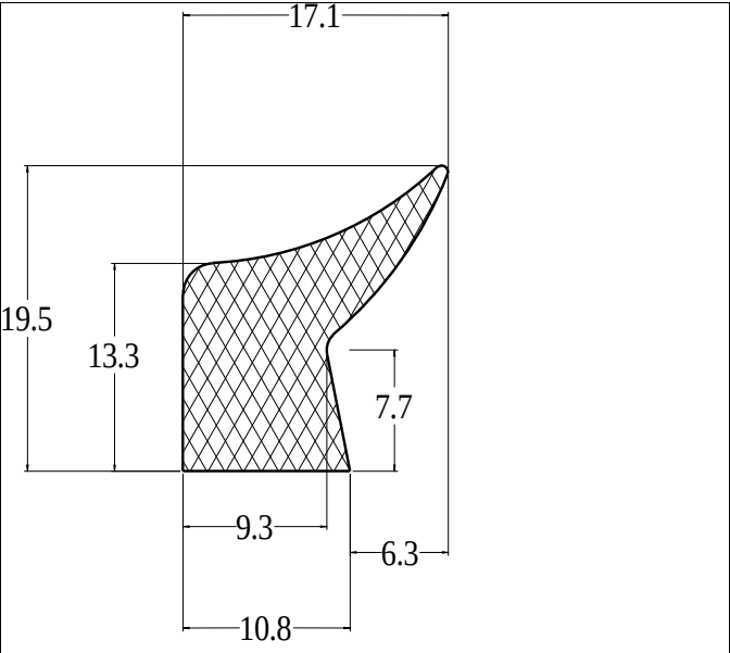
Die No: 9447 Category: Lip-Seal
