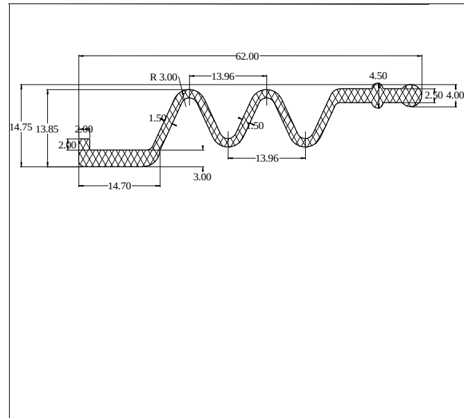
Die No: 5453
