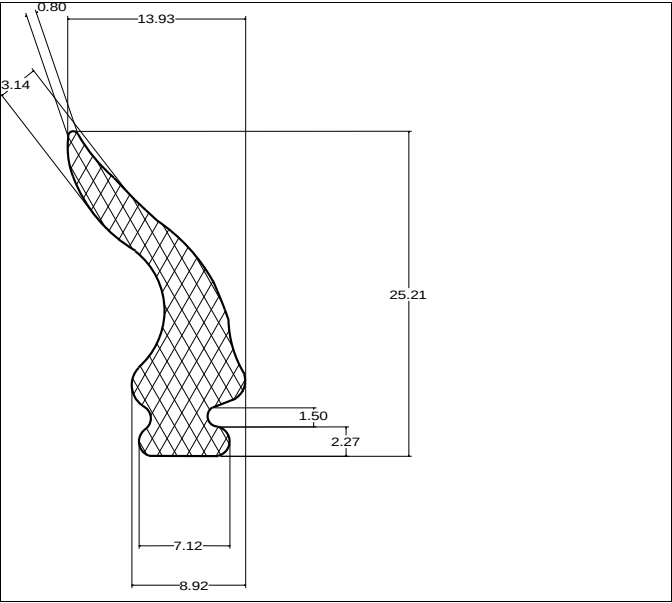
Die No: 4358 Category: Lip-Seal
