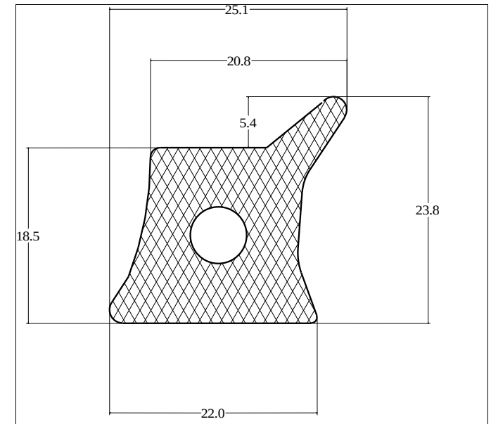
Die No: 5462
