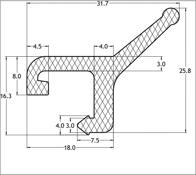
Die No: 6955 Category: Lip-Seal
