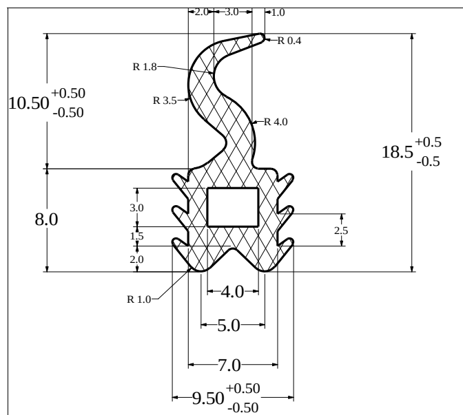
Die No: 2826
