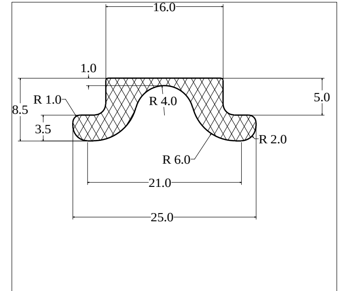
Die No: 3630
