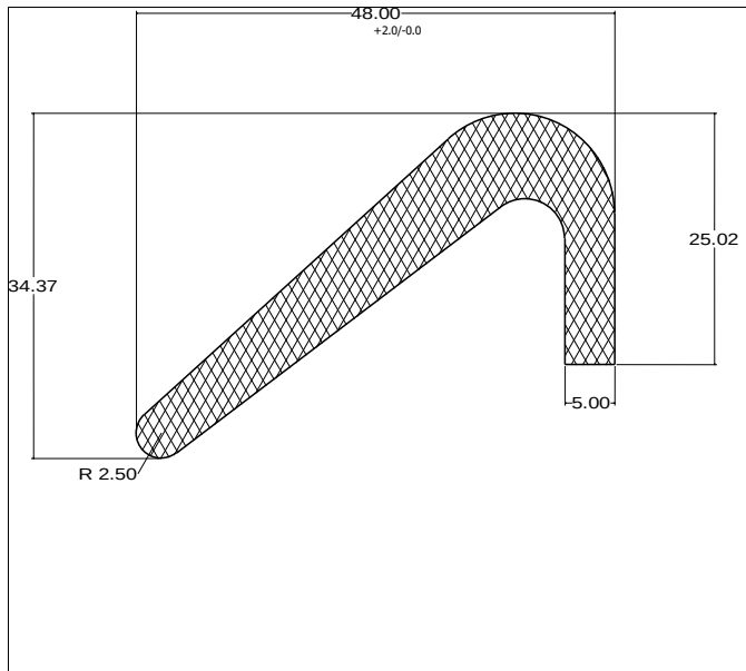
Die No: 5610
