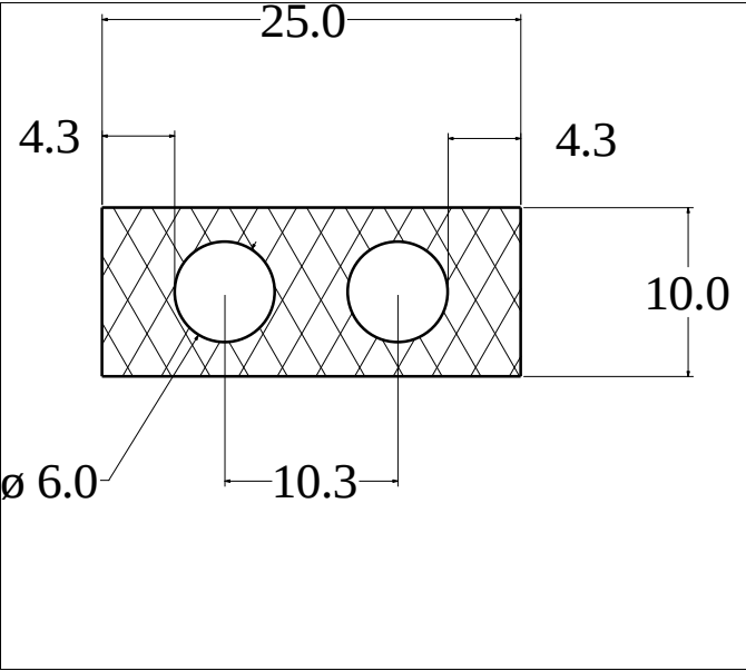
Die No: 2899 Category: Hollow Strip
