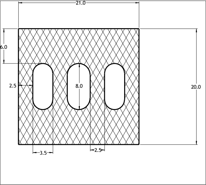
Die No: 6747 Category: Hollow Strip
