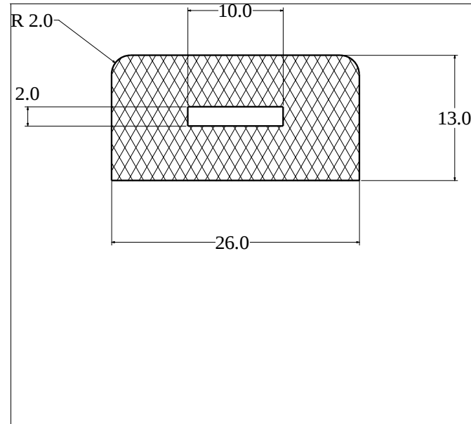
Die No: 2032 Category: Hollow Strip
