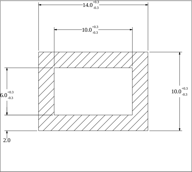
Die No: 1829 Category: Hollow Strip
