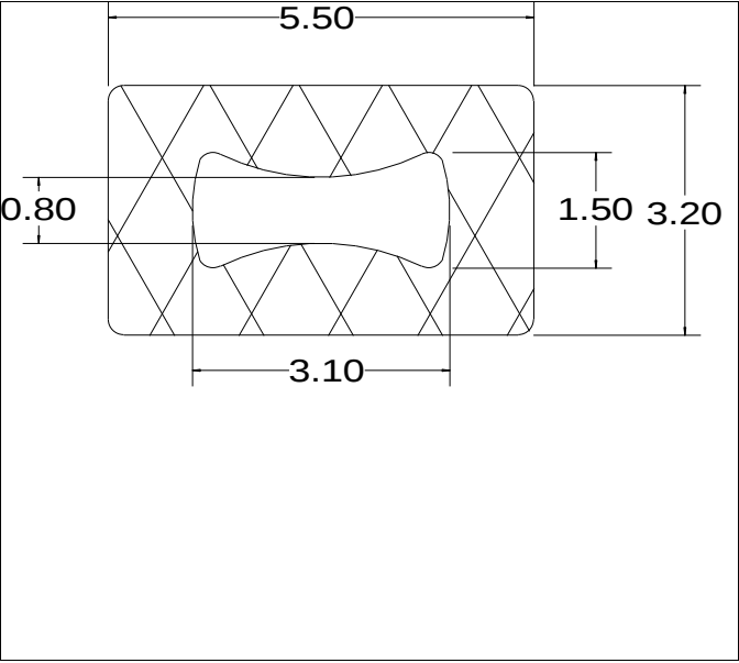
Die No: 4130 Category: Hollow Strip
