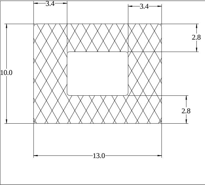
Die No: 5422 Category: Hollow Strip
