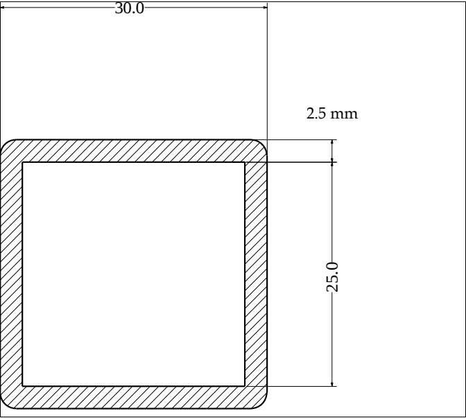
Die No: 145 Category: Hollow Strip
