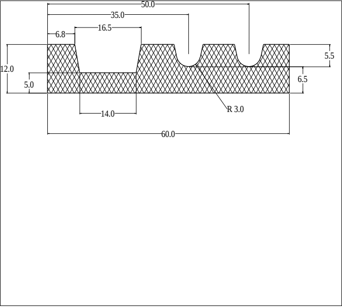
Die No: 9291 Category: Hollow Strip
