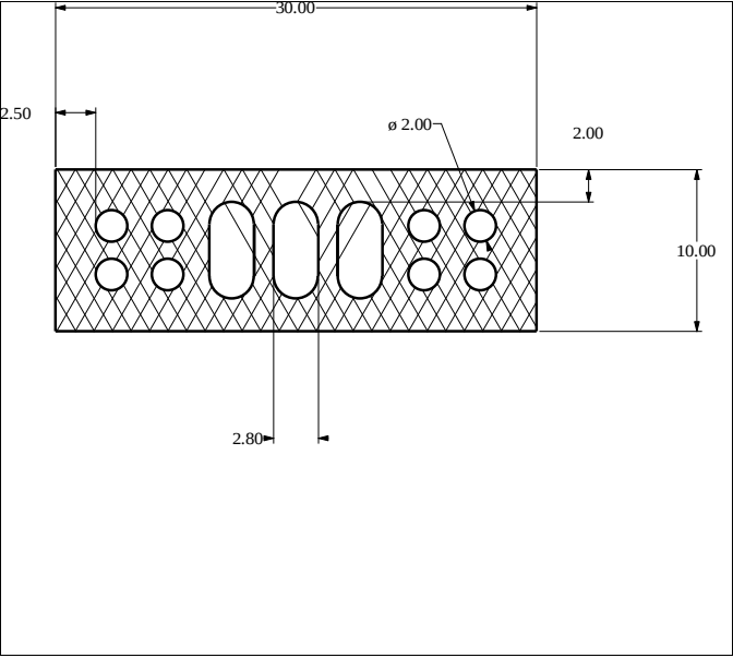
Die No: 3503 Category: Hollow Strip
