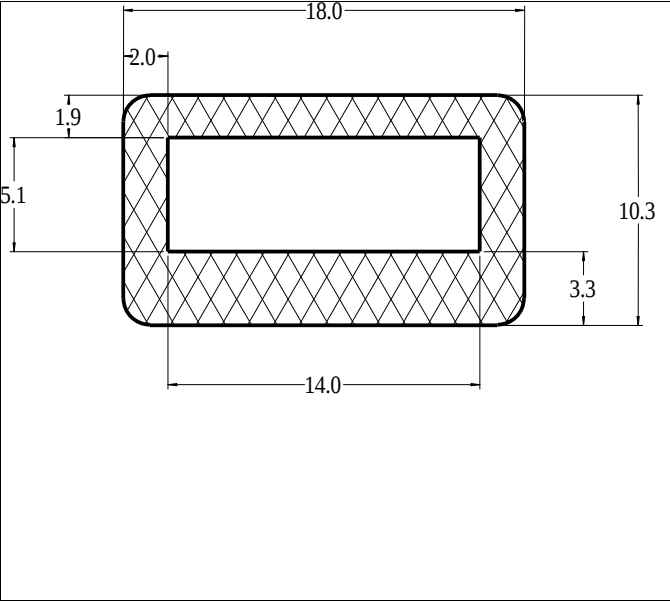
Die No: 9304 Category: Hollow Strip
