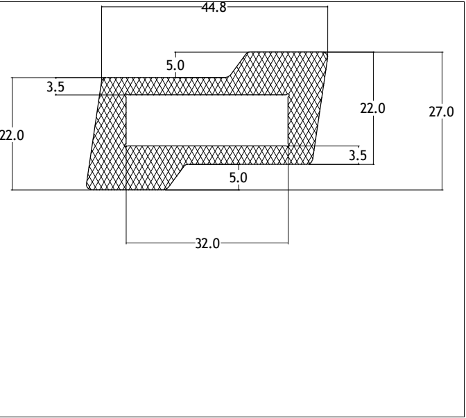
Die No: 6114 Category: Hollow Strip
