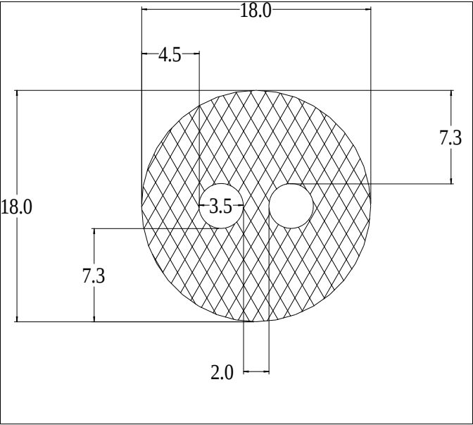
Die No: 5647 Category: Hollow Strip
