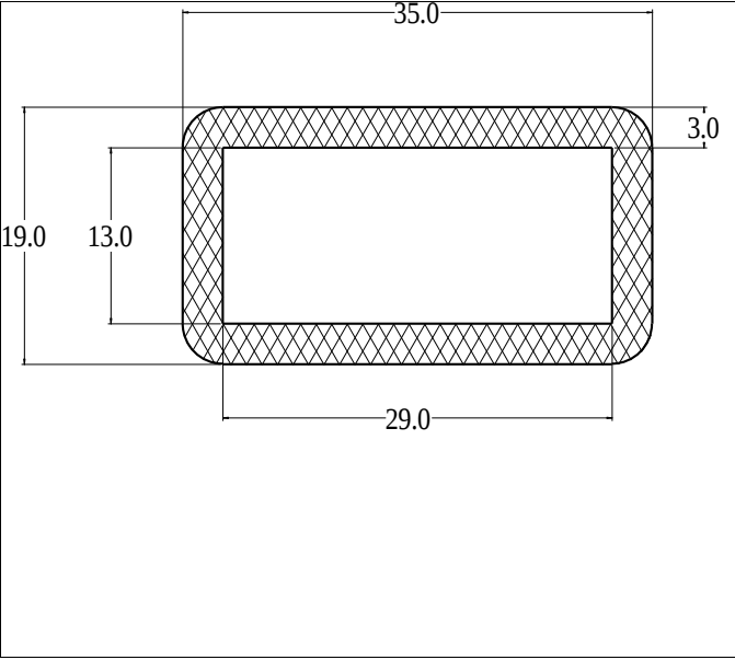
Die No: 9058 Category: Hollow Strip
