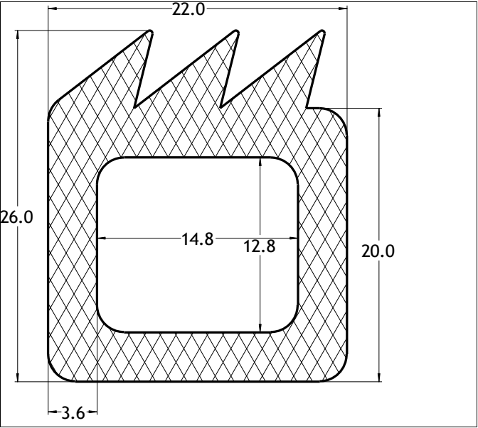
Die No: 6434 Category: Hollow Strip
