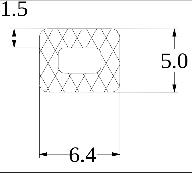
Die No: 3640 Category: Hollow Strip
