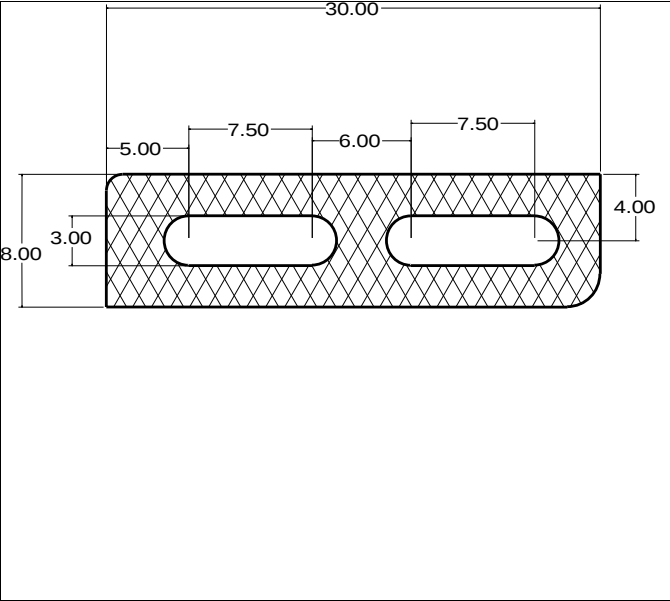
Die No: 3980 Category: Hollow Strip
