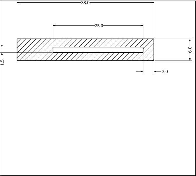
Die No: 150 Category: Hollow Strip
