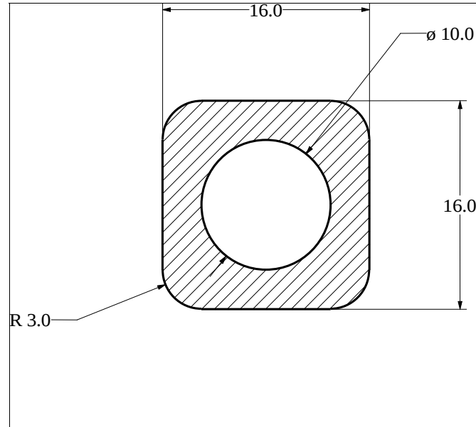
Die No: 1810 Category: Hollow Strip
