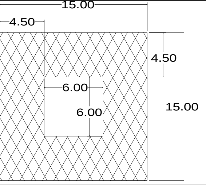
Die No: 5657 Category: Hollow Strip
