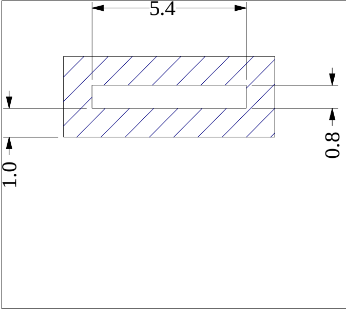
Die No: 844 Category: Hollow Strip
