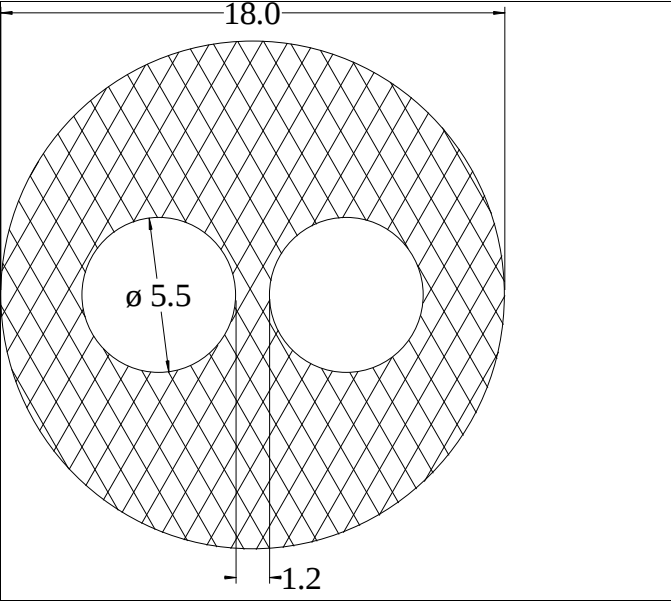
Die No: 5548 Category: Hollow Strip
