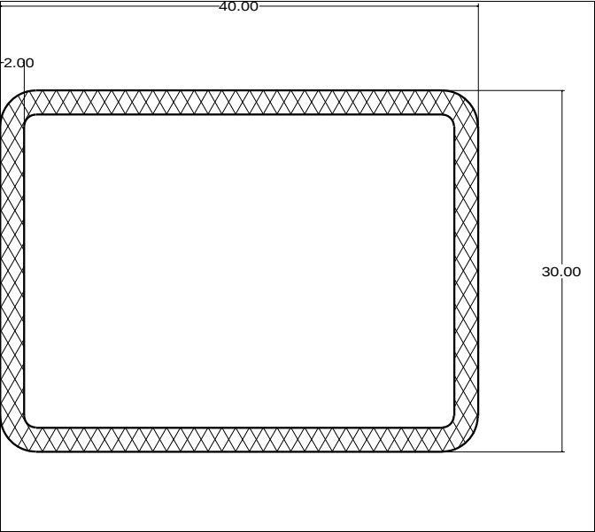
Die No: 3977 Category: Hollow Strip
