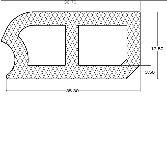
Die No: 4020 Category: Hollow Strip
