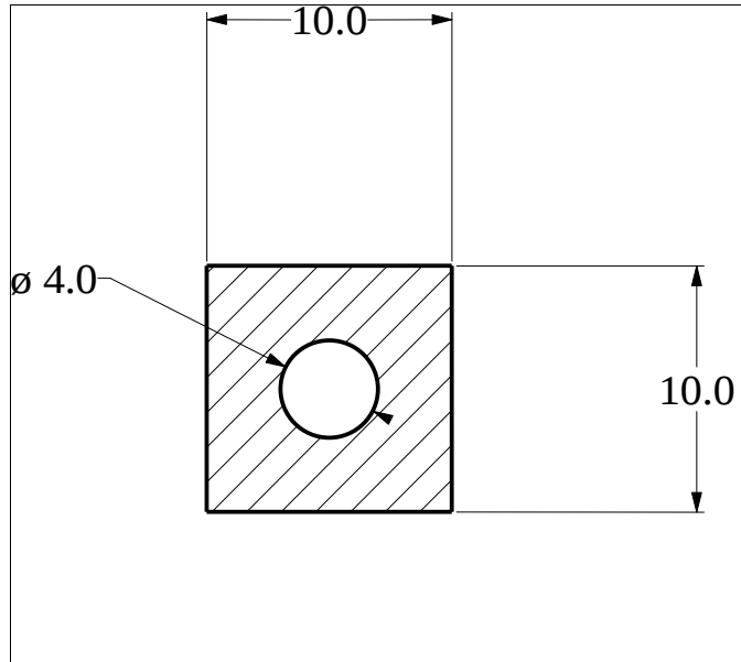
Die No: 2030 Category: Hollow Strip
