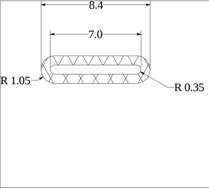
Die No: 3093 Category: Hollow Strip
