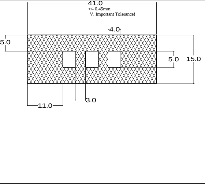
Die No: 5017 Category: Hollow Strip
