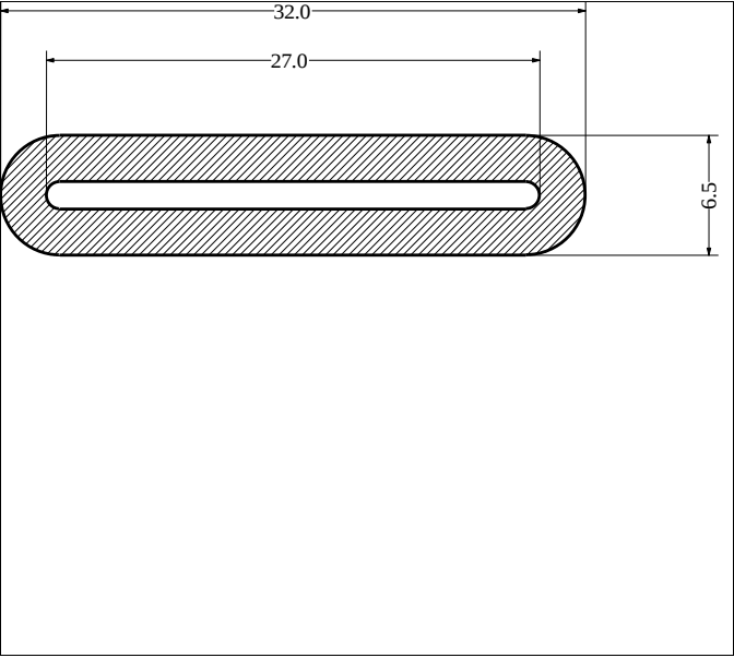
Die No: 1272 Category: Hollow Strip
