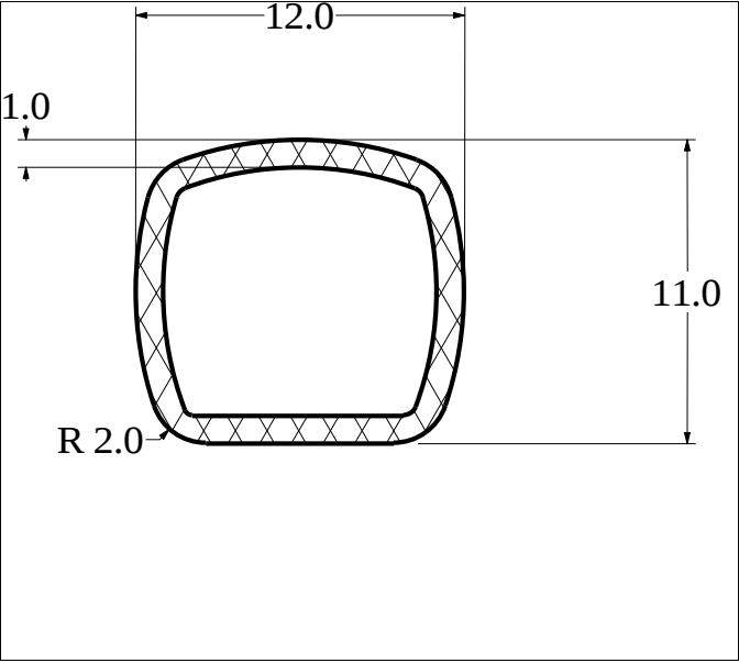
Die No: 2290 Category: Hollow Strip
