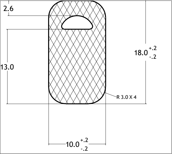
Die No: 6113 Category: Hollow Strip
