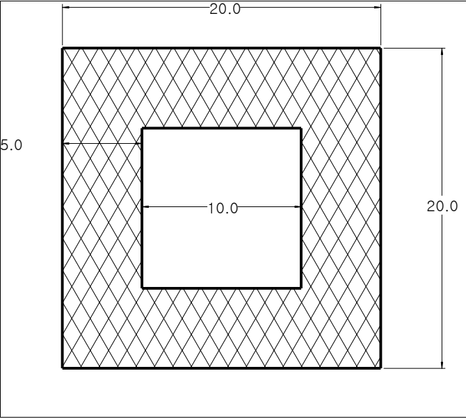
Die No: 7883 Category: Hollow Strip
