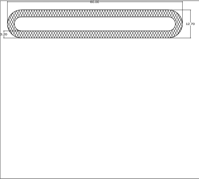
Die No: 4256 Category: Hollow Strip
