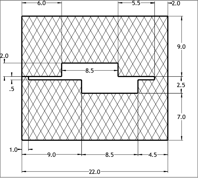
Die No: 7047 Category: Hollow Strip
