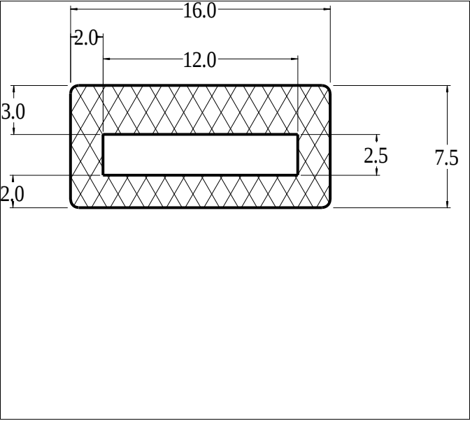
Die No: 9045 Category: Hollow Strip
