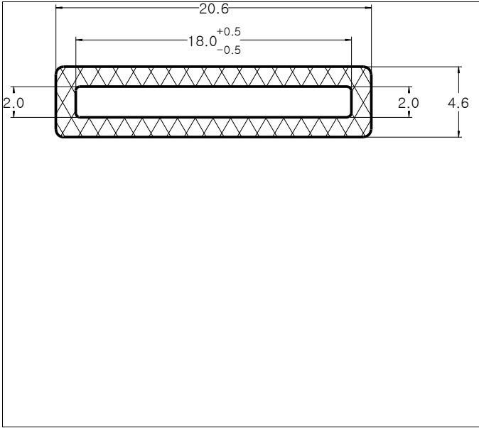
Die No: 2605 Category: Hollow Strip
