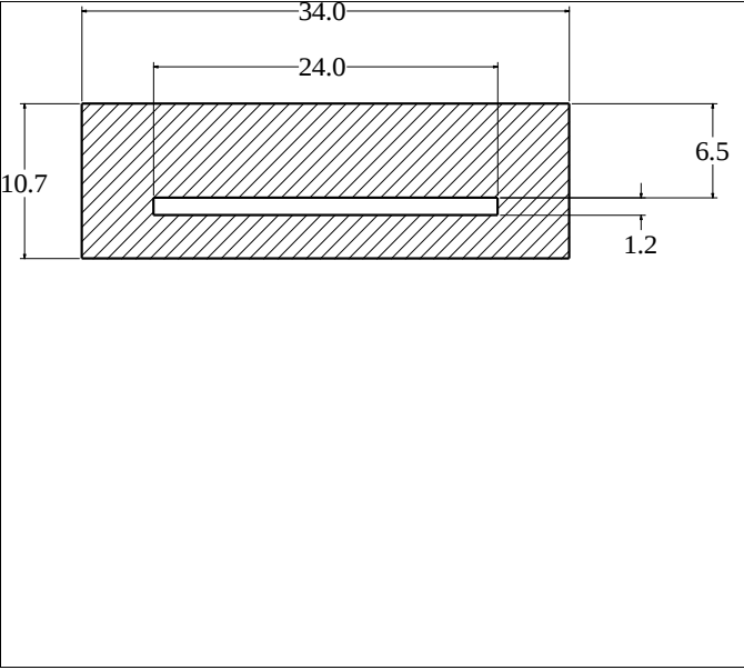
Die No: 1872 Category: Hollow Strip
