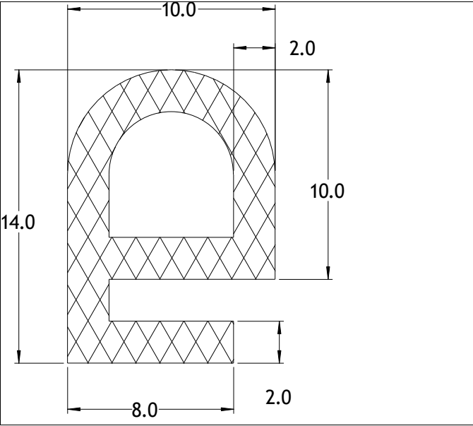
Die No: 6369 Category: E-Section
