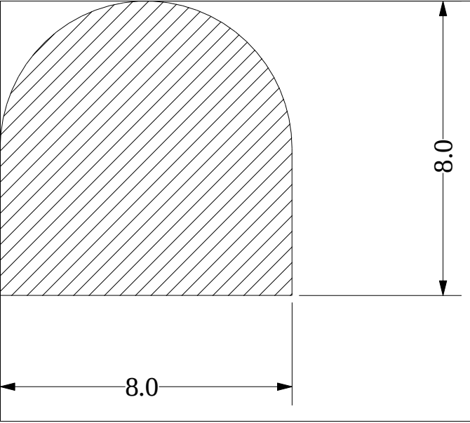
Die No: 1640 Category: D-Solid
