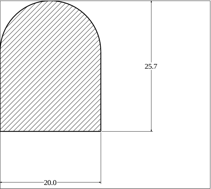
Die No: 976 Category: D-Solid
