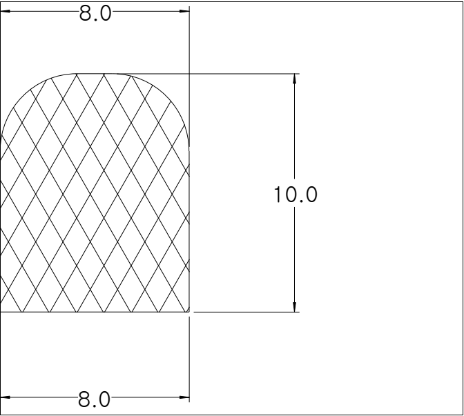
Die No: 8906 Category: D-Solid
