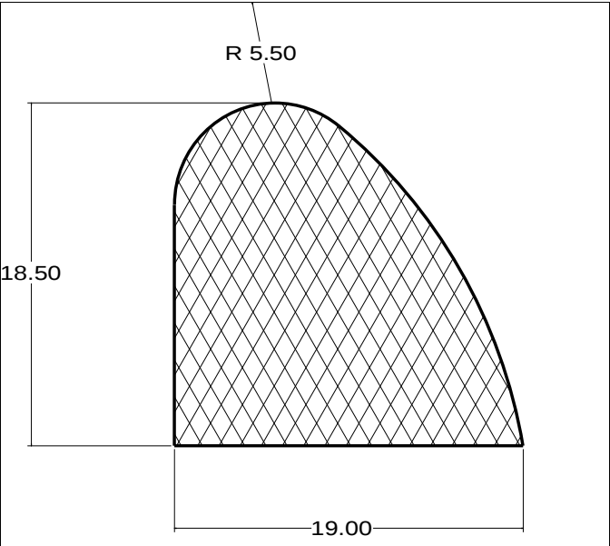
Die No: 5625 Category: D-Solid
