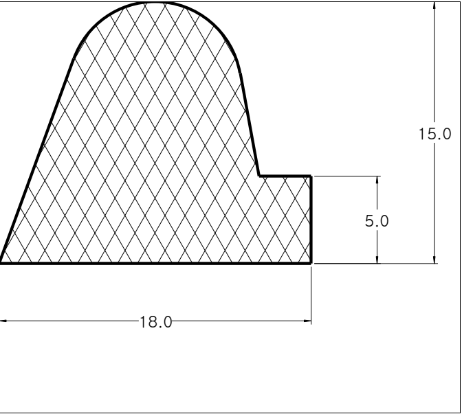
Die No: 8833 Category: D-Solid
