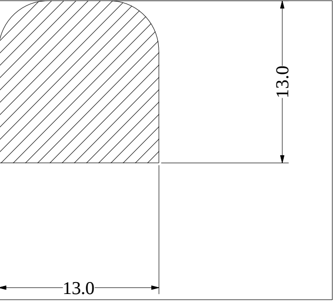
Die No: 374 Category: D-Solid
