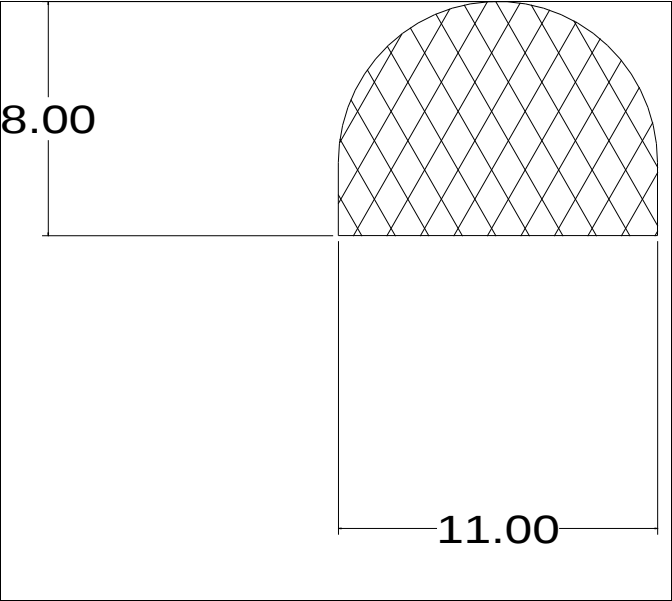
Die No: 4478 Category: D-Solid
