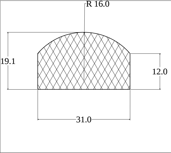
Die No: 2634 Category: D-Solid
