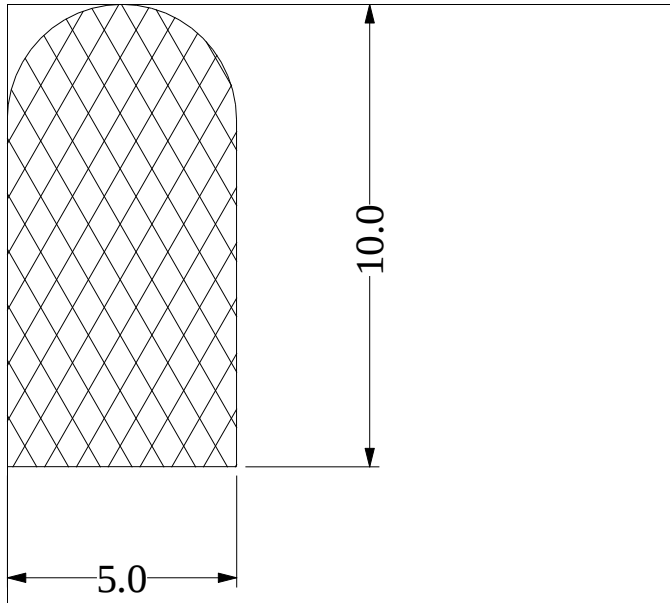
Die No: 1847 Category: D-Solid
