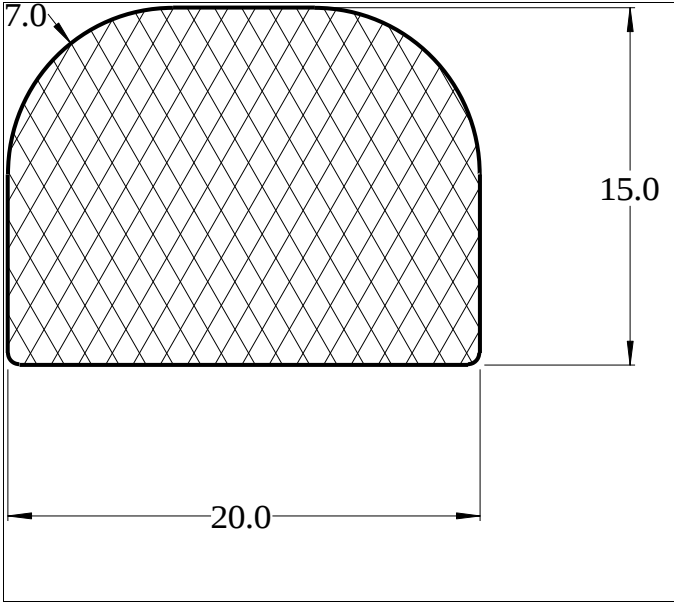
Die No: 4963 Category: D-Solid
