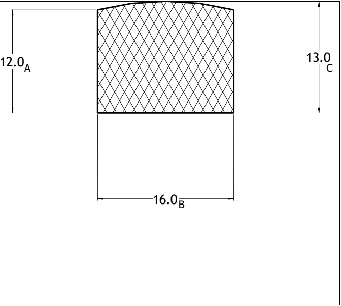
Die No: 6990 Category: D-Solid
