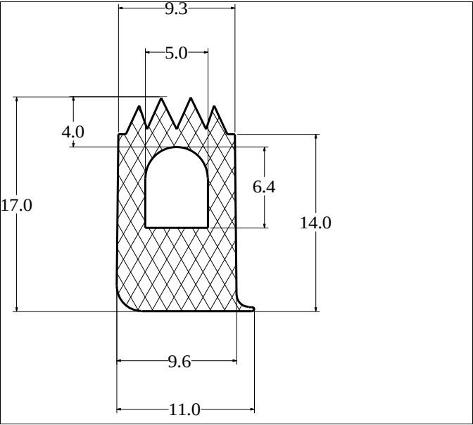
Die No: 2119 Category: D-Hollow
