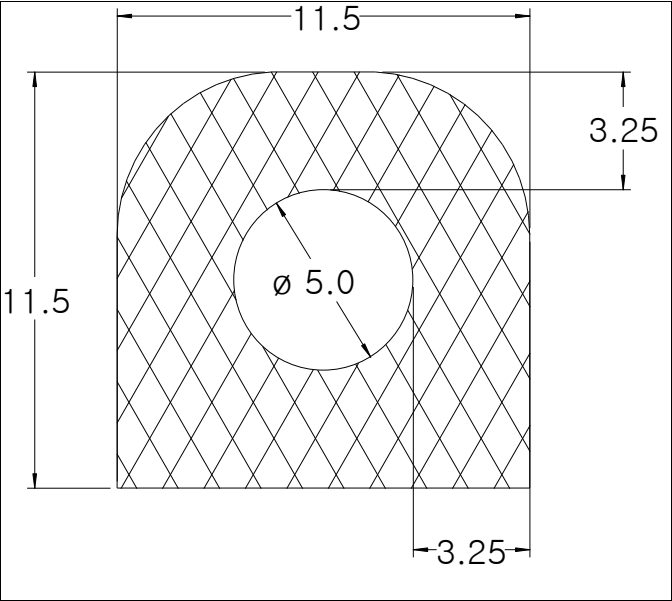
Die No: 8406 Category: D-Hollow
