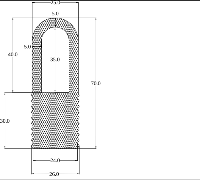
Die No: 5523 Category: D-Hollow
