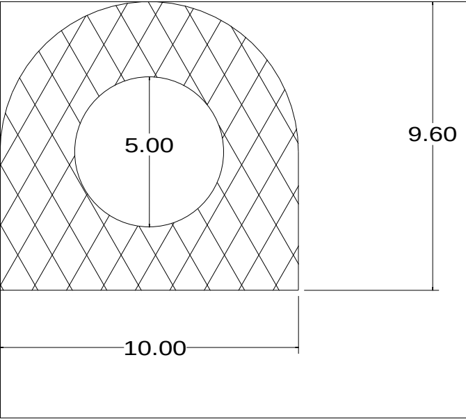
Die No: 4172 Category: D-Hollow
