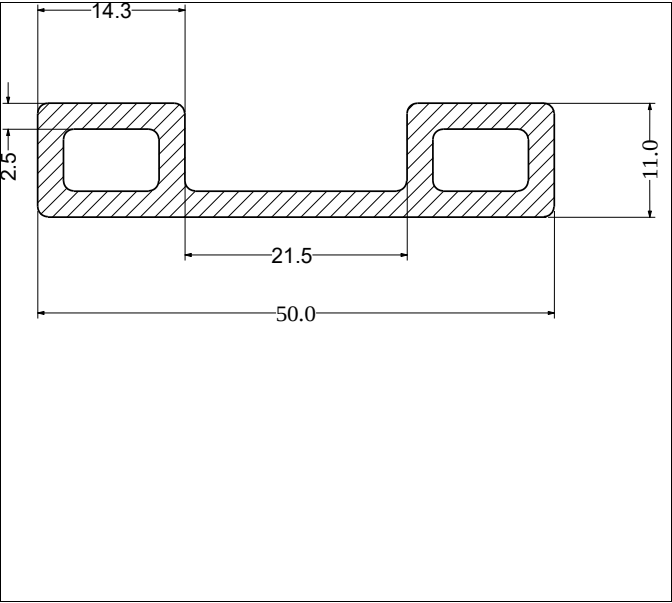
Die No: 9329 Category: D-Hollow
