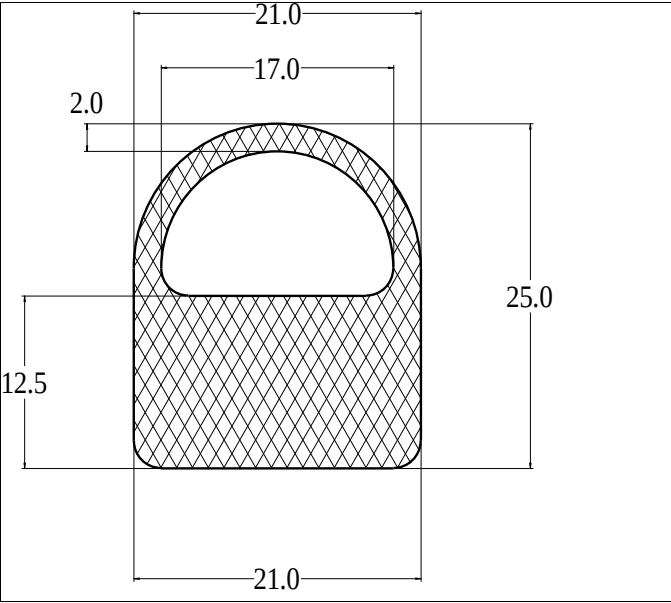
Die No: 2250 Category: D-Hollow
