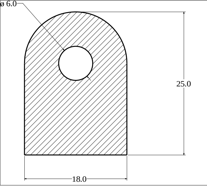
Die No: 1020 Category: D-Hollow
