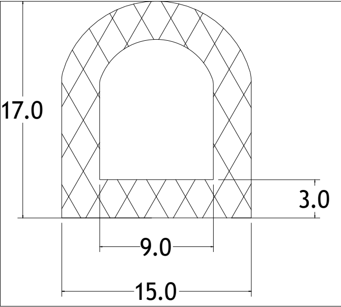
Die No: 7059 Category: D-Hollow
