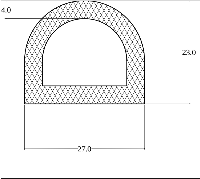
Die No: 3373 Category: D-Hollow
