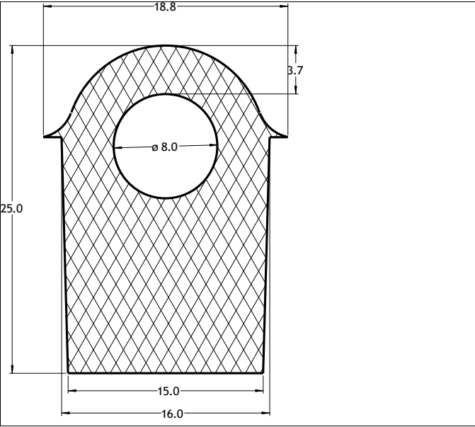
Die No: 6124 Category: D-Hollow
