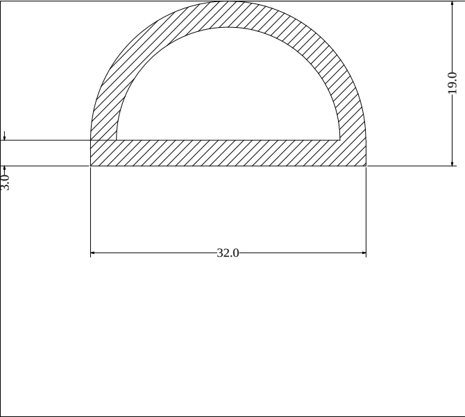
Die No: 595 Category: D-Hollow
