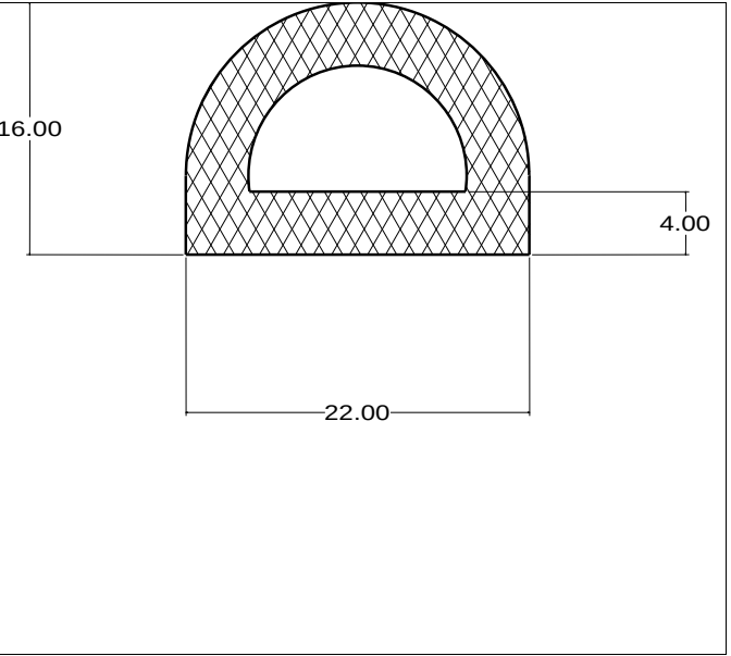
Die No: 4526 Category: D-Hollow
