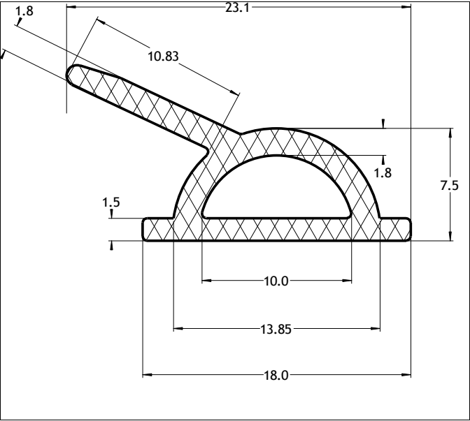
Die No: 7313 Category: D-Hollow
