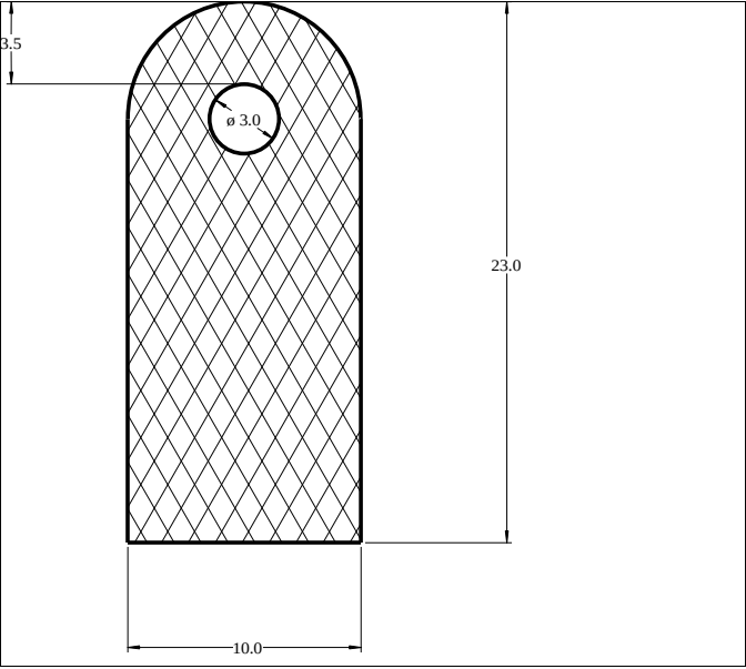
Die No: 5328 Category: D-Hollow
