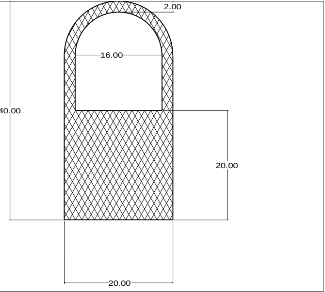
Die No: 4497 Category: D-Hollow
