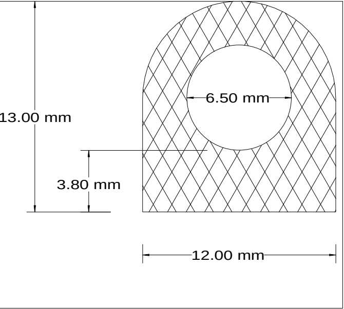
Die No: 3866 Category: D-Hollow
