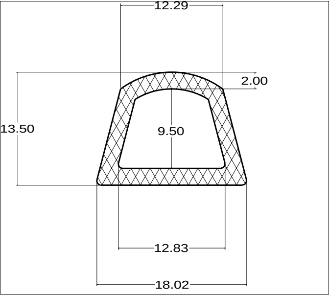
Die No: 4435 Category: D-Hollow
