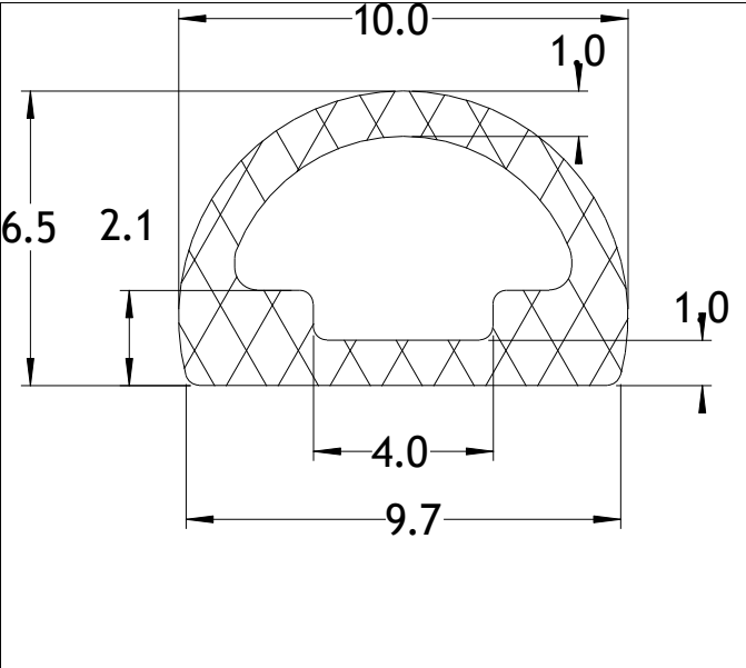
Die No: 6442 Category: D-Hollow
