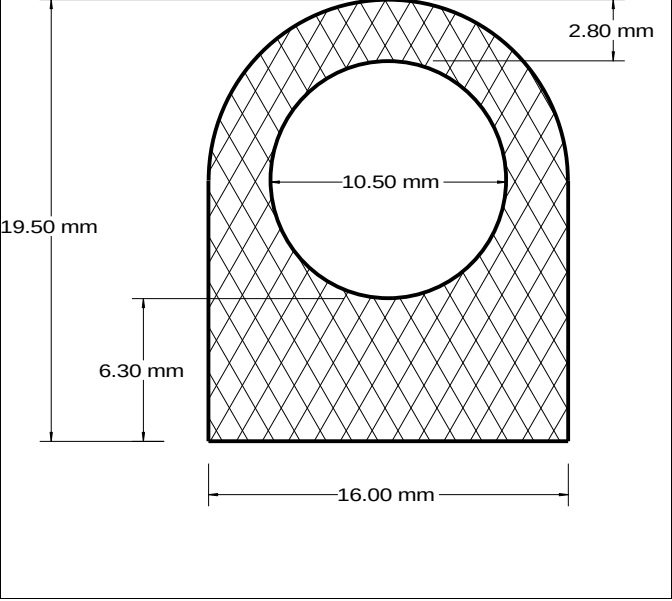
Die No: 3864 Category: D-Hollow
