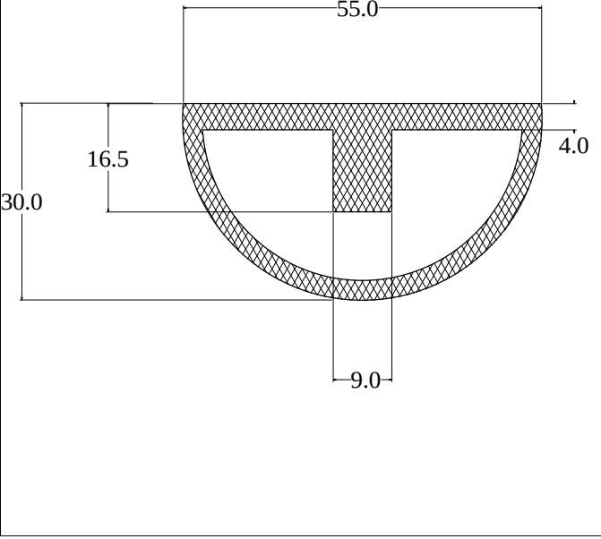
Die No: 2931 Category: D-Hollow
