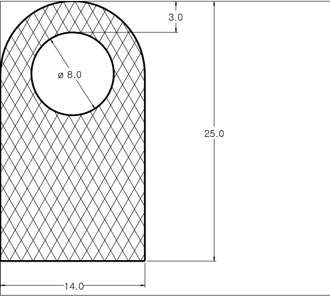
Die No: 7669 Category: D-Hollow
