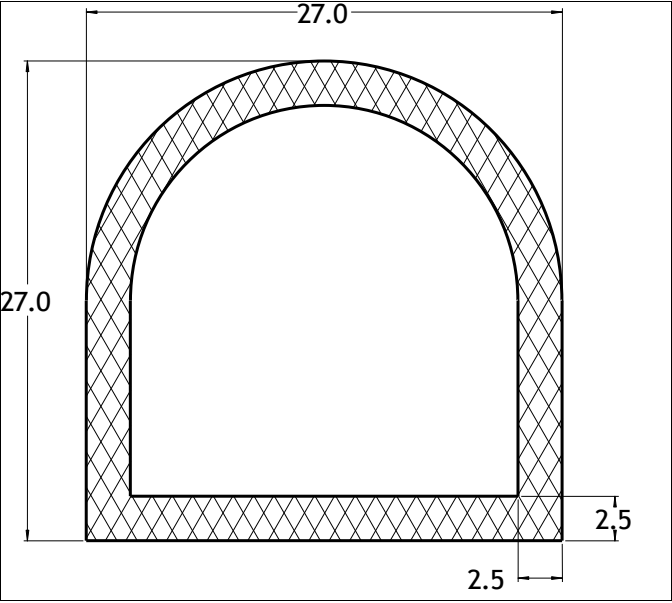
Die No: 6684 Category: D-Hollow
