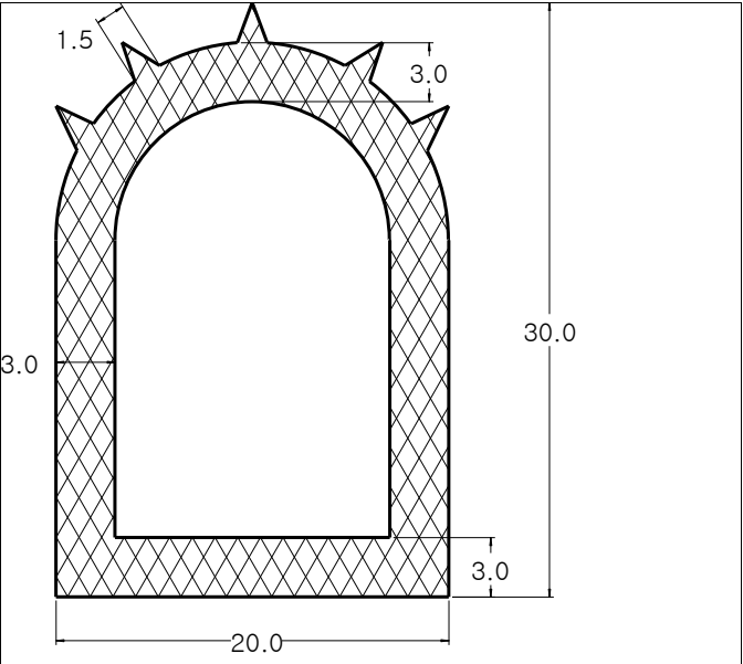
Die No: 8248 Category: D-Hollow
