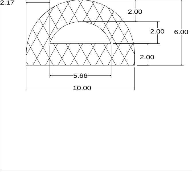
Die No: 5803 Category: D-Hollow
