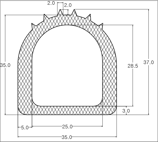
Die No: 8957 Category: D-Hollow
