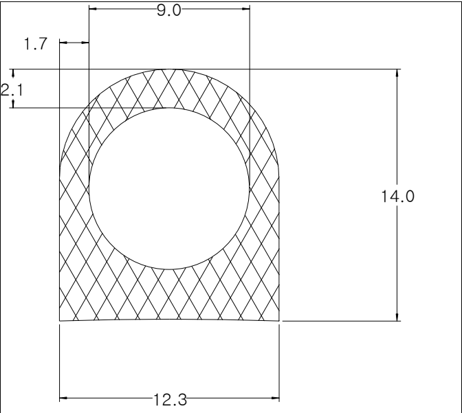
Die No: 8811 Category: D-Hollow
