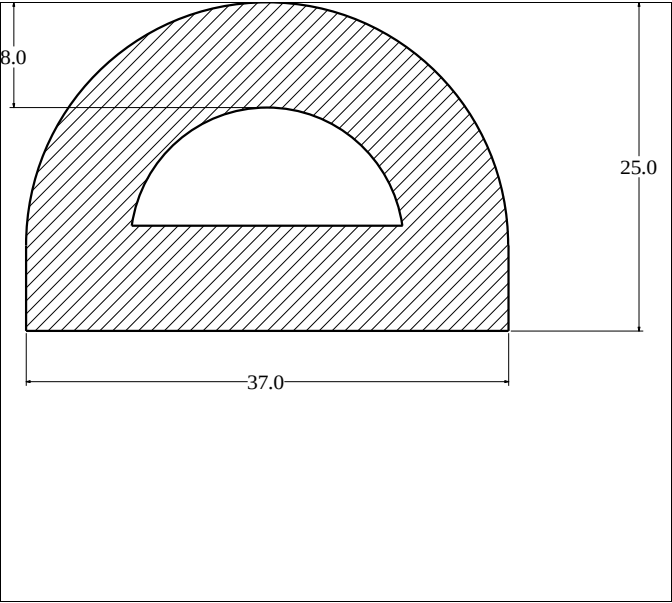
Die No: 1213 Category: D-Hollow
