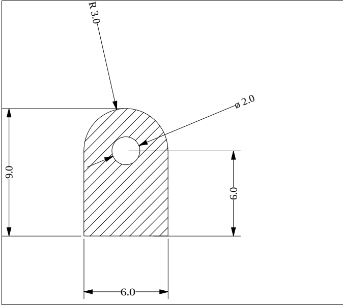
Die No: 797 Category: D-Hollow
