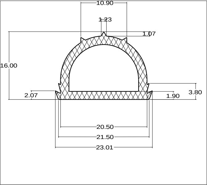
Die No: 4458 Category: D-Hollow
