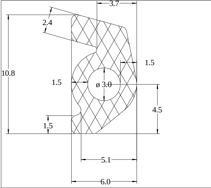
Die No: 5166 Category: D-Hollow
