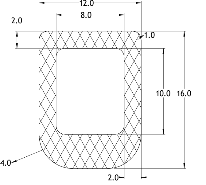
Die No: 6013 Category: D-Hollow
