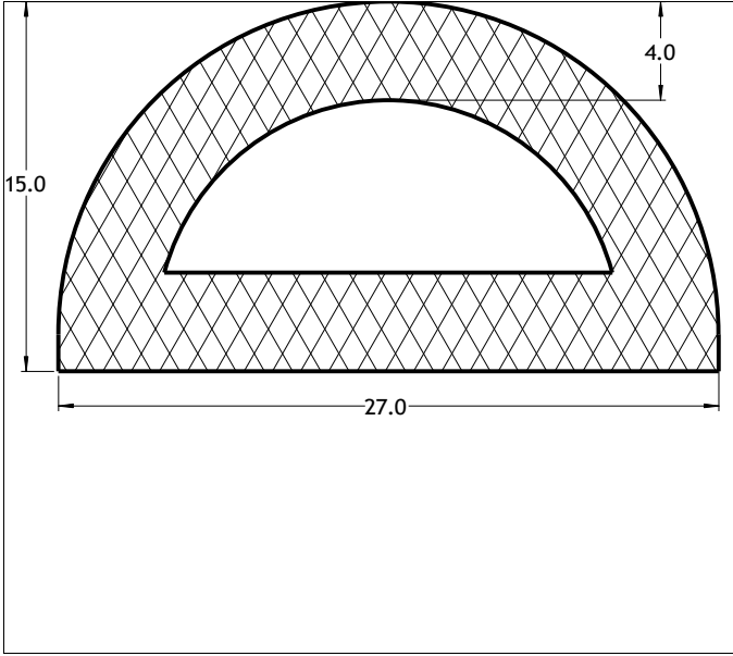
Die No: 6720 Category: D-Hollow
