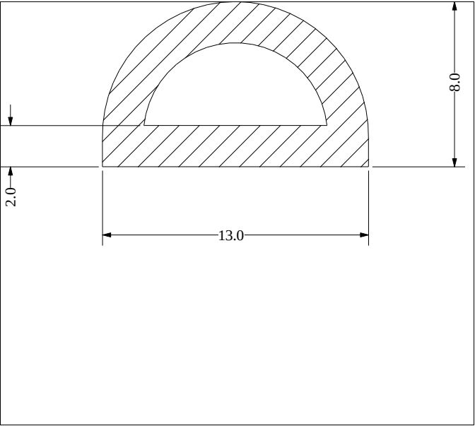
Die No: 794 Category: D-Hollow
