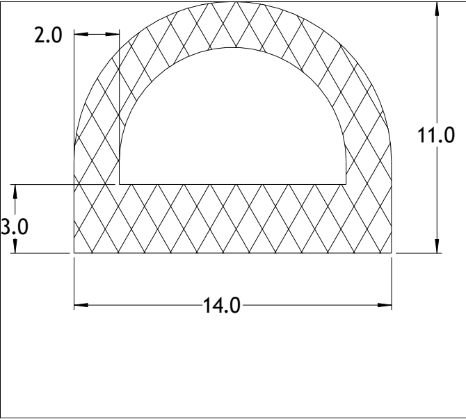
Die No: 6121 Category: D-Hollow
