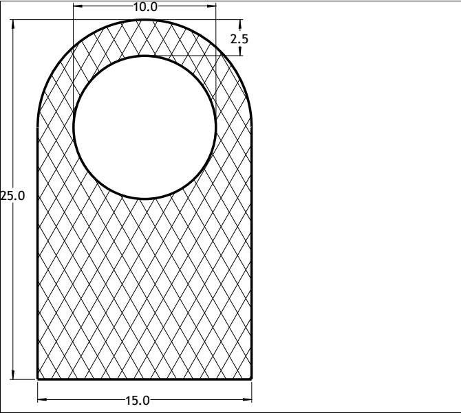
Die No: 6440 Category: D-Hollow
