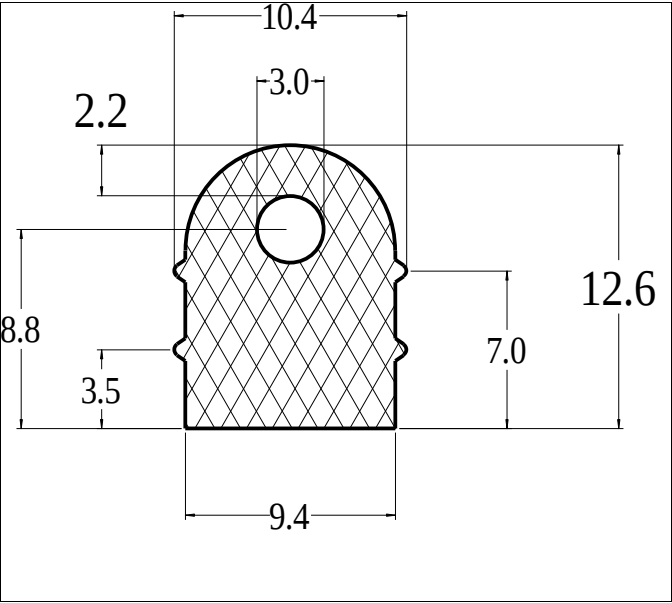
Die No: 9167 Category: D-Hollow
