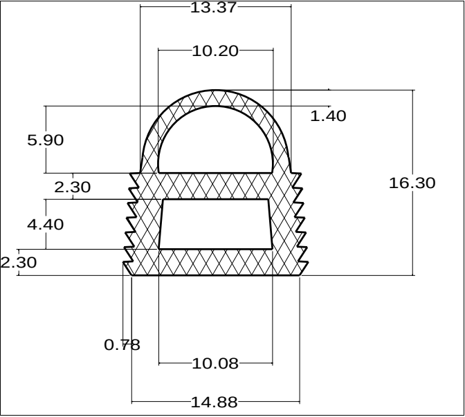
Die No: 4436 Category: D-Hollow
