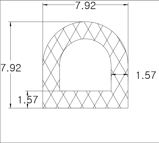
Die No: 8178 Category: D-Hollow
