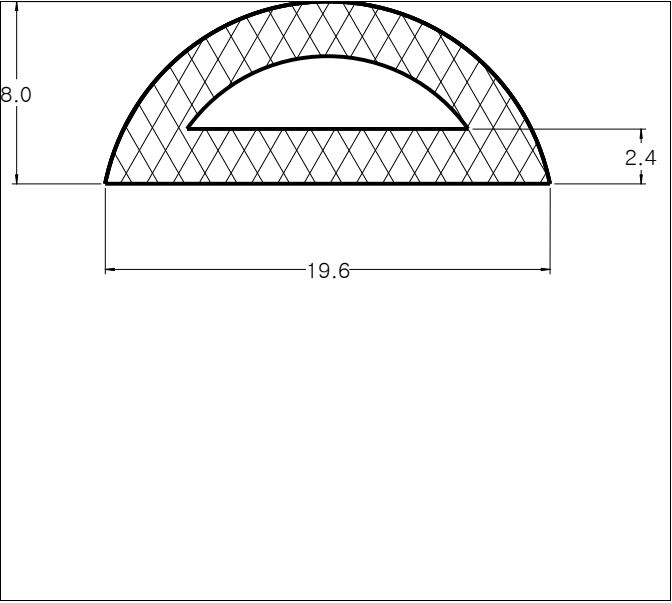
Die No: 8670 Category: D-Hollow
