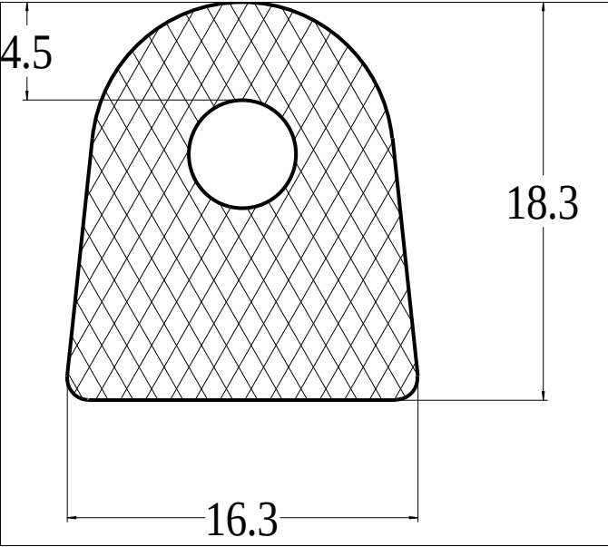
Die No: 9210 Category: D-Hollow
