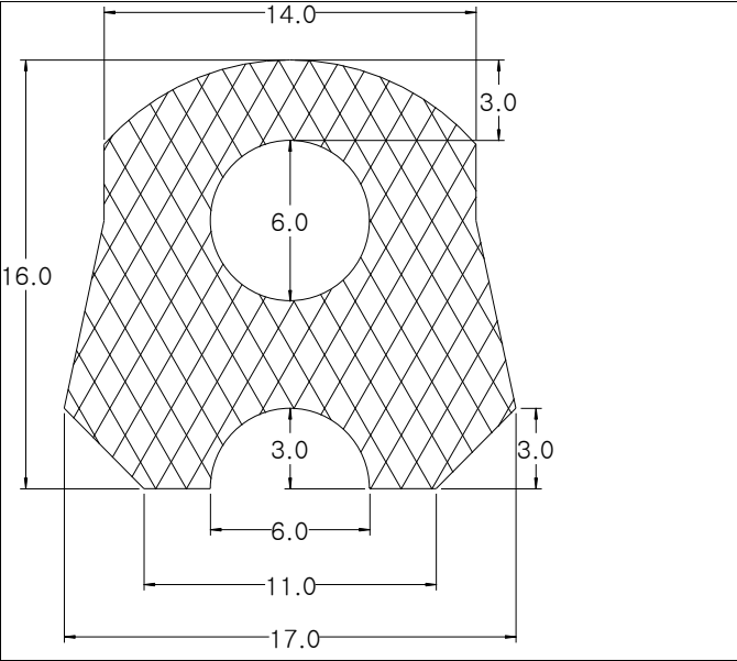
Die No: 8416 Category: D-Hollow
