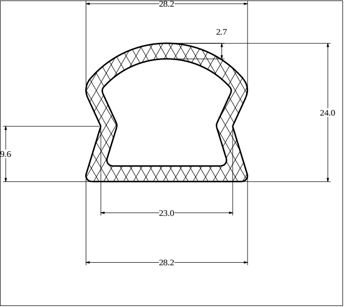
Die No: 2215 Category: D-Hollow
