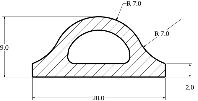
Die No: 1087 Category: D-Hollow
