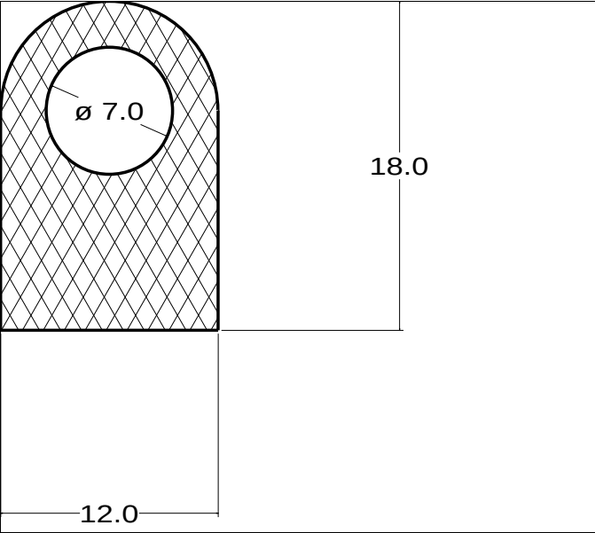
Die No: 4718 Category: D-Hollow
