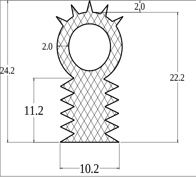
Die No: 9330 Category: D-Hollow
