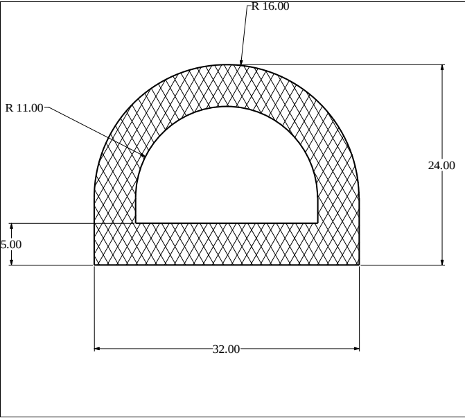
Die No: 3604 Category: D-Hollow
