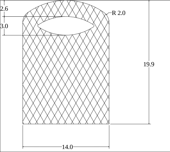
Die No: 3171 Category: D-Hollow
