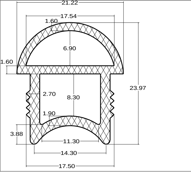
Die No: 5581 Category: D-Hollow
