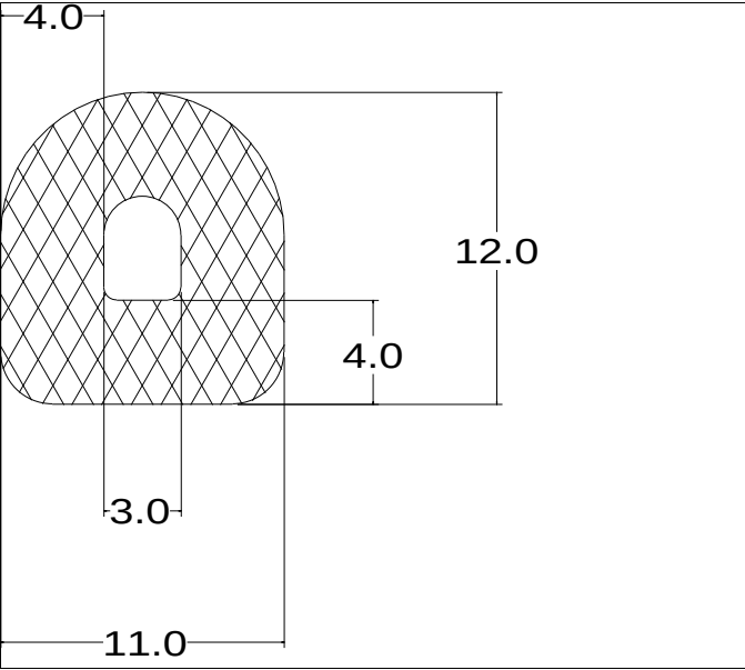
Die No: 4810 Category: D-Hollow
