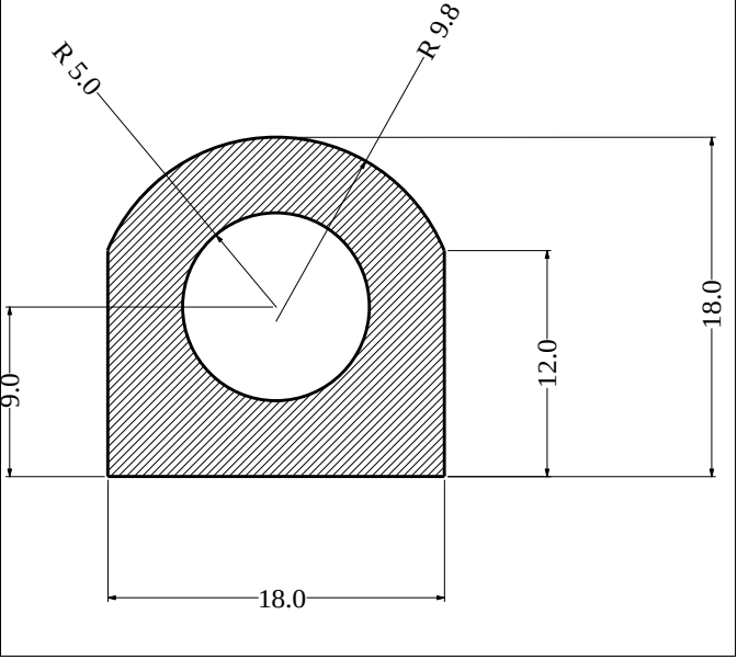
Die No: 1665 Category: D-Hollow
