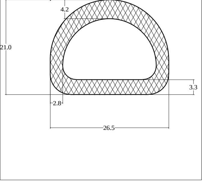
Die No: 5455 Category: D-Hollow
