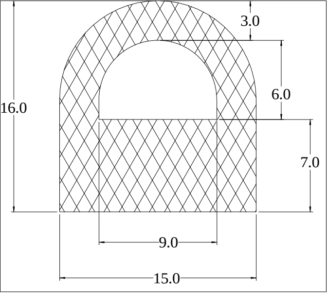
Die No: 5528 Category: D-Hollow
