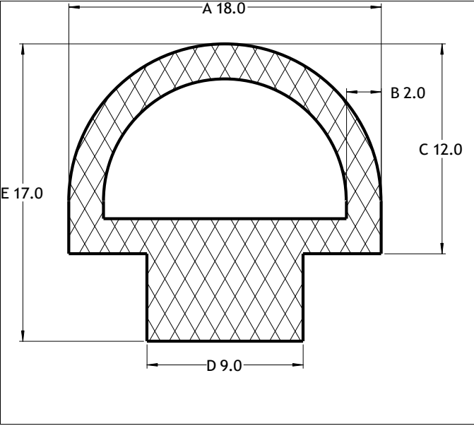
Die No: 6898 Category: D-Hollow
