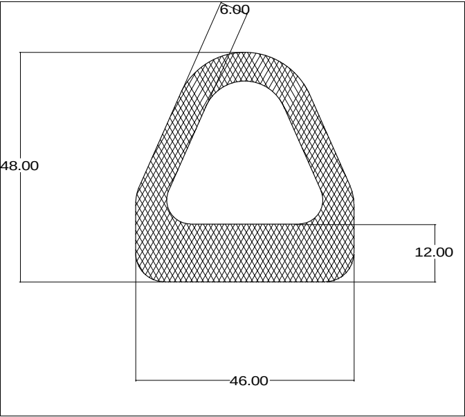
Die No: 4519 Category: D-Hollow
