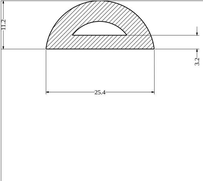
Die No: 598 Category: D-Hollow
