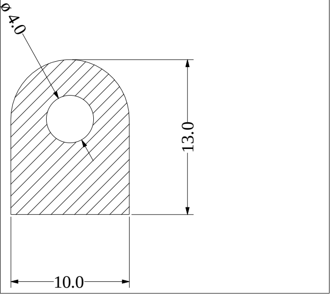
Die No: 1478 Category: D-Hollow
