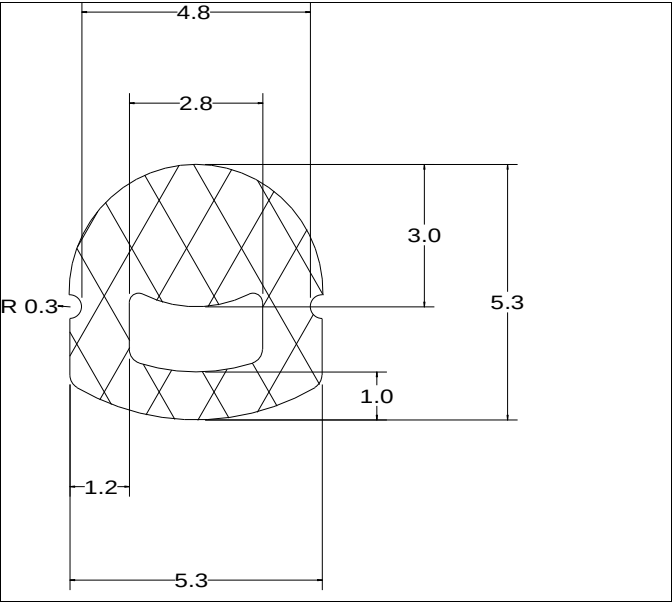
Die No: 4760 Category: D-Hollow
