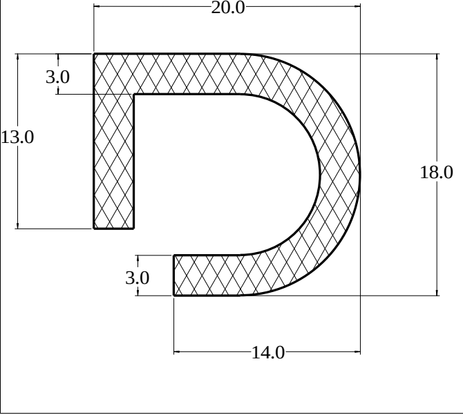
Die No: 5006 Category: D-Hollow
