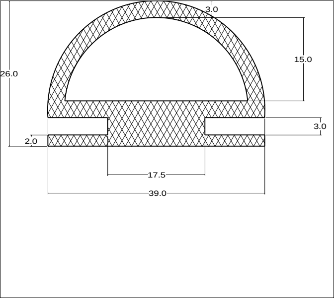
Die No: 5228 Category: D-Hollow
