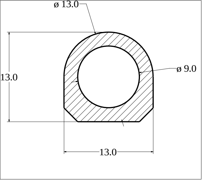
Die No: 825 Category: D-Hollow
