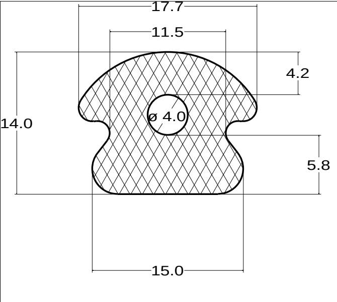
Die No: 4709 Category: D-Hollow
