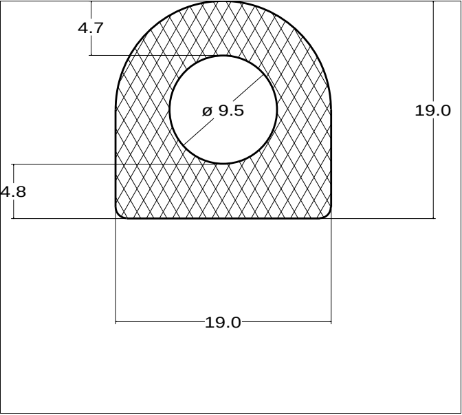
Die No: 4761 Category: D-Hollow
