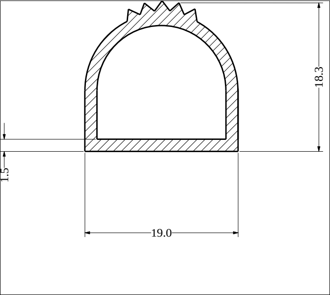
Die No: 329 Category: D-Hollow
