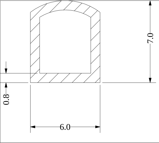
Die No: 1503 Category: D-Hollow
