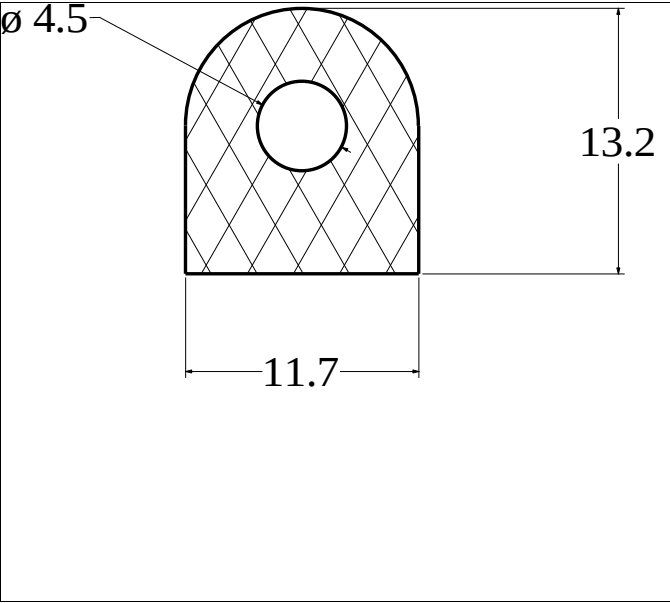
Die No: 2650 Category: D-Hollow
