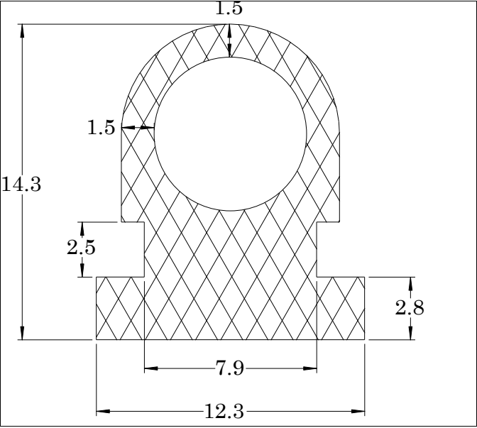
Die No: 7660 Category: D-Hollow
