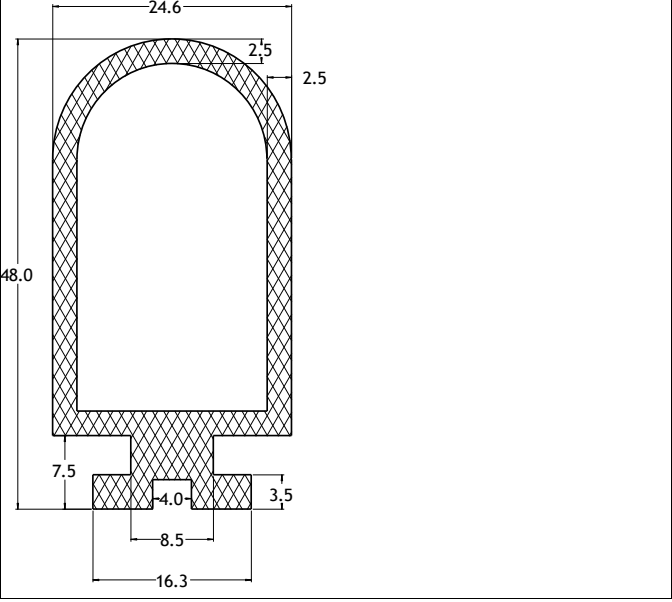
Die No: 6550 Category: D-Hollow
