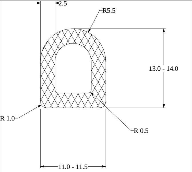
Die No: 3469 Category: D-Hollow
