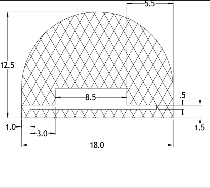
Die No: 7049 Category: D-Hollow
