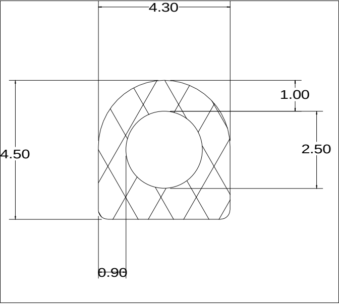
Die No: 4200 Category: D-Hollow
