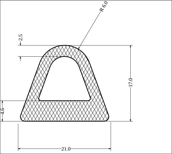
Die No: 1712 Category: D-Hollow
