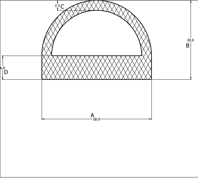
Die No: 6893 Category: D-Hollow
