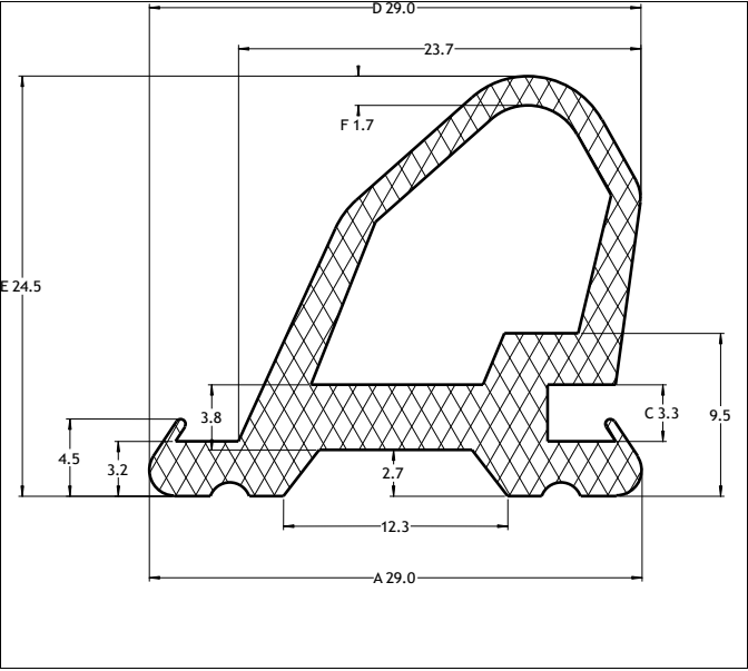
Die No: 6889 Category: D-Hollow
