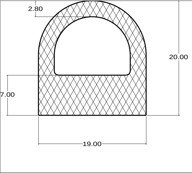
Die No: 5690 Category: D-Hollow
