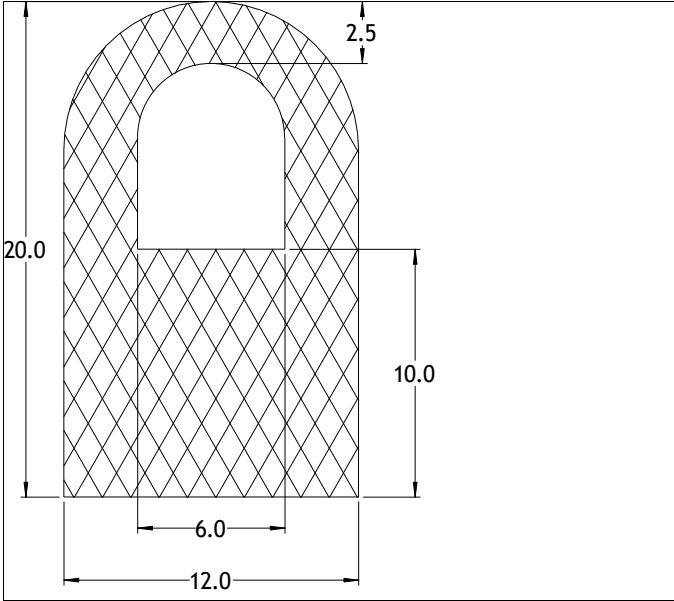
Die No: 7018 Category: D-Hollow
