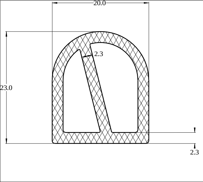
Die No: 5124 Category: D-Hollow
