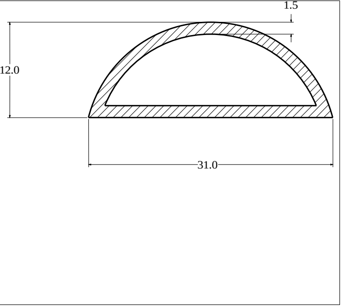
Die No: 869 Category: D-Hollow
