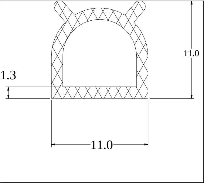
Die No: 2239 Category: D-Hollow
