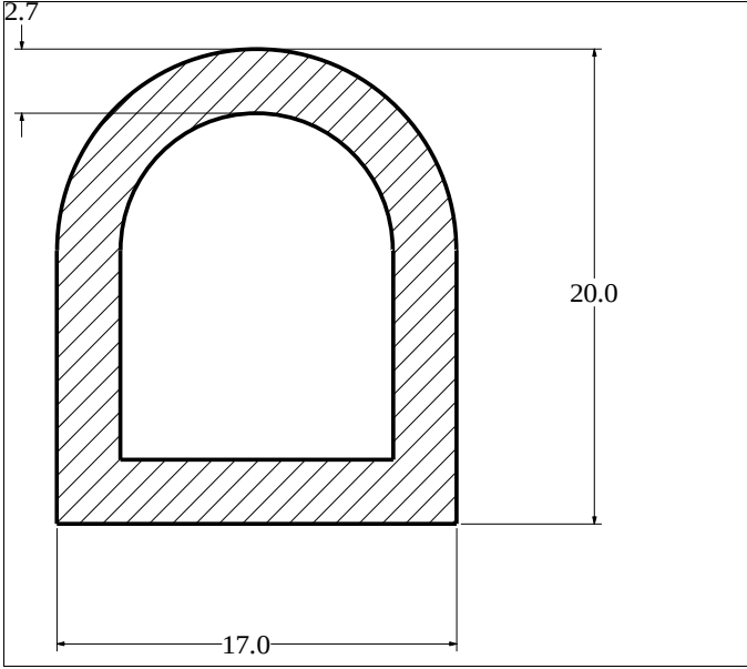
Die No: 1035 Category: D-Hollow
