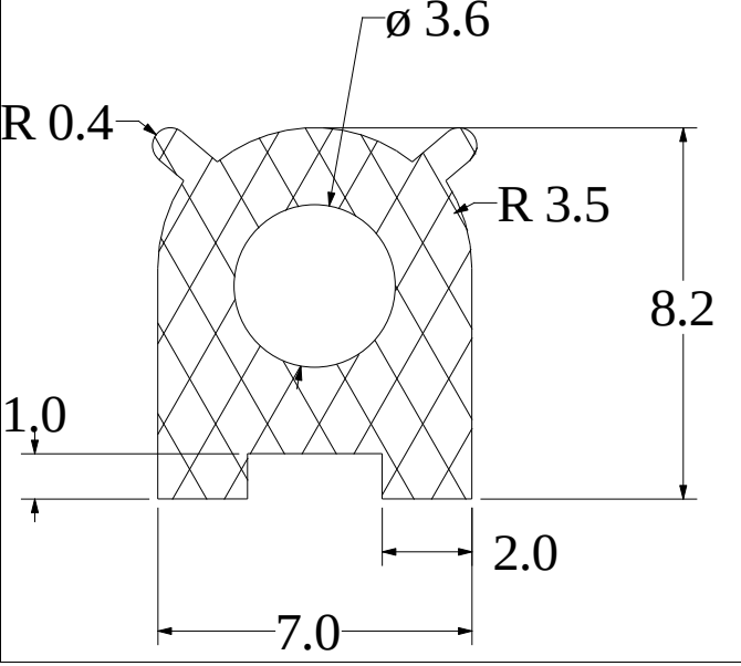
Die No: 2400 Category: D-Hollow
