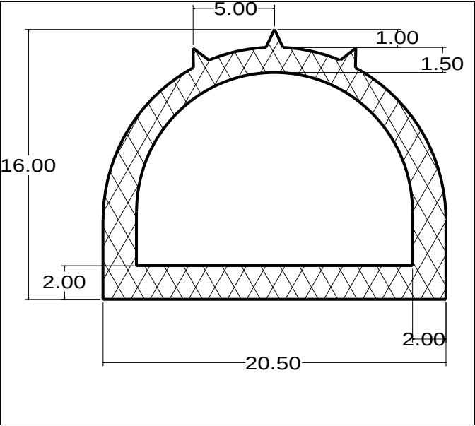
Die No: 4016 Category: D-Hollow
