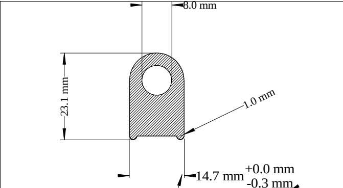
Die No: 1064 Category: D-Hollow
