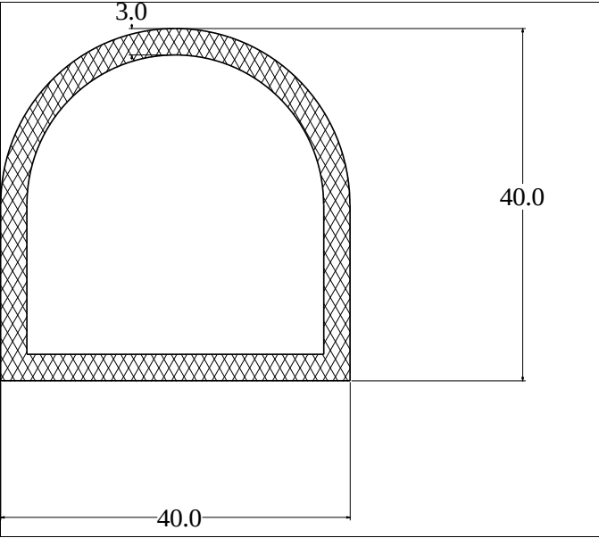
Die No: 2987 Category: D-Hollow
