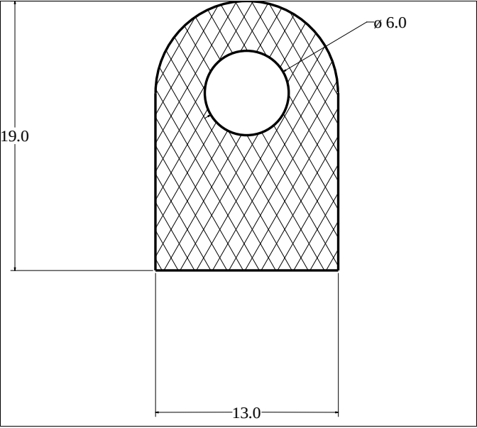
Die No: 3585 Category: D-Hollow
