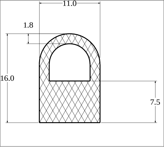
Die No: 2505 Category: D-Hollow
