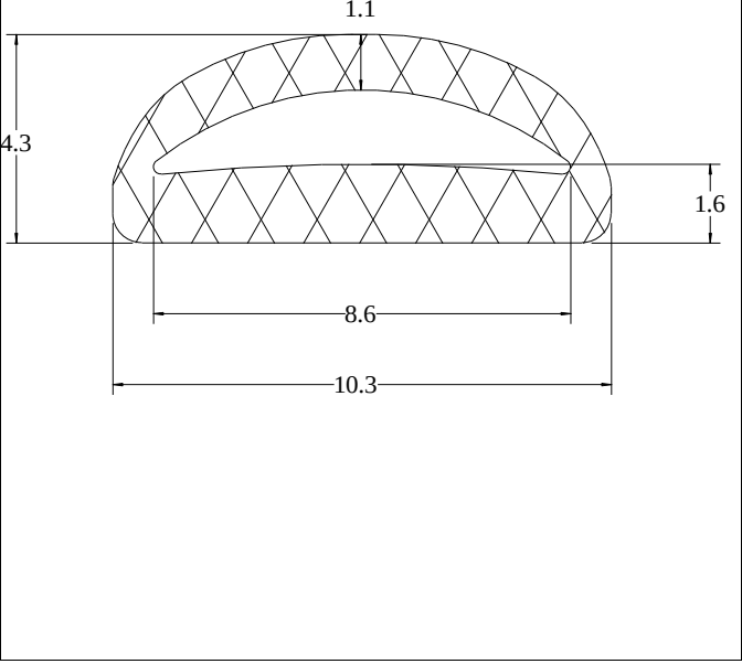
Die No: 5435 Category: D-Hollow
