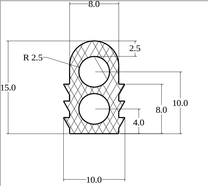
Die No: 3164 Category: D-Hollow
