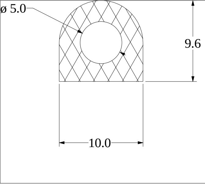
Die No: 4401 Category: D-Hollow
