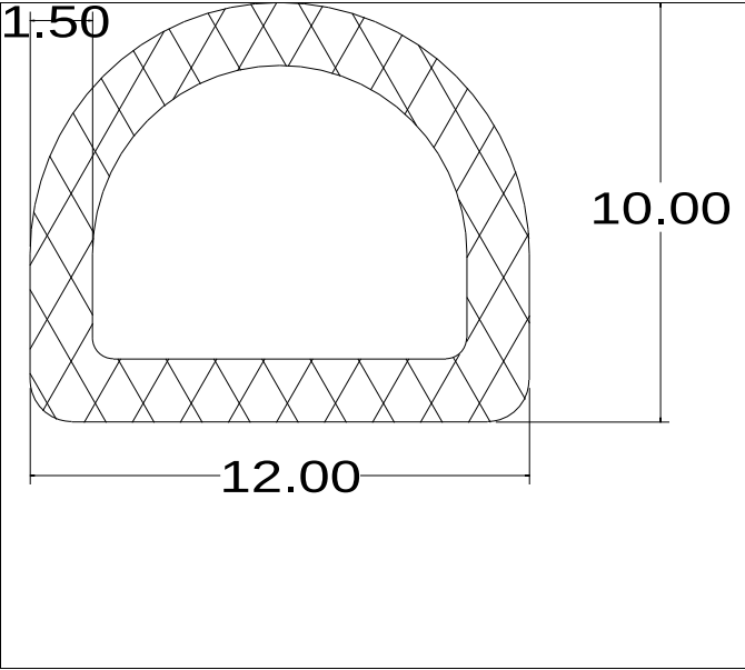
Die No: 4039 Category: D-Hollow
