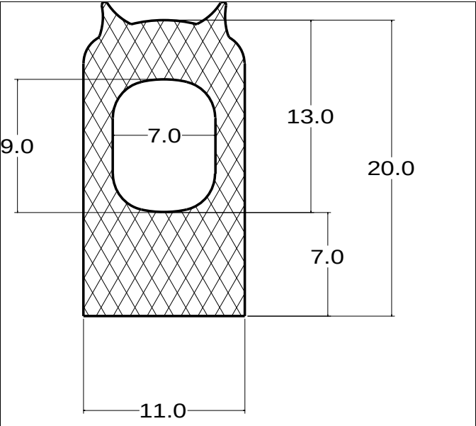
Die No: 4688 Category: D-Hollow
