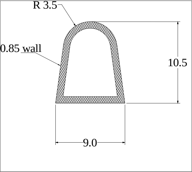
Die No: 2621 Category: D-Hollow
