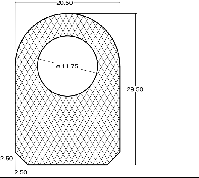
Die No: 5675 Category: D-Hollow
