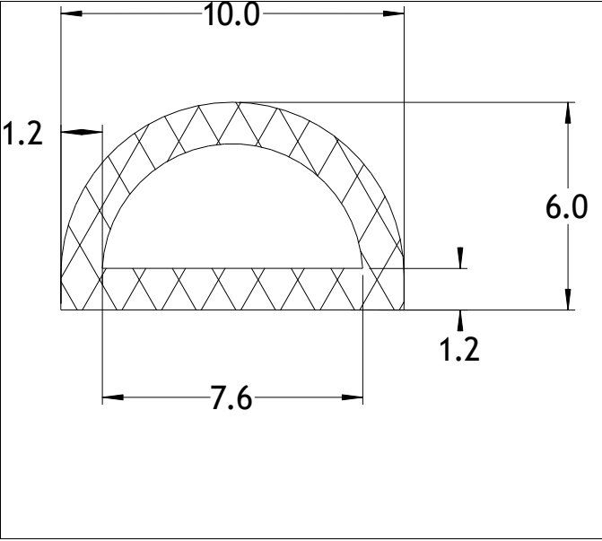
Die No: 7075 Category: D-Hollow
