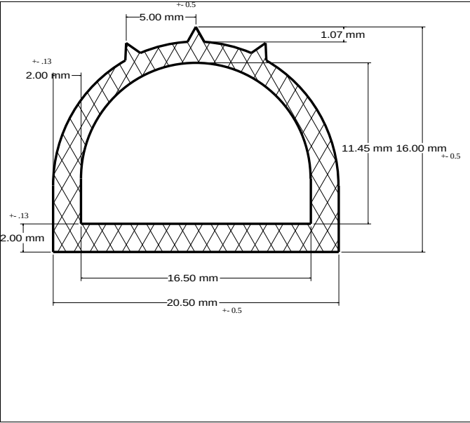
Die No: 3990 Category: D-Hollow
