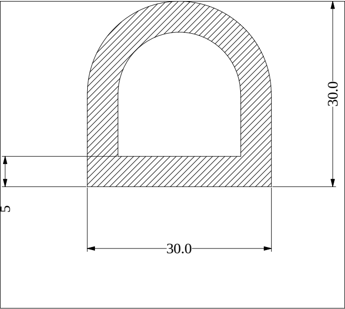
Die No: 134 Category: D-Hollow
