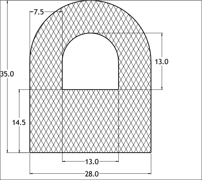
Die No: 6410 Category: D-Hollow
