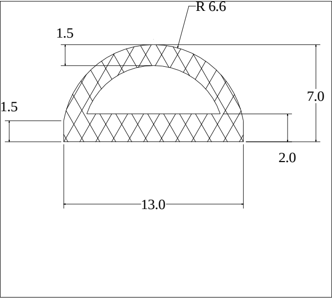
Die No: 3285 Category: D-Hollow
