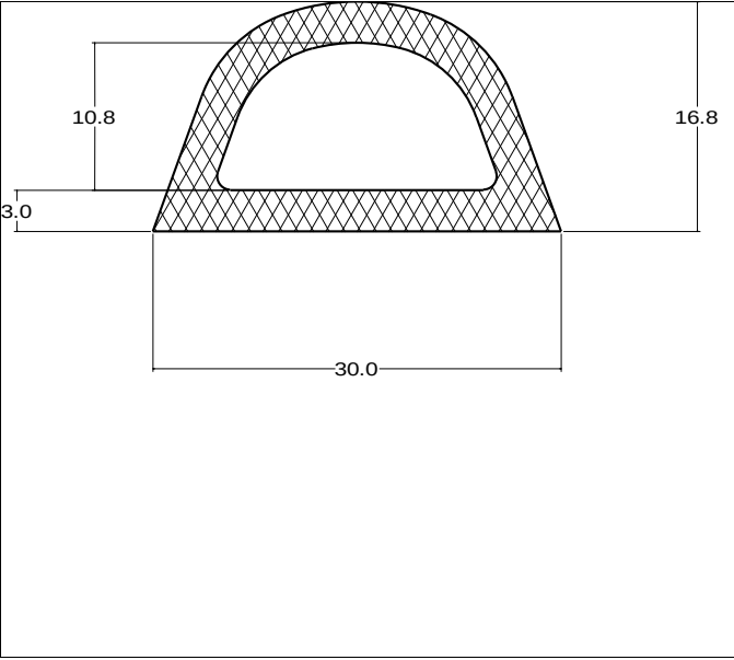
Die No: 4645 Category: D-Hollow
